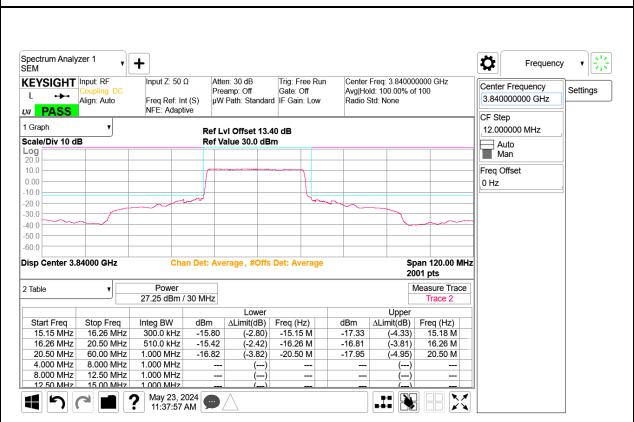
5G NR n77 30MHz BPSK Mid Channel RB75-0 Port B, ID:32061
