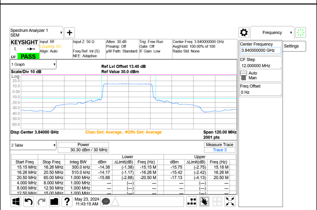
5G NR n77 BPSK Mid Channel RB75-0 Port A+B, ID:32061
