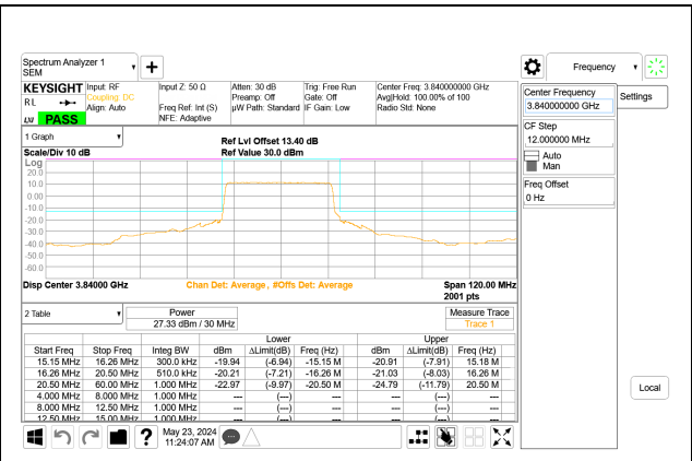
5G NR n77 30MHz BPSK Mid Channel RB75-0 Port A, ID:32061
