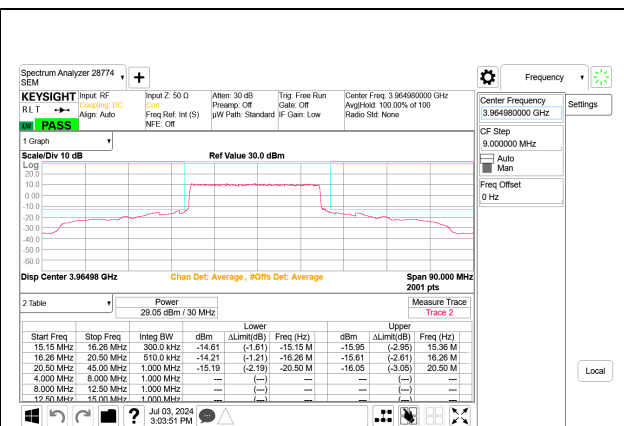
5G NR n77 BPSK BPSK High Channel RB75-0 Port B
