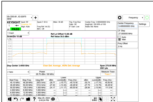
5G NR n77 90MHz BPSK Low Channel RB243-0 Port A
