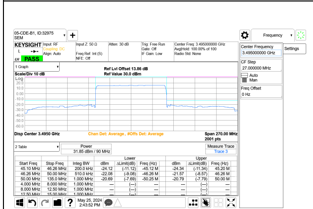
5G NR n77 90MHz BPSK Low Channel RB243-0 Port A+B
