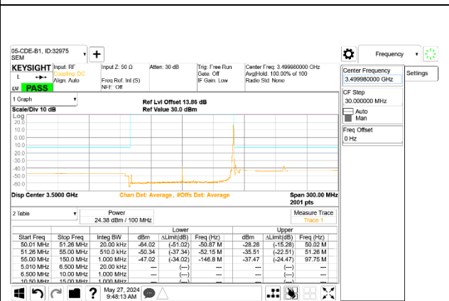
5G NR n77 100MHz BPSK Mid Channel RB1-272 Port B
