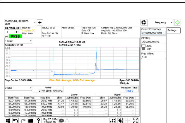
5G NR n77 100MHz BPSK Mid Channel RB1-272 Port A+B
