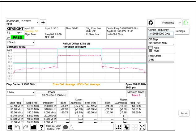
5G NR n77 100MHz BPSK Middle Channel RB270-0 Port B
