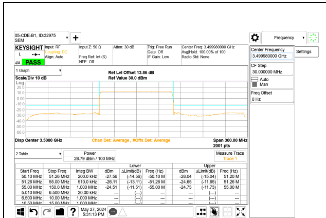
5G NR n77 100MHz BPSK Middle Channel RB270-0 Port A
