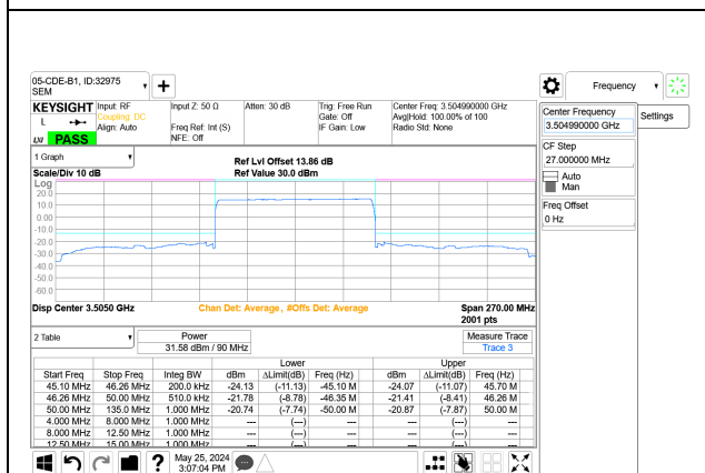
5G NR n77 90MHz BPSK High Channel RB243-0 Port A+B
