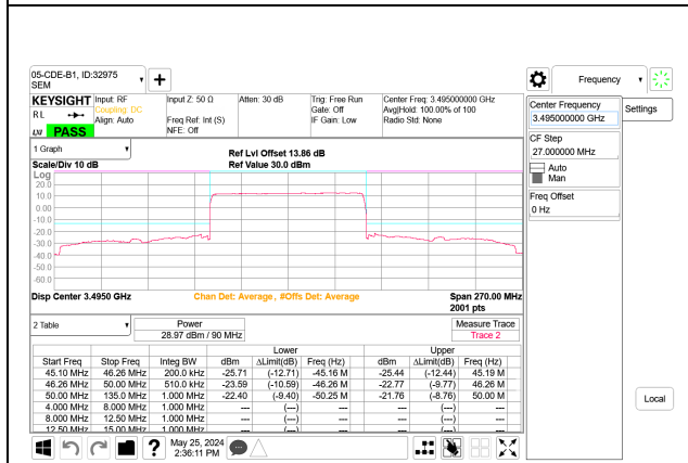
5G NR n77 90MHz BPSK Low Channel RB243-0 Port B
