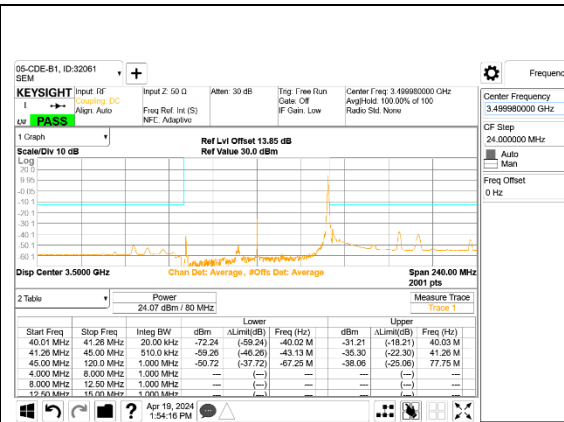
5G NR n77 80MHz BPSK Mid Channel RB1-216 Port A
