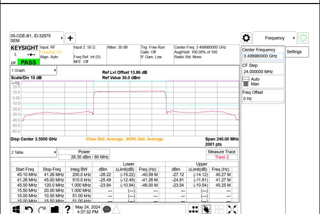
5G NR n77 80MHz BPSK Mid Channel RB216-0 Port B
