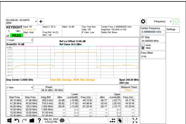
5G NR n77 80MHz BPSK Mid Channel RB216-0 Port A
