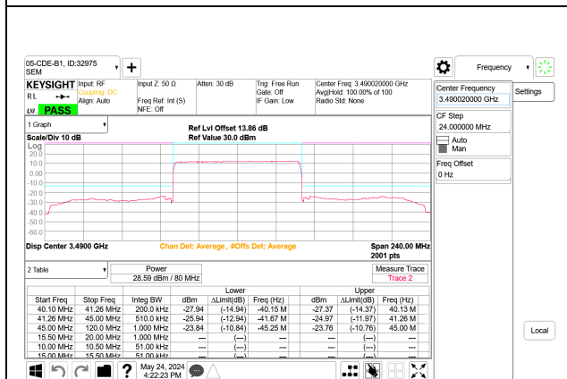
5G NR n77 80MHz BPSK Low Channel RB216-0 Port B
