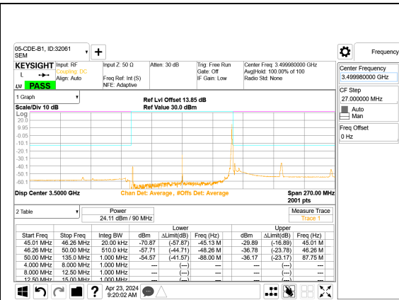
5G NR n77 90MHz BPSK Mid Channel RB1-244 Port A
