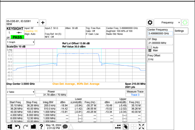
5G NR n77 70MHz BPSK Mid Channel RB180-0 Port A+B
