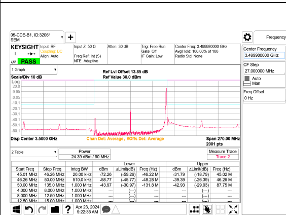
5G NR n77 90MHz BPSK Mid Channel RB1-244 Port B
