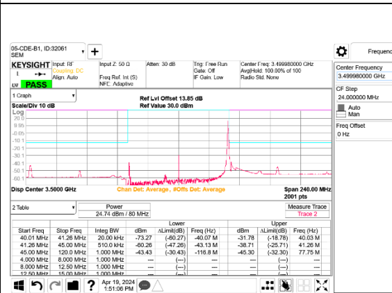
5G NR n77 80MHz BPSK Mid Channel RB1-216 Port B
