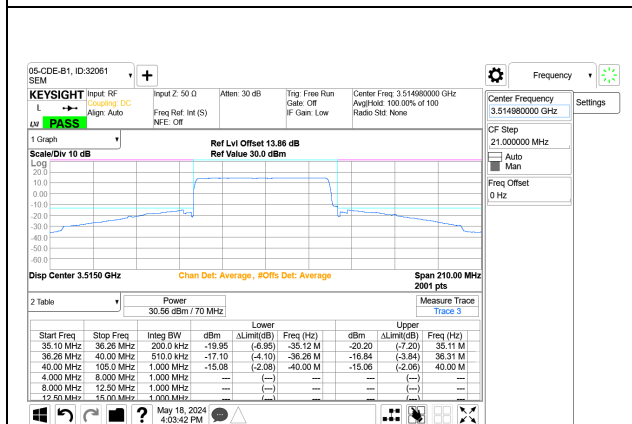
5G NR n77 70MHz BPSK High Channel RB180-0 Port A+B
