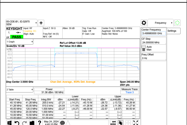
5G NR n77 80MHz BPSK Mid Channel RB216-0 Port A+B
