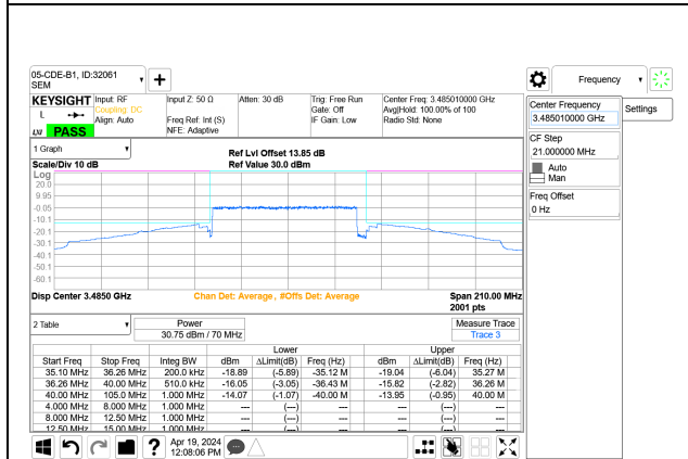
5G NR n77 70MHz BPSK Low Channel RB180-0 Port A+B
