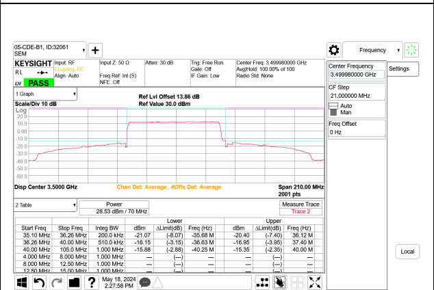
5G NR n77 70MHz BPSK Mid Channel RB180-0 Port B
