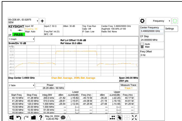
5G NR n77 80MHz BPSK Low Channel RB216-0 Port A
