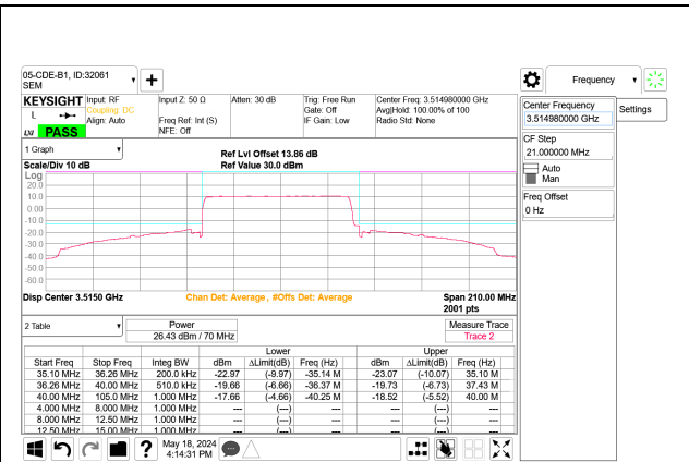
5G NR n77 70MHz BPSK High Channel RB180-0 Port B
