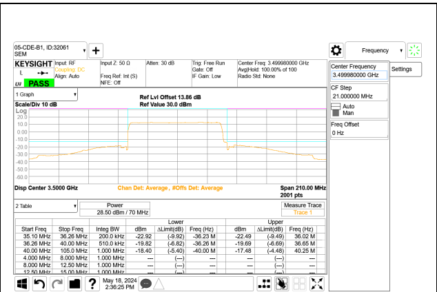
5G NR n77 70MHz BPSK Mid Channel RB180-0 Port A
