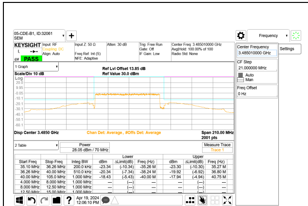
5G NR n77 70MHz BPSK Low Channel RB180-0 Port A
