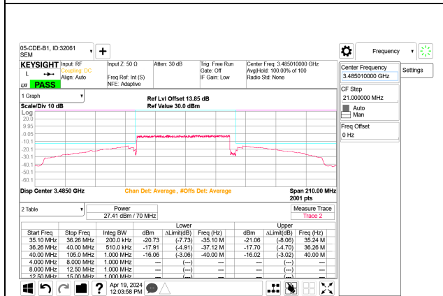
5G NR n77 70MHz BPSK Low Channel RB180-0 Port B
