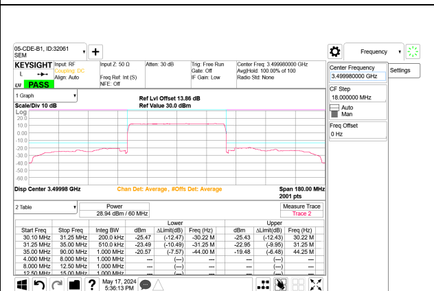
5G NR n77 60MHz BPSK Mid Channel RB162-0 Port B
