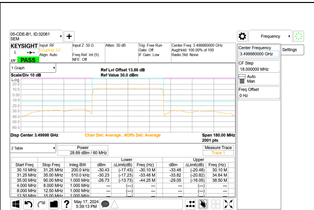
5G NR n77 60MHz BPSK Mid Channel RB162-0 Port A
