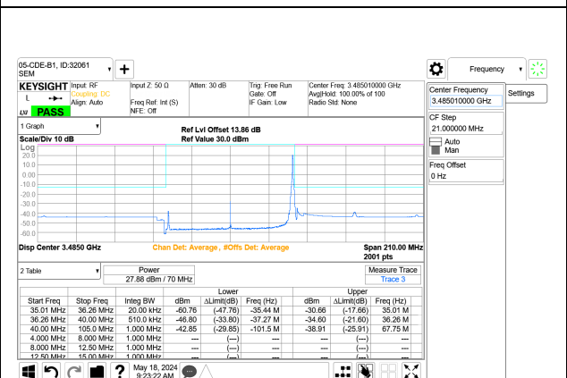
5G NR n77 70MHz BPSK Low Channel RB1-188 Port A+B
