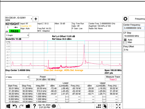
5G NR n77 60MHz BPSK Mid Channel RB1-161 Port B
