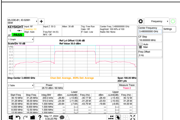
5G NR n77 60MHz BPSK Low Channel RB162-0 Port B
