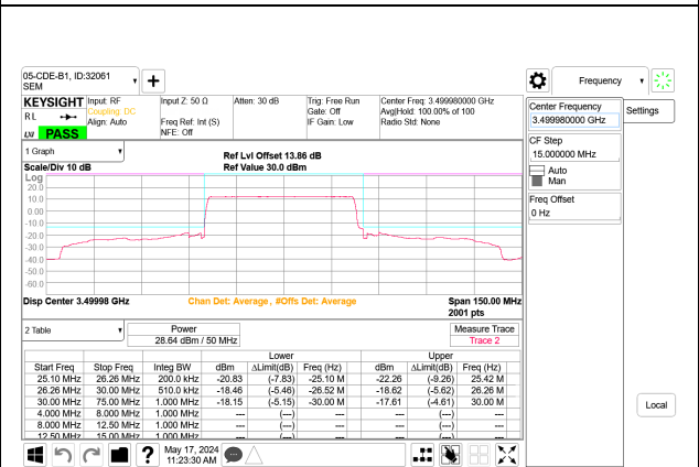
5G NR n77 50MHz BPSK Mid Channel RB128-0 Port B
