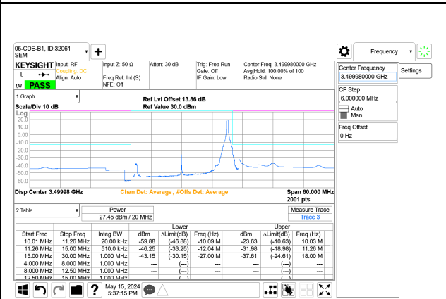
5G NR n77 20MHz BPSK Mid Channel RB1-50 Port A+B
