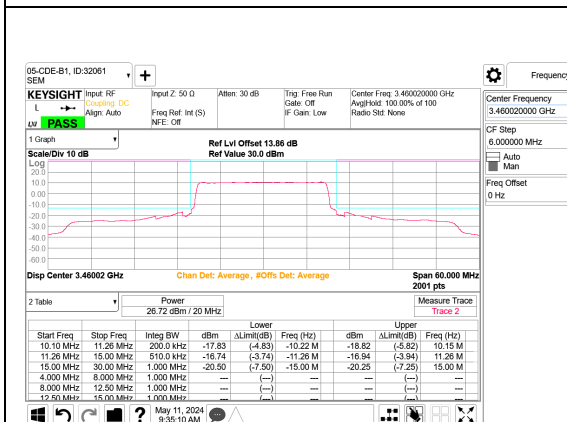
5G NR n77 20MHz BPSK Low Channel RB50-0 Port B
