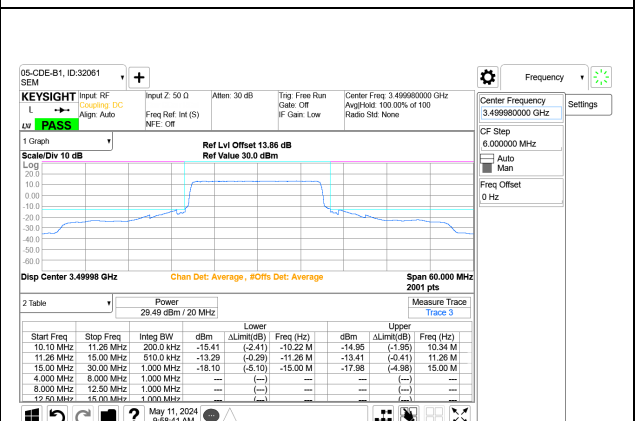
5G NR n77 20MHz BPSK Mid Channel RB50-0 Port A+B
