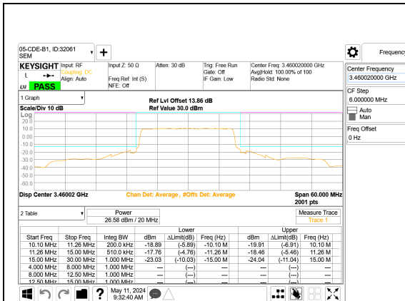
5G NR n77 20MHz BPSK Low Channel RB50-0 Port A
