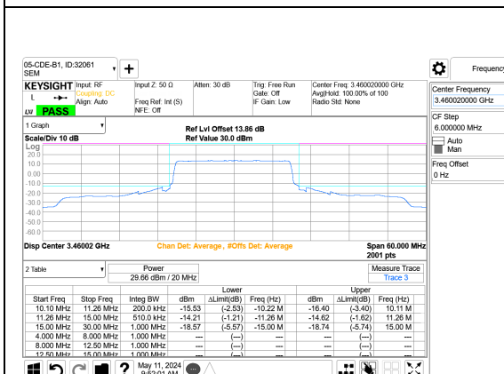
5G NR n77 20MHz BPSK Low Channel RB50-0 Port A+B
