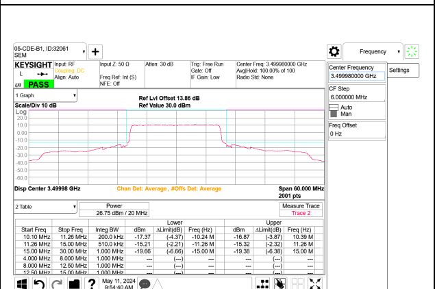
5G NR n77 20MHz BPSK Mid Channel RB50-0 Port B
