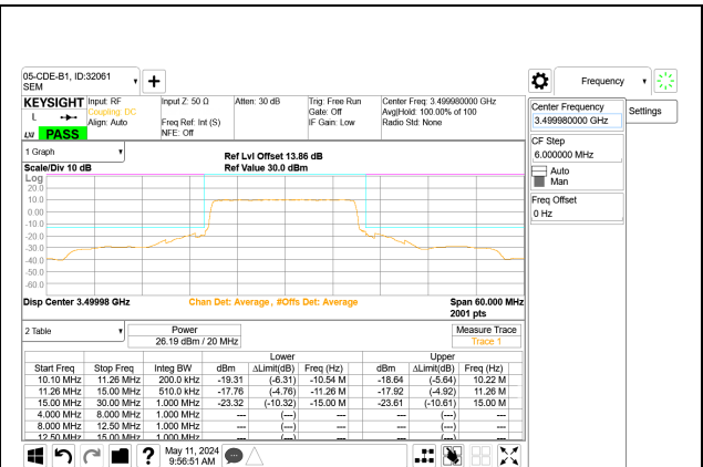
5G NR n77 20MHz BPSK Mid Channel RB50-0 Port A
