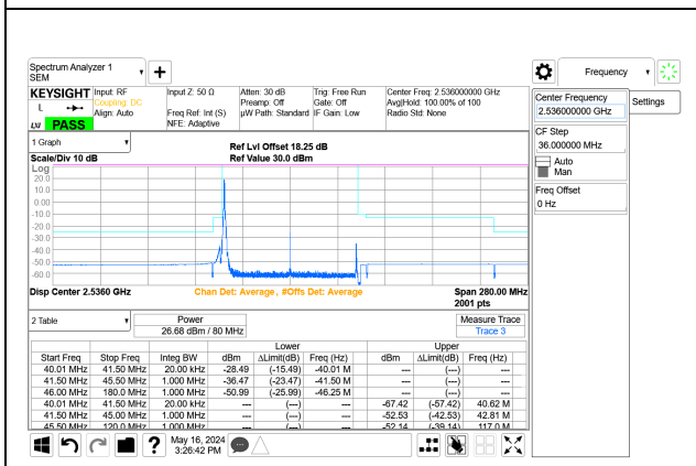
5G NR n41 80MHz BPSK Low Channel RB1-0 Port A+B ID: 32546
