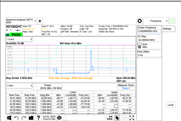
5G NR n41 80MHz BPSK Mid Channel RB1-216 Port A+B
