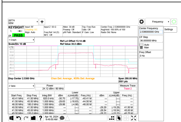
5G NR n41 80MHz BPSK Low Channel RB216-0 Port B
