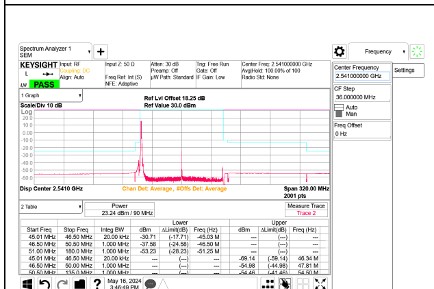
5G NR n41 90MHz BPSK Low Channel RB1-0 Port B ID: 32546
