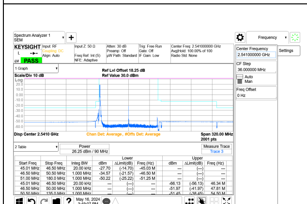
5G NR n41 90MHz BPSK Low Channel RB1-0 Port A+B ID: 32546
