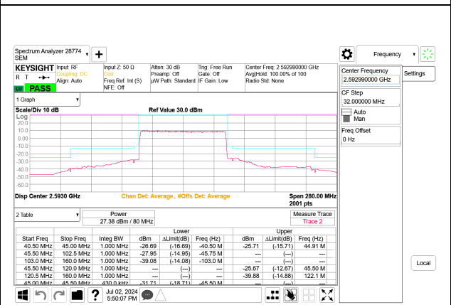
5G NR n41 80MHz BPSK Mid Channel RB216-0 Port B
