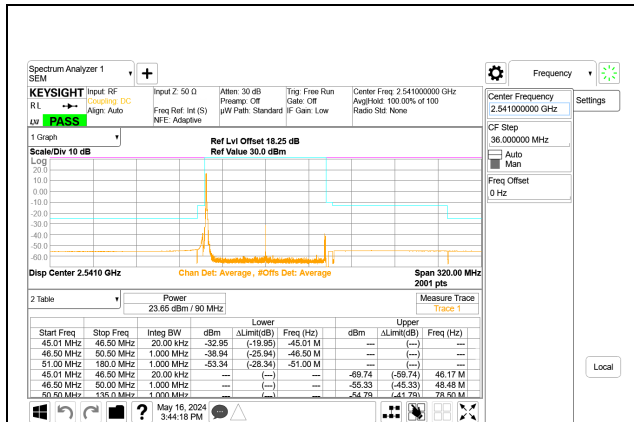
5G NR n41 90MHz BPSK Low Channel RB1-0 Port A ID: 32546
