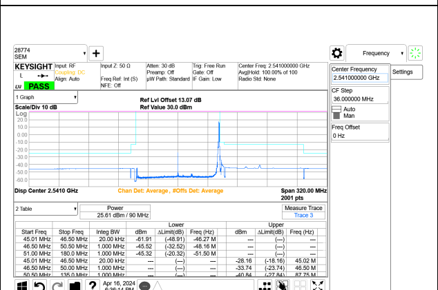
5G NR n41 90MHz BPSK Low Channel RB1-244 Port A+B ID: 32546
