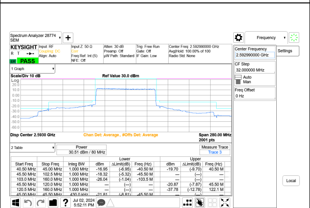
5G NR n41 80MHz BPSK Mid Channel RB216-0 Port A+B
