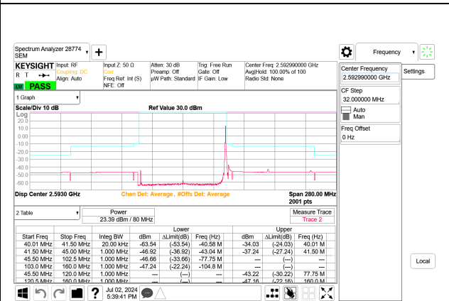
5G NR n41 80MHz BPSK Mid Channel RB1-216 Port B
