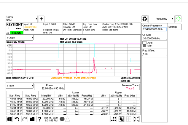
5G NR n41 90MHz BPSK Low Channel RB1-244 Port B ID: 32546
