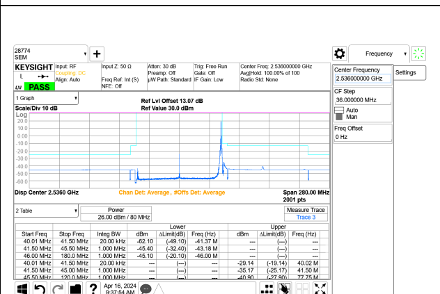
5G NR n41 80MHz BPSK Low Channel RB1-216 Port A+B
