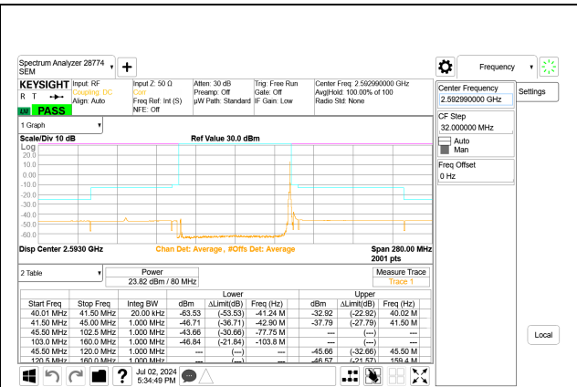
5G NR n41 80MHz BPSK Mid Channel RB1-216 Port A
