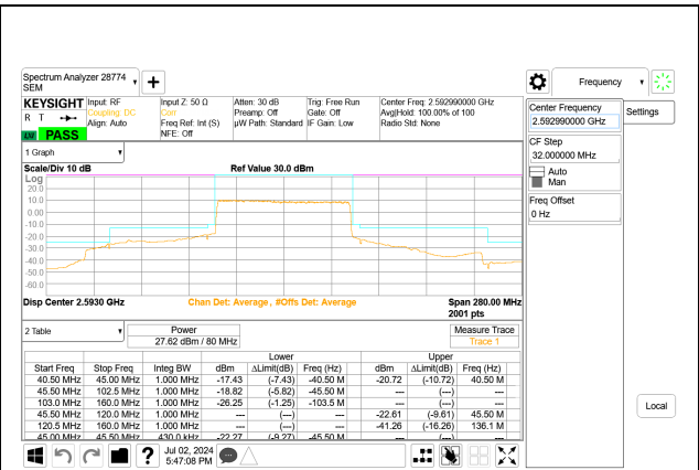
5G NR n41 80MHz BPSK Mid Channel RB216-0 Port A
