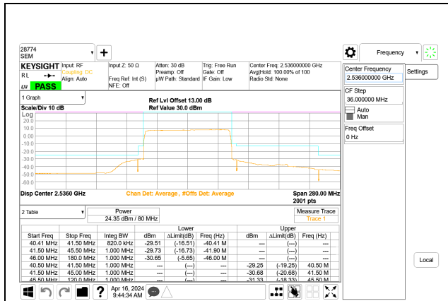
5G NR n41 80MHz BPSK Low Channel RB216-0 Port A
