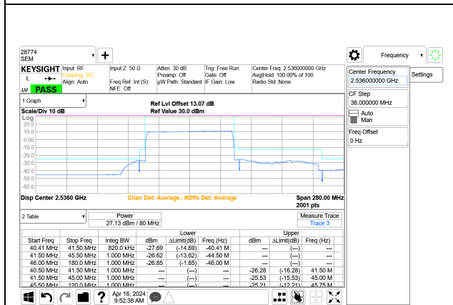
5G NR n41 80MHz BPSK Low Channel RB216-0 Port A+B
