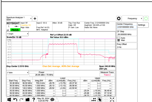
5G NR n41 70MHz BPSK Low Channel RB180-0 Port B ID: 32546
