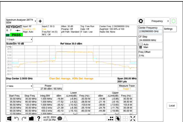
5G NR n41 60MHz BPSK Mid Channel RB162-0 Port
