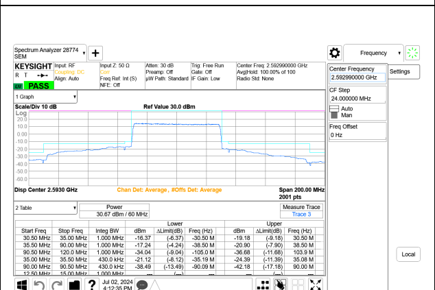
5G NR n41 60MHz BPSK Mid Channel RB162-0 Port A+B
