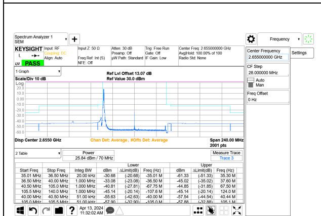
5G NR n41 70MHz BPSK High Channel RB1-0 Port A+B ID: 32546
