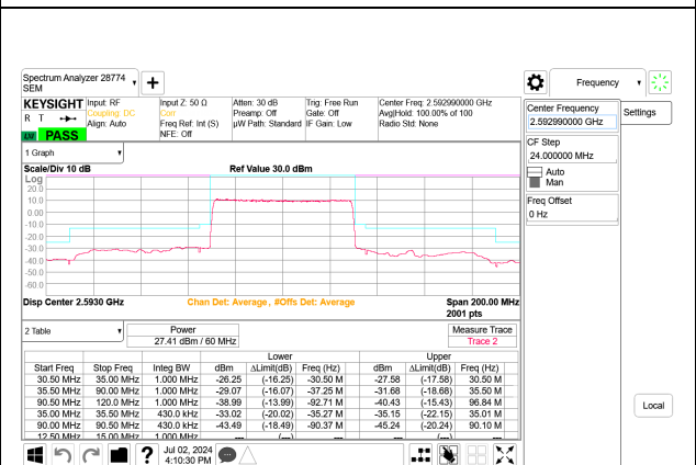
5G NR n41 60MHz BPSK Mid Channel RB162-0 Port B
