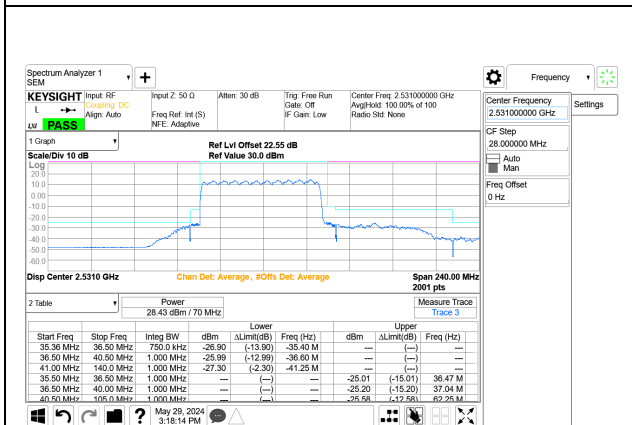
5G NR n41 70MHz BPSK Low Channel RB180-0 Port A+B ID: 32546
