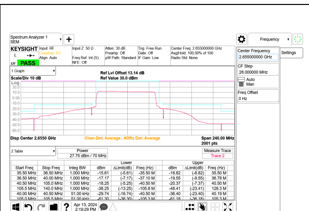
5G NR n41 70MHz BPSK High Channel RB180-0 Port B ID: 32546
