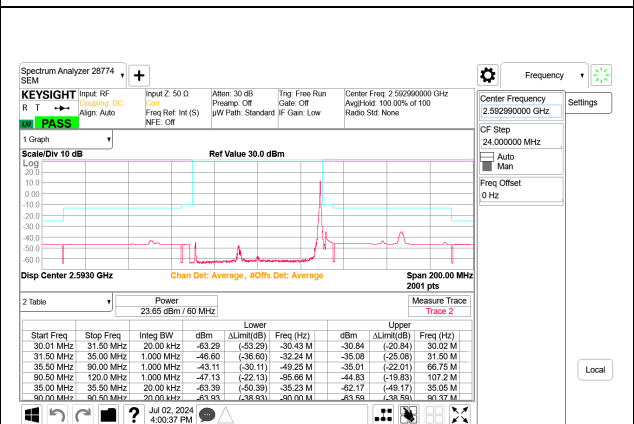
5G NR n41 60MHz BPSK Mid Channel RB1-161 Port B
