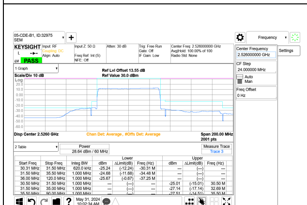
5G NR n41 60MHz BPSK Low Channel RB162-0 Port A+B
