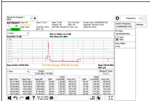
5G NR n41 70MHz BPSK High Channel RB1-0 Port B ID: 32546
