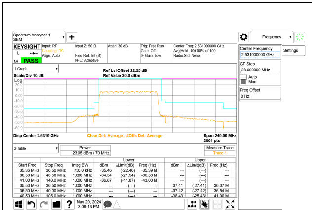
5G NR n41 70MHz BPSK Low Channel RB180-0 Port A ID: 32546
