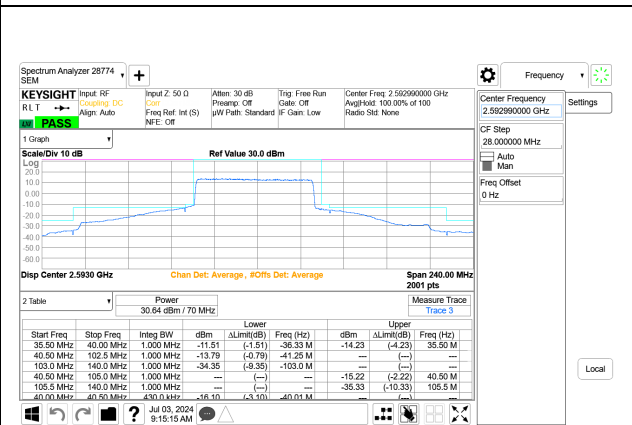
5G NR n41 70MHz BPSK Mid Channel RB180-0 Port A+B
