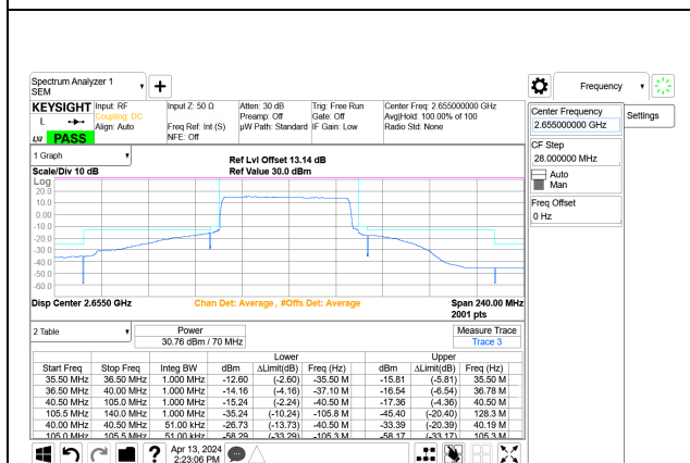
5G NR n41 70MHz BPSK High Channel RB180-0 Port A+B ID: 32546
