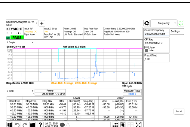
5G NR n41 70MHz BPSK Mid Channel RB1-188 Port A+B
