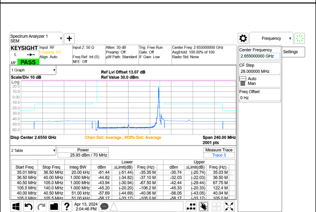
5G NR n41 70MHz BPSK High Channel RB1-188 Port A+B ID: 32546
