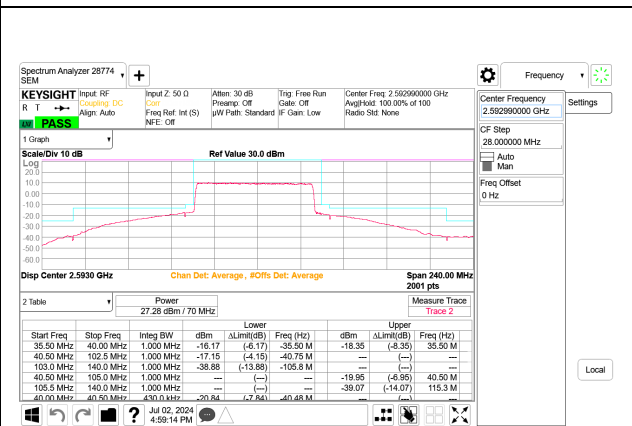
5G NR n41 70MHz BPSK Mid Channel RB180-0 Port B
