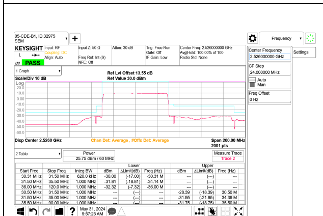
5G NR n41 60MHz BPSK Low Channel RB162-0 Port B
