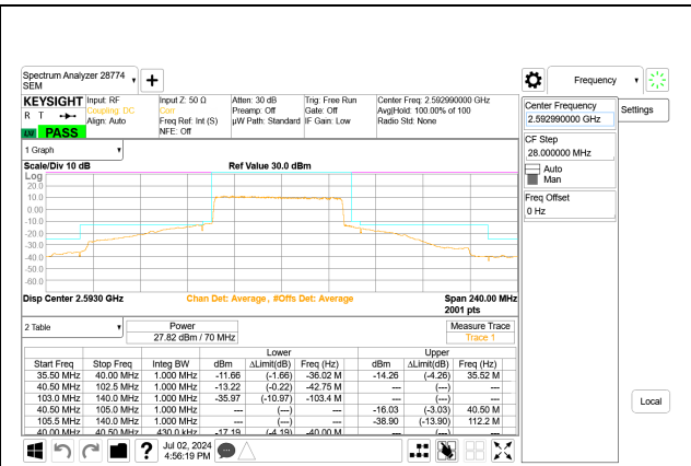
5G NR n41 70MHz BPSK Mid Channel RB180-0 Port
