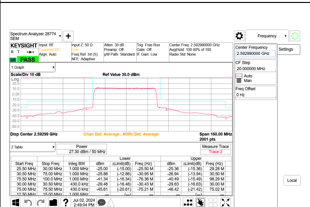
5G NR n41 50MHz BPSK Mid Channel RB128-0 Port
