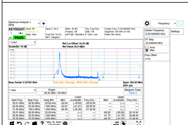
5G NR n41 50MHz BPSK Low Channel RB1-0 Port A+B ID: 32546
