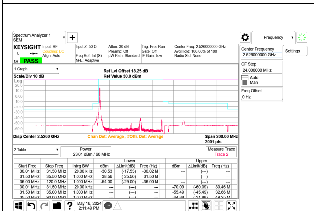
5G NR n41 60MHz BPSK Low Channel RB1-0 Port B ID: 32546
