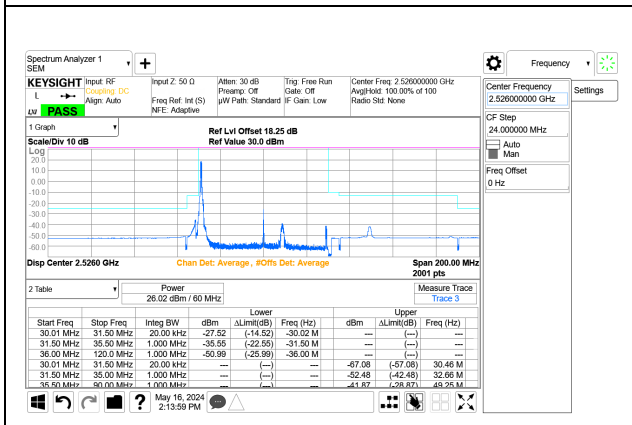
5G NR n41 60MHz BPSK Low Channel RB1-0 Port A+B ID: 32546
