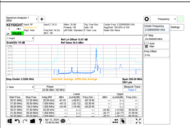
5G NR n41 60MHz BPSK Low Channel RB1-161 Port A+B ID: 32546
