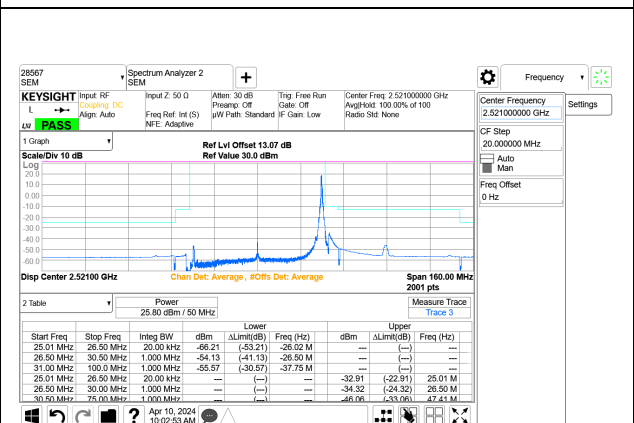
5G NR n41 50MHz BPSK Low Channel RB1-132 Port A+B ID:
