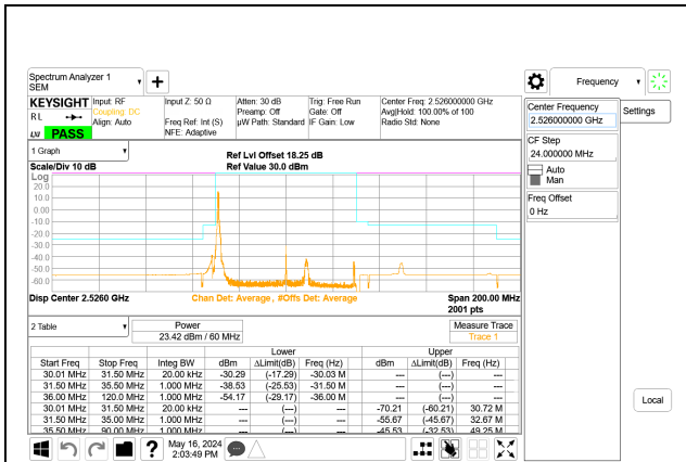
5G NR n41 60MHz BPSK Low Channel RB1-0 Port A ID: 32546
