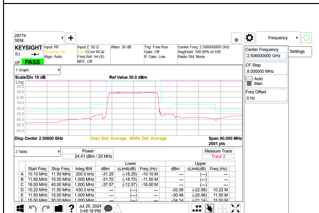
5G NR n41 20MHz BPSK Low Channel RB50-0 Port B
