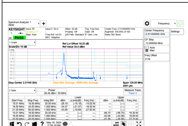
5G NR n41 30MHz BPSK Low Channel RB1-0 Port A+B ID: 32546
