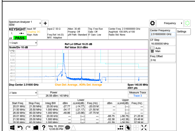
5G NR n41 40MHz BPSK Low Channel RB1-0 Port A+B ID: 32546
