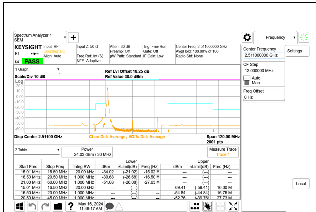
5G NR n41 30MHz BPSK Low Channel RB1-0 Port A, ID: 32546
