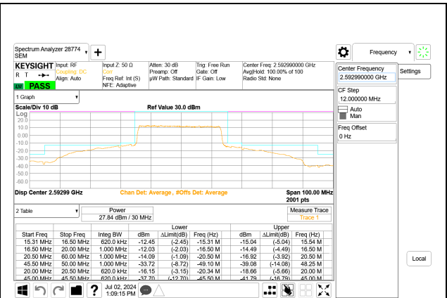
5G NR n41 30MHz BPSK Mid Channel RB75-0 Port A
