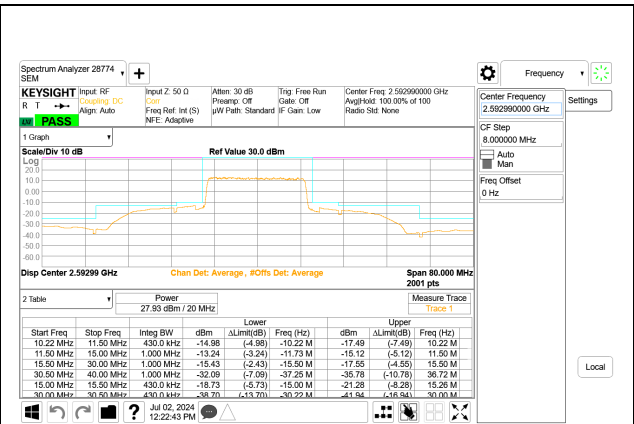
5G NR n41 20MHz BPSK Mid Channel RB50-0 Port A
