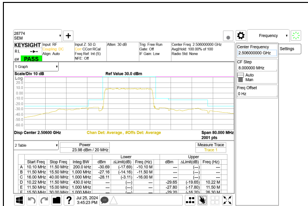
5G NR n41 20MHz BPSK Low Channel RB50-0 Port A
