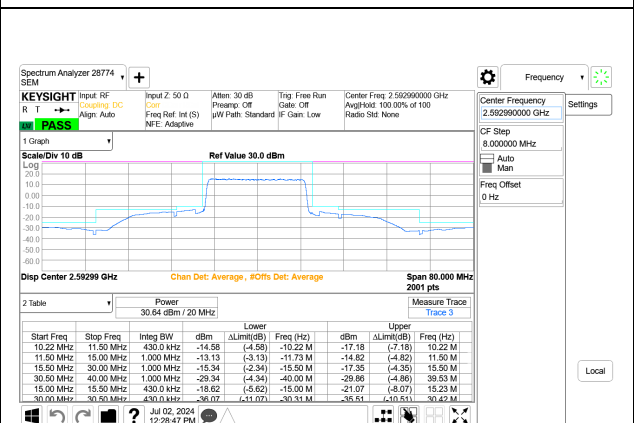
5G NR n41 20MHz BPSK Mid Channel RB50-0 Port A+B
