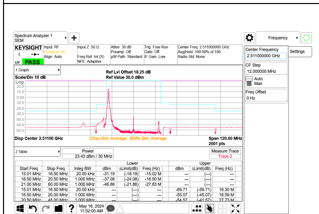
5G NR n41 30MHz BPSK Low Channel RB1-0 Port B ID: 32546
