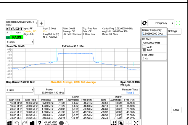
5G NR n41 30MHz BPSK Mid Channel RB75-0 Port A+B
