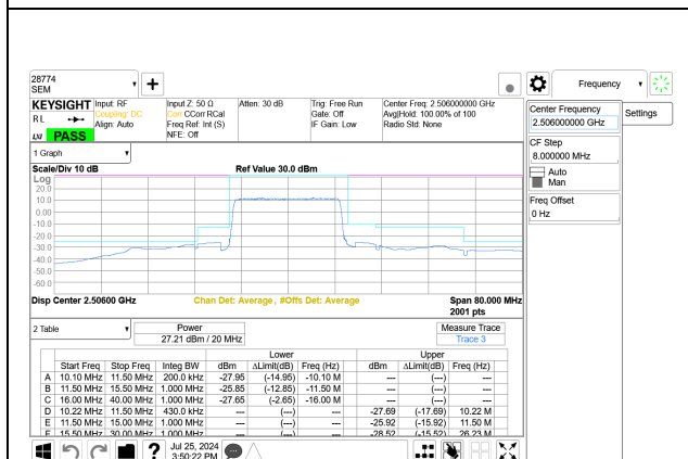
5G NR n41 20MHz BPSK Low Channel RB50-0 Port A+B
