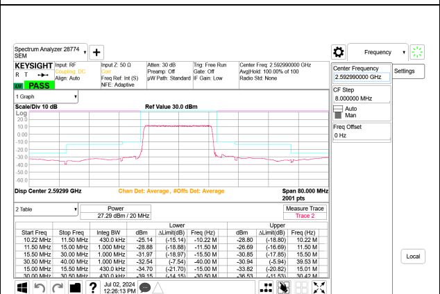
5G NR n41 20MHz BPSK Mid Channel RB50-0 Port B
