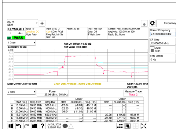
5G NR n41 30MHz BPSK Low Channel RB75-0 Port B
