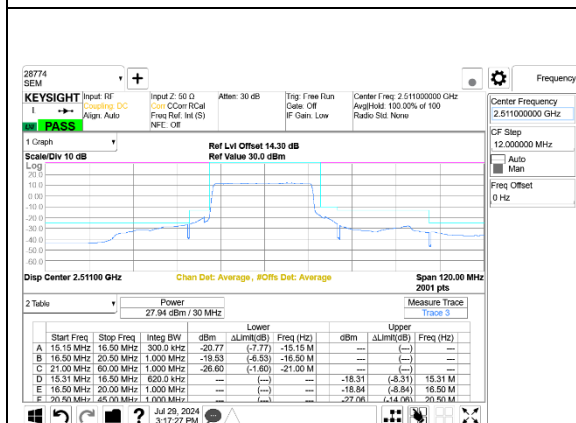
5G NR n41 30MHz BPSK Low Channel RB75-0 Port A+B
