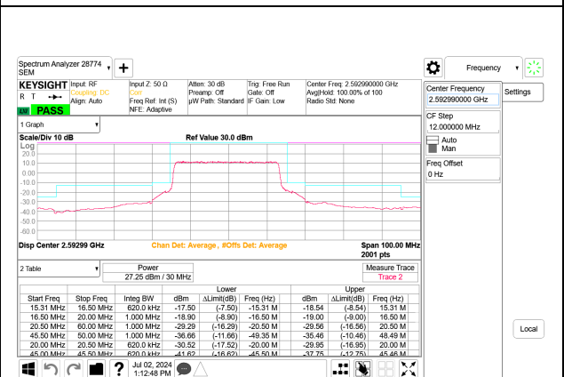
5G NR n41 30MHz BPSK Mid Channel RB75-0 Port B
