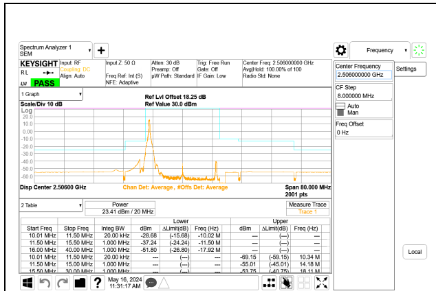
5G NR n41 20MHz BPSK Low Channel RB1-0 Port A ID: 32546
