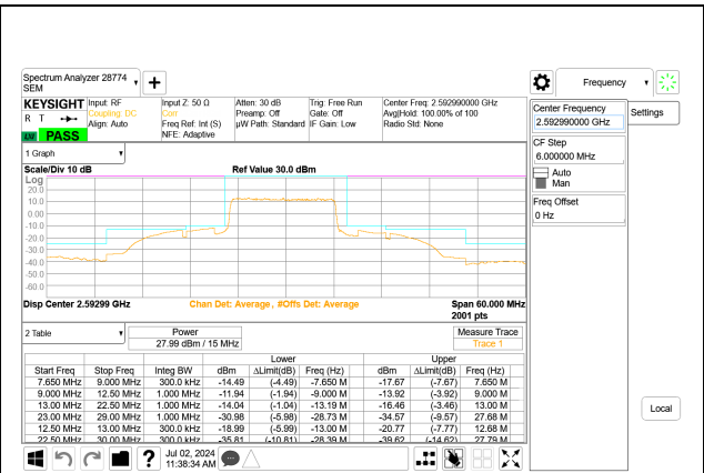
5G NR n41 15MHz BPSK Mid Channel RB36-0 Port A
