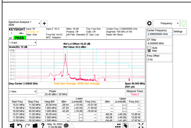
5G NR n41 20MHz BPSK Low Channel RB1-0 Port B, ID: 32546
