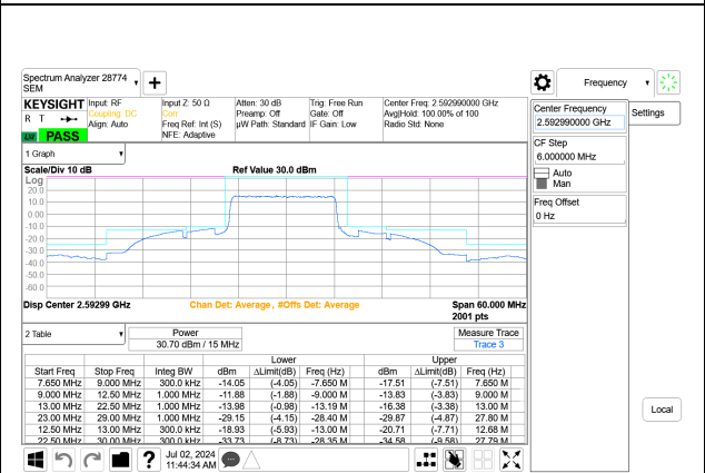
5G NR n41 15MHz BPSK Mid Channel RB36-0 Port A+B
