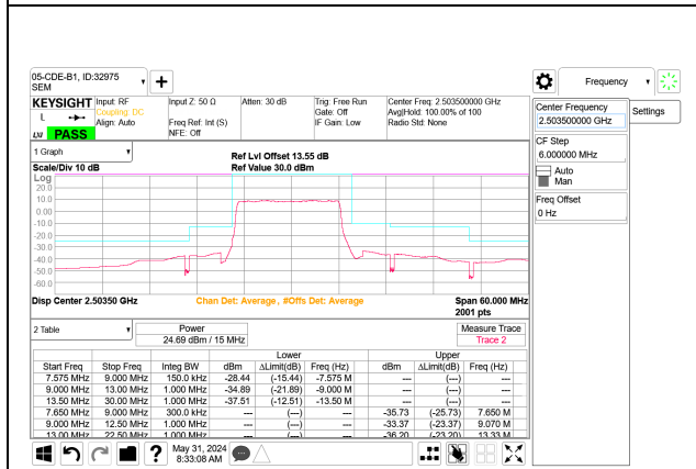
5G NR n41 15MHz BPSK Low Channel RB36-0 Port B
