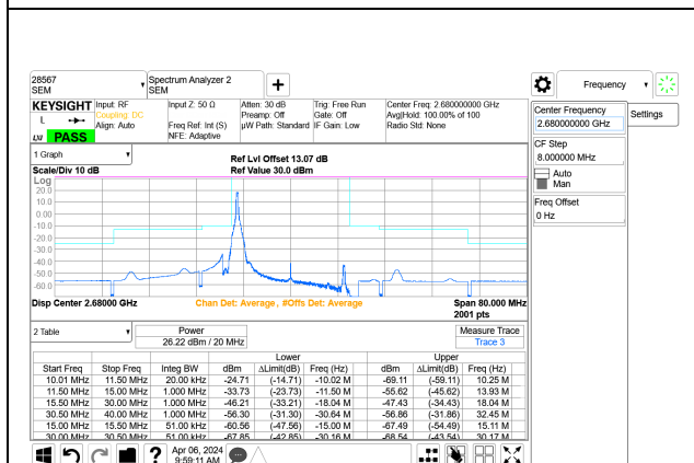
5G NR n41 20MHz BPSK High Channel RB1-0 Port A+B
