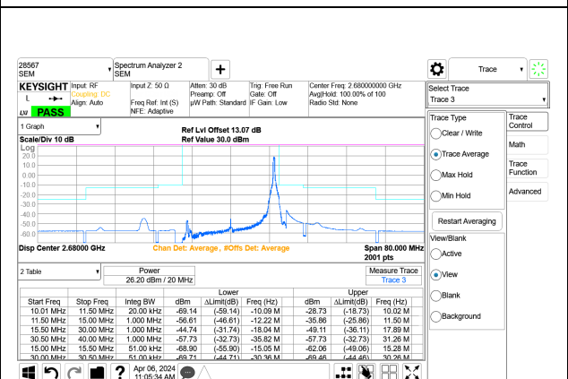
5G NR n41 20MHz BPSK High Channel RB1-50 Port A+B
