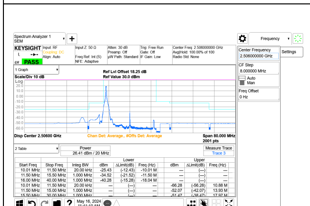
5G NR n41 20MHz BPSK Low Channel RB1-0 Port A+B ID: 32546
