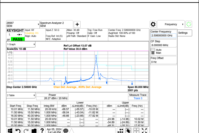
5G NR n41 20MHz BPSK Low Channel RB1-50 Port A+B
