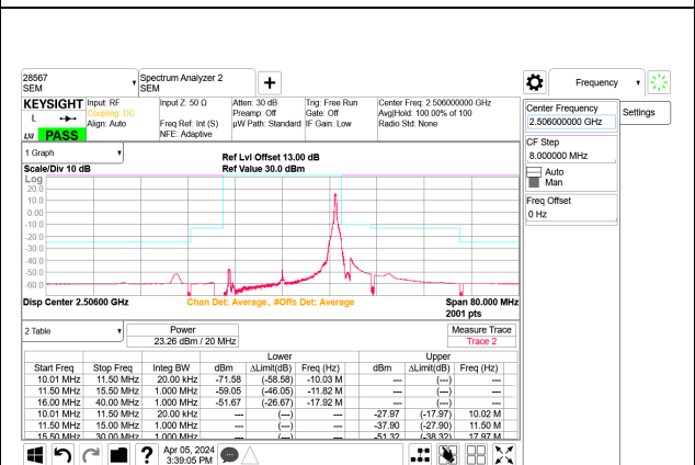
5G NR n41 20MHz BPSK Low Channel RB1-50 Port B
