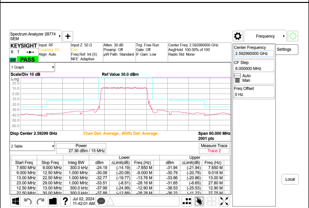
5G NR n41 15MHz BPSK Mid Channel RB36-0 Port B
