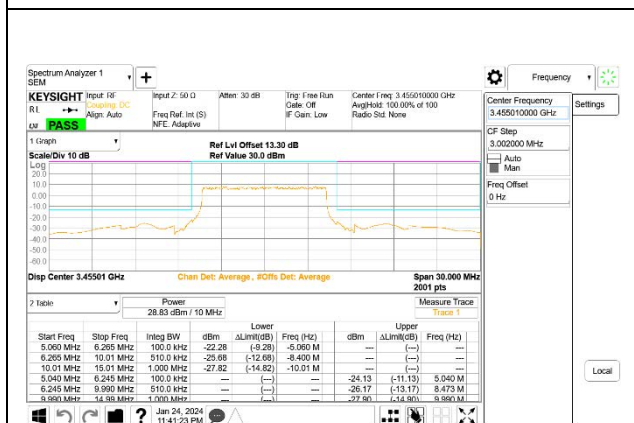
5G NR n77 10MHz BPSK Low Channel RB24-0, ID:27957
