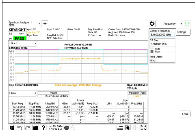
5G NR n77 20MHz BPSK Low Channel RB50-0, ID:27957
