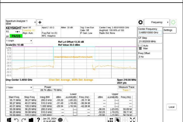
5G NR n77 70MHz BPSK Low Channel RB180-0, ID:27957
