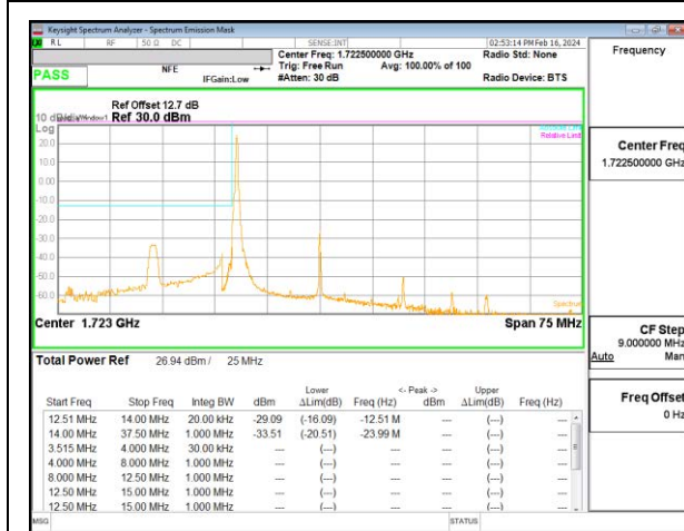
5G NR n66 25MHz BPSK Low Channel RB1-0, ID:27342
