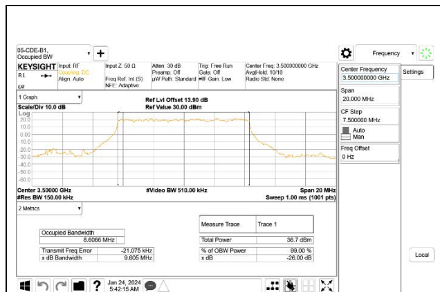
5G NR n77 10MHz BPSK Middle Channel RB24-0, ID 27342
