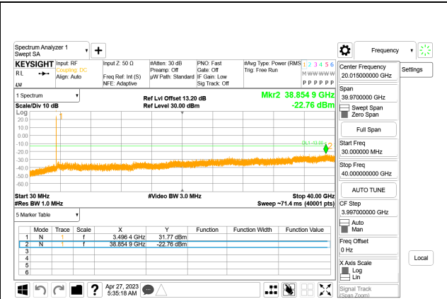
5G NR n77 10MHz BPSK Middle Channel RB1-1, ID:19210
