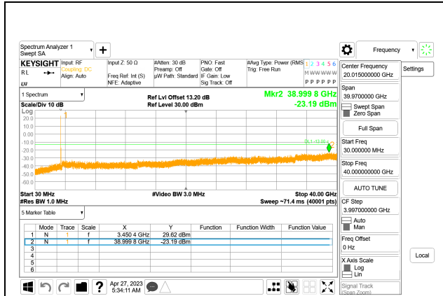
5G NR n77 10MHz BPSK Low Channel RB1-0, ID:19210
