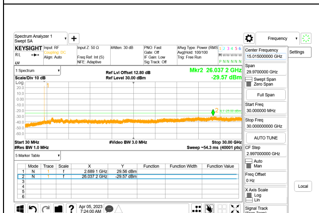
5G NR n41 20MHz BPSK High Channel RB1-50, ID:19210
