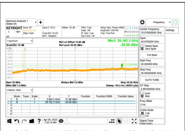
5G NR n41 20MHz BPSK Middle Channel RB1-1, ID:19210
