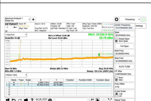
5G NR n41 70MHz BPSK High Channel RB1-188, ID:19210
