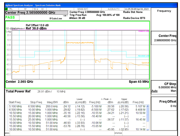
5G NR n7 10MHz BPSK High Channel RB50-0, ID:28568
