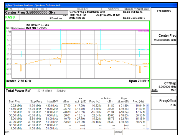
5G NR n7 20MHz BPSK High Channel RB100-0, ID:28568
