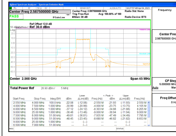
5G NR n7 5MHz BPSK High Channel RB25-0, ID:28568
