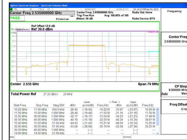
5G NR n7 20MHz BPSK Middle Channel RB100-0, ID:28568
