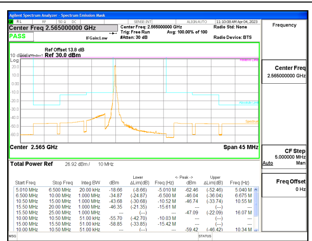
5G NR n7 10MHz BPSK High Channel RB1-0, ID:28568
