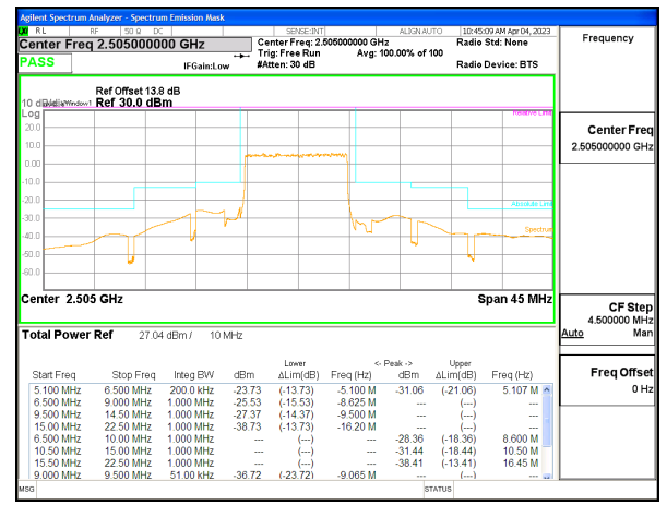
5G NR n7 10MHz BPSK Low Channel RB50-0, ID:28568
