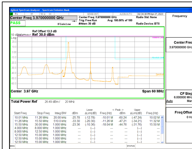
5G NR n77 20MHz BPSK High Channel RB1-0, ID:28568
