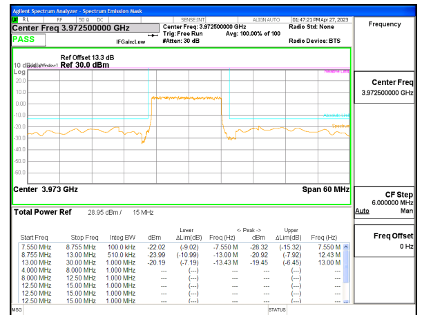
5G NR n77 15MHz BPSK High Channel RB36-0, ID:28568
