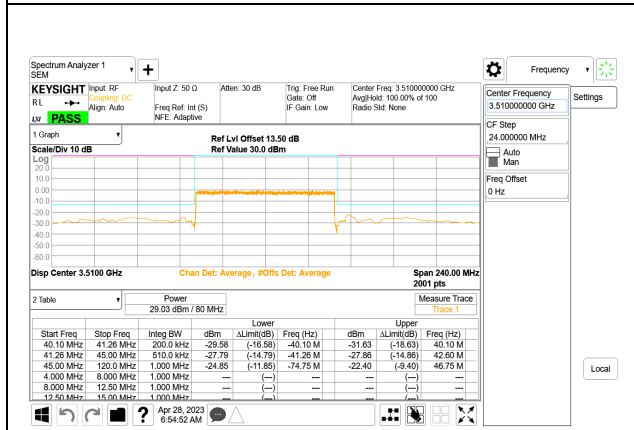
5G NR n77 80MHz BPSK High Channel RB216-0, ID:28568
