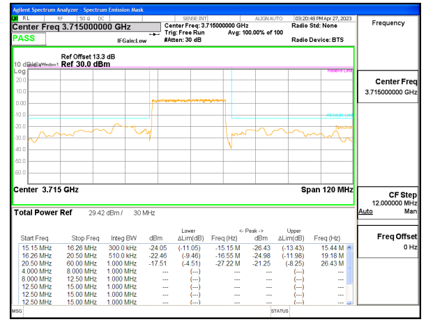
5G NR n77 30MHz BPSK Low Channel RB75-0, ID:28568
