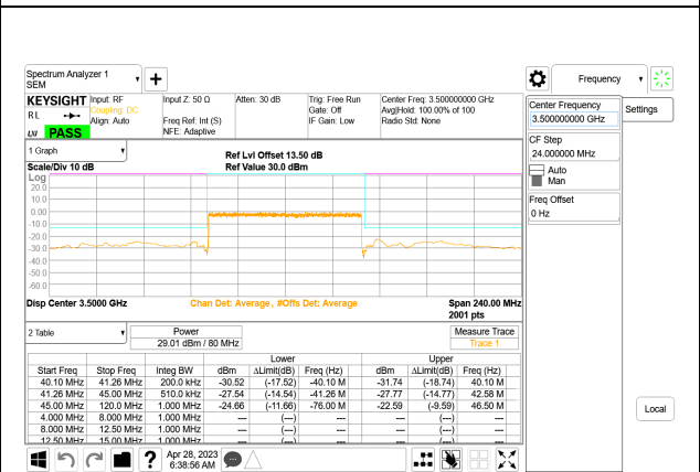
5G NR n77 80MHz BPSK Middle Channel RB216-0, ID:28568
