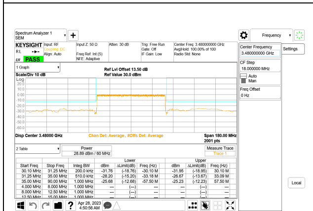
5G NR n77 60MHz BPSK Low Channel RB162-0, ID:28568
