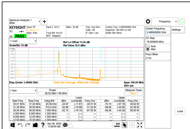
5G NR n77 60MHz BPSK Low Channel RB1-0, ID:28568
