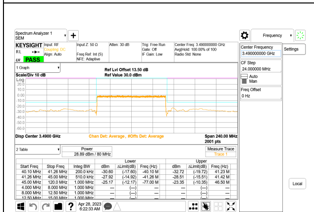
5G NR n77 80MHz BPSK Low Channel RB216-0, ID:28568
