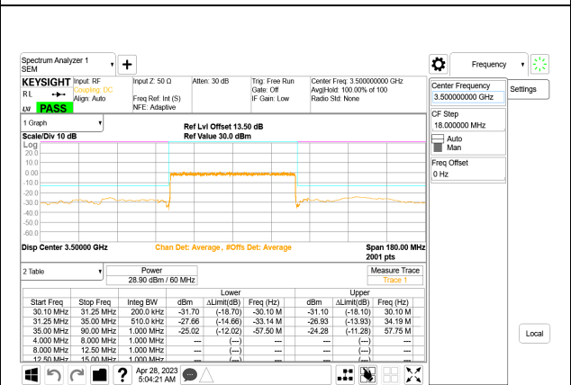
5G NR n77 60MHz BPSK Middle Channel RB162-0, ID:28568
