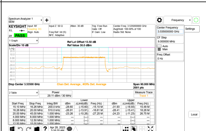
5G NR n77 30MHz BPSK High Channel RB75-0, ID:28568
