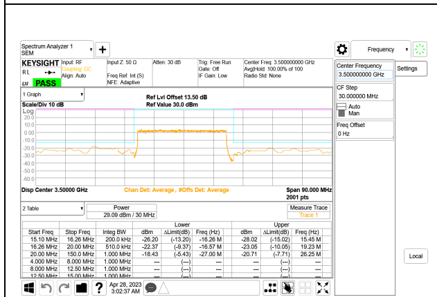
5G NR n77 30MHz BPSK Middle Channel RB75-0, ID:28568
