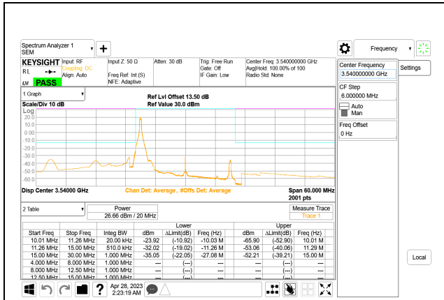
5G NR n77 20MHz BPSK High Channel RB1-0, ID:28568
