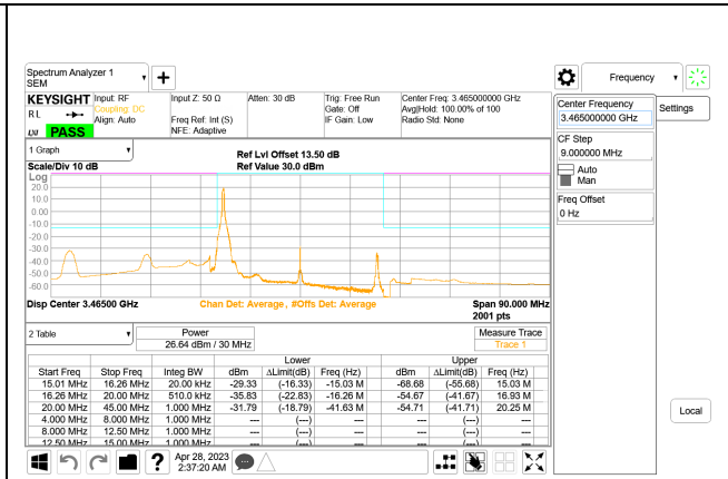
5G NR n77 30MHz BPSK Low Channel RB1-0, ID:28568
