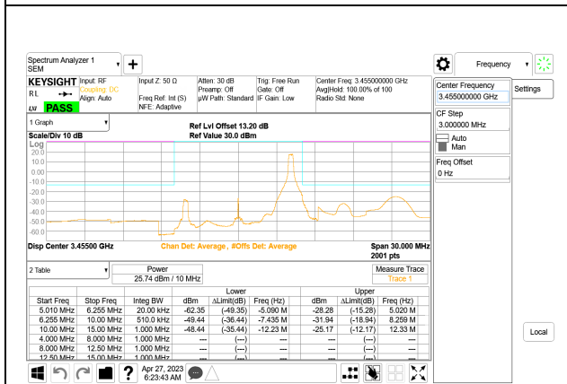
5G NR n77 10MHz BPSK Low Channel RB1-23, ID:28568
