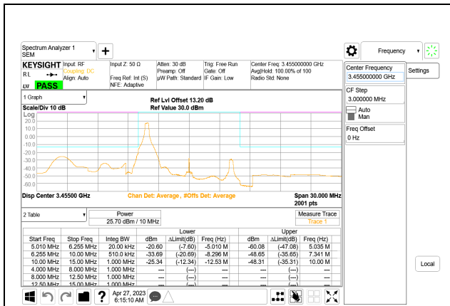
5G NR n77 10MHz BPSK Low Channel RB1-0, ID:28568
