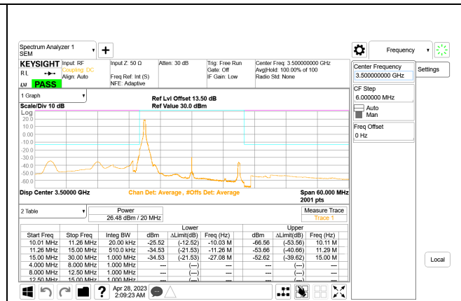
5G NR n77 20MHz BPSK Middle Channel RB1-0, ID:28568
