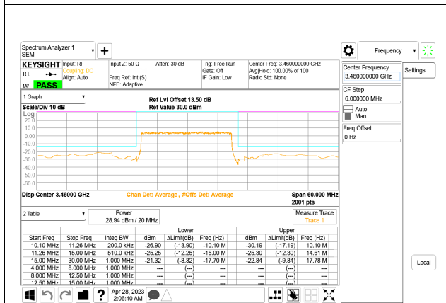
5G NR n77 20MHz BPSK Low Channel RB50-0, ID:28568
