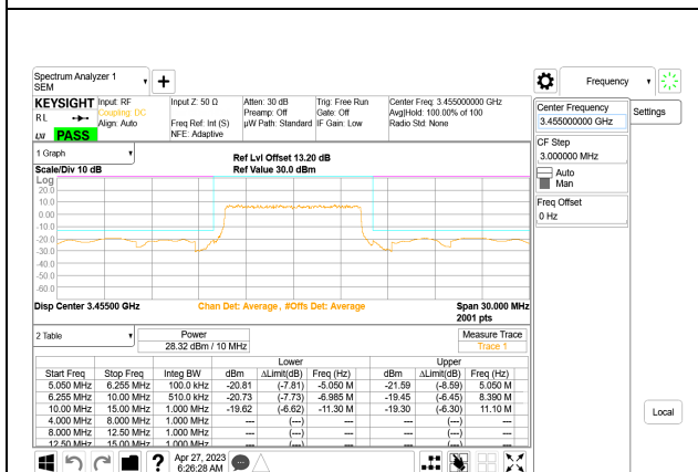
5G NR n77 10MHz BPSK Low Channel RB24-0, ID:28568
