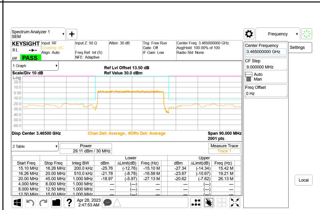
5G NR n77 30MHz BPSK Low Channel RB75-0, ID:28568
