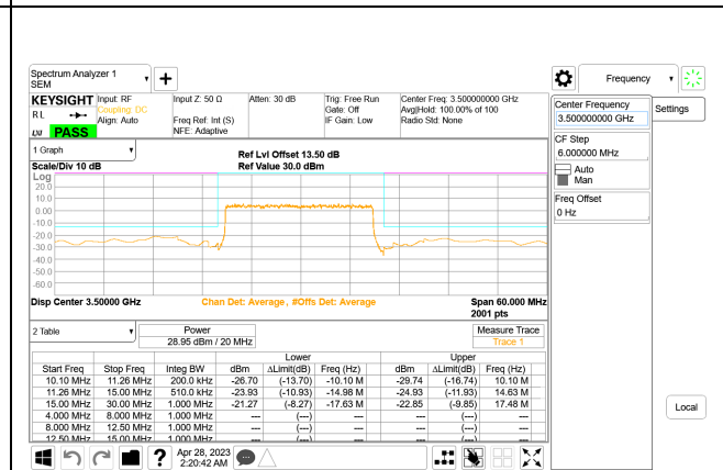
5G NR n77 20MHz BPSK Middle Channel RB50-0, ID:28568
