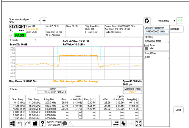
5G NR n77 20MHz BPSK High Channel RB50-0, ID:28568
