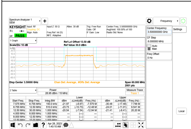
5G NR n77 15MHz BPSK Middle Channel RB36-0, ID:28568
