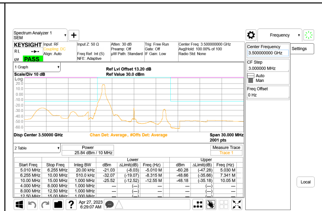
5G NR n77 10MHz BPSK Middle Channel RB1-0, ID:28568
