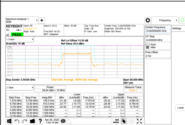
5G NR n77 15MHz BPSK High Channel RB36-0, ID:28568
