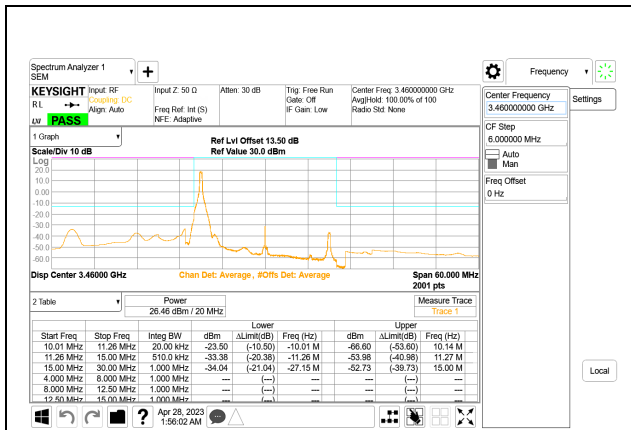
5G NR n77 20MHz BPSK Low Channel RB1-0, ID:28568
