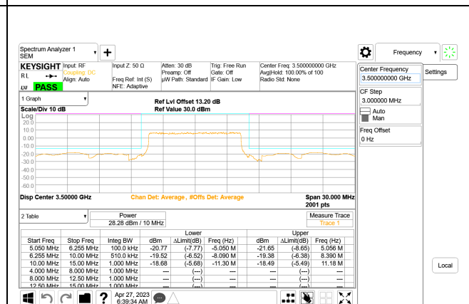
5G NR n77 10MHz BPSK Middle Channel RB24-0, ID:28568
