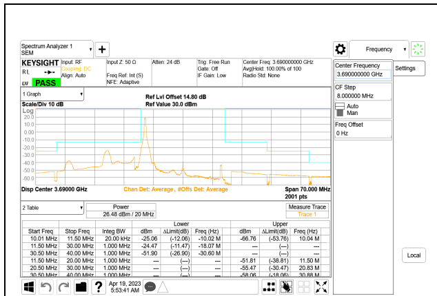
5G NR n48 20MHz BPSK High Channel RB1-0, ID:28567
