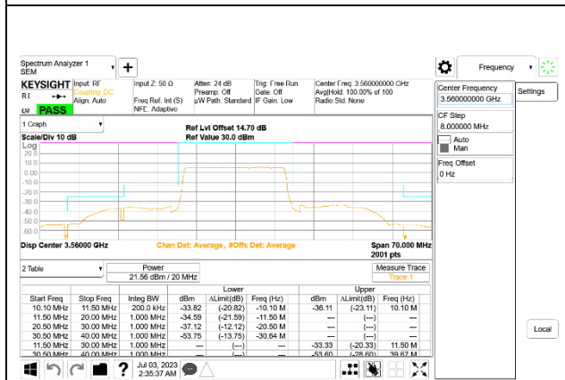
5G NR n48 20MHz BPSK Low Channel RB50-0, ID:28567
