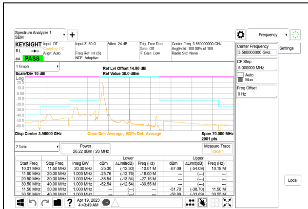
5G NR n48 20MHz BPSK Low Channel RB1-0, ID:28567
