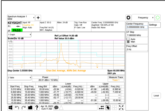
5G NR n48 10MHz BPSK Low Channel RB1-0, ID:28567
