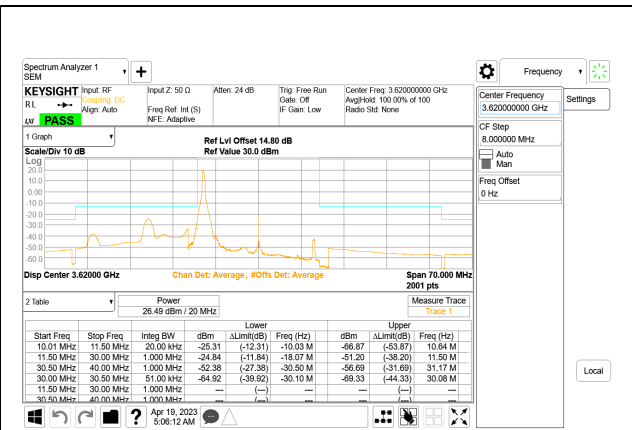
5G NR n48 20MHz BPSK Middle Channel RB1-0, ID:28567
