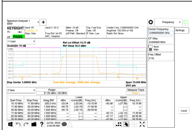
5G NR n48 20MHz BPSK High Channel RB50-0, ID:28567
