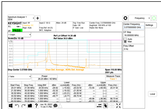
5G NR n48 40MHz BPSK Low Channel RB1-0, ID:32586
