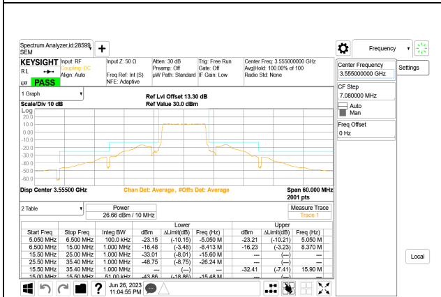
5G NR n48 10MHz BPSK Low Channel RB24-0
