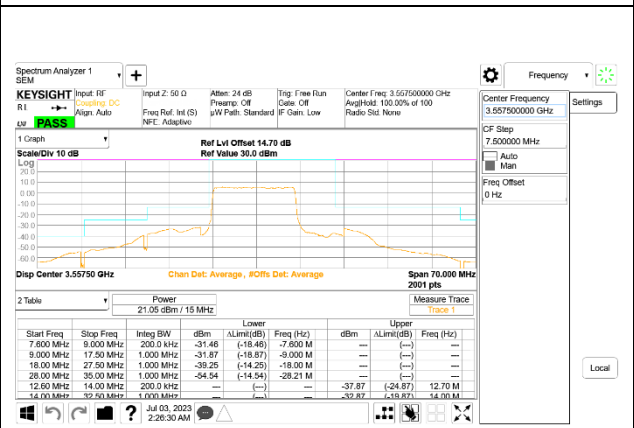
5G NR n48 15MHz BPSK Low Channel RB36-0, ID:28567
