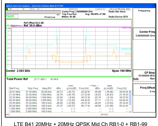
LTE B41 20MHz + 20MHz QPSK Mid Ch RB1-0 + RB1-99
