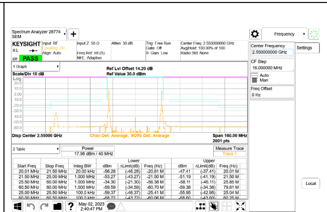
LTE B7 20MHz + 20MHz 16QAM High Ch RB1-0 + RB1-99
