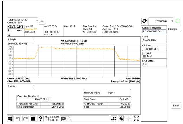
LTE B41 5MHz + 20MHz QPSK RB25-0 + RB100-0
