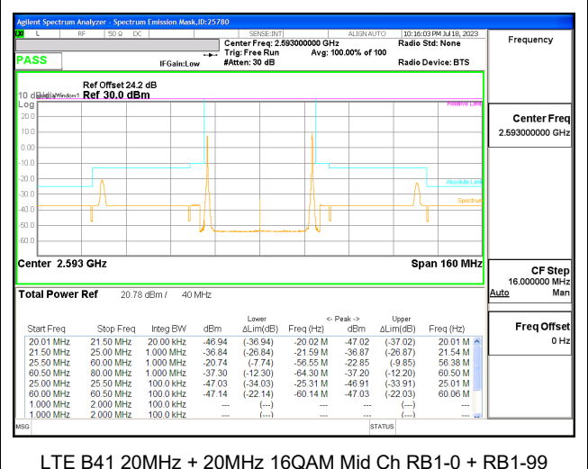
LTE B41 20MHz + 20MHz 16QAM Mid Ch RB1-0 + RB1-99
