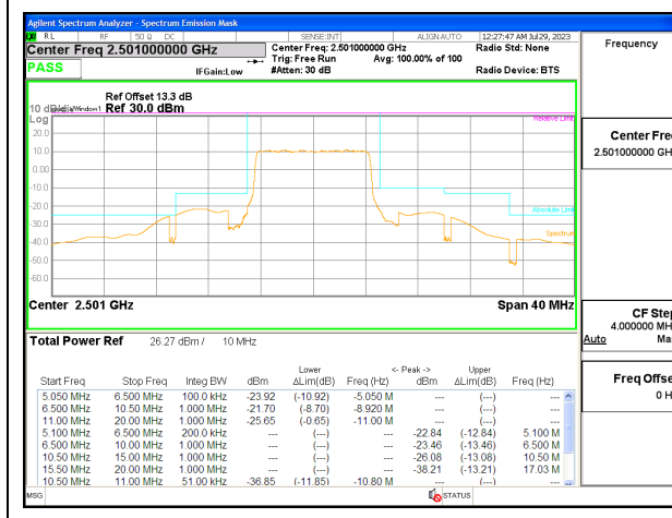
5G NR n41 10MHz BPSK Low Channel RB24-0, ID:12482
