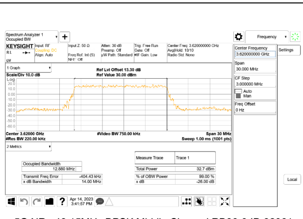
5G NR n48 15MHz BPSK Middle Channel RB36-0 ID:32061
