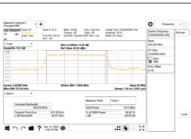
5G NR n48 30MHz BPSK Middle Channel RB75-0 ID:32061
