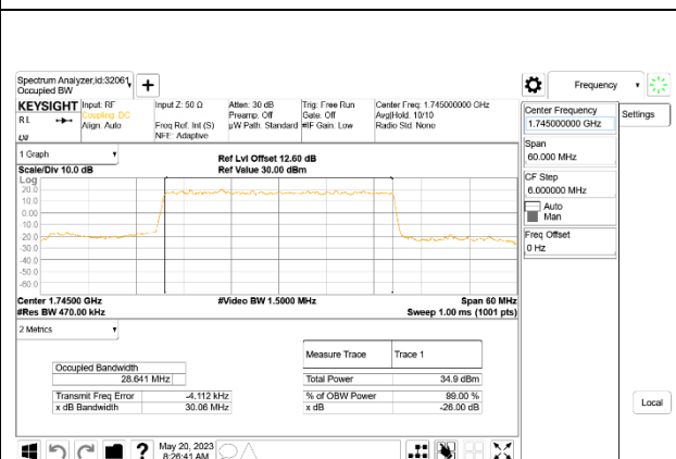
5G NR n66 35MHz BPSK Middle Channel RB160-0
