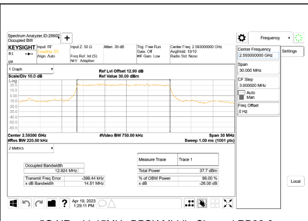
5G NR n41 15MHz BPSK Middle Channel RB36-0
