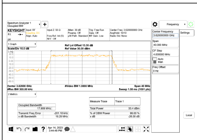
5G NR n48 20MHz BPSK Middle Channel RB50-0, ID:32061
