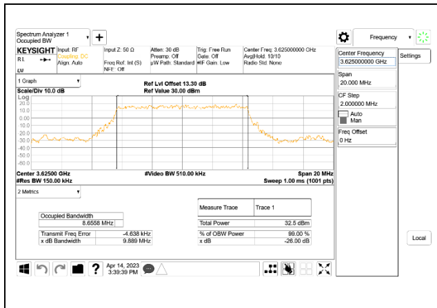
5G NR n48 10MHz BPSK Middle Channel RB24-0, ID:32061
