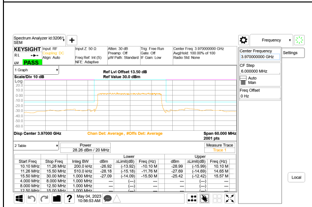
5G NR n77 20MHz BPSK High Channel RB50-0
