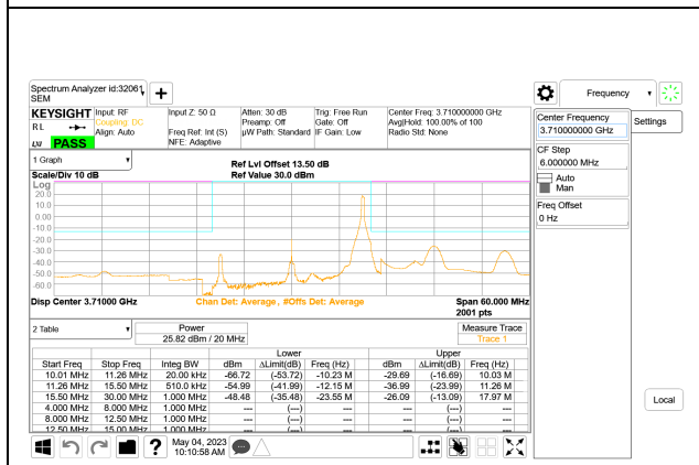
5G NR n77 20MHz BPSK Low Channel RB1-50
