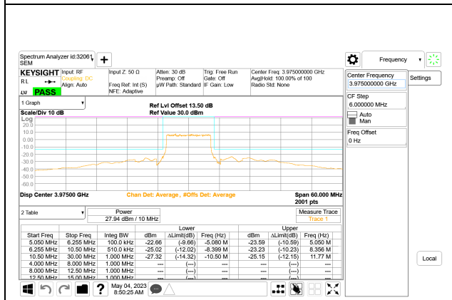
5G NR n77 10MHz BPSK High Channel RB24-0
