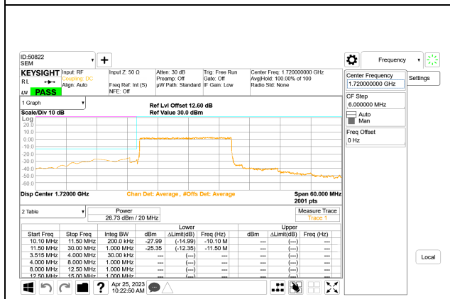
5G NR n66 20MHz BPSK Low Channel RB100-0
