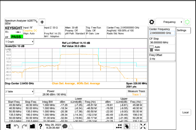
5G NR n41 90MHz BPSK High Channel RB243-0
