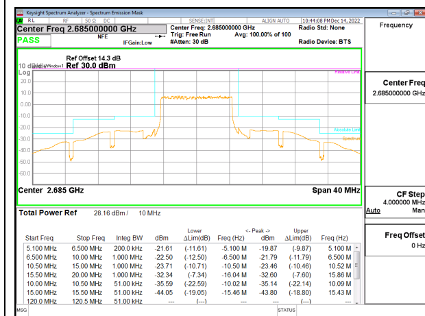
5G NR n41 10MHz BPSK High Channel RB24-0, ID:25780
