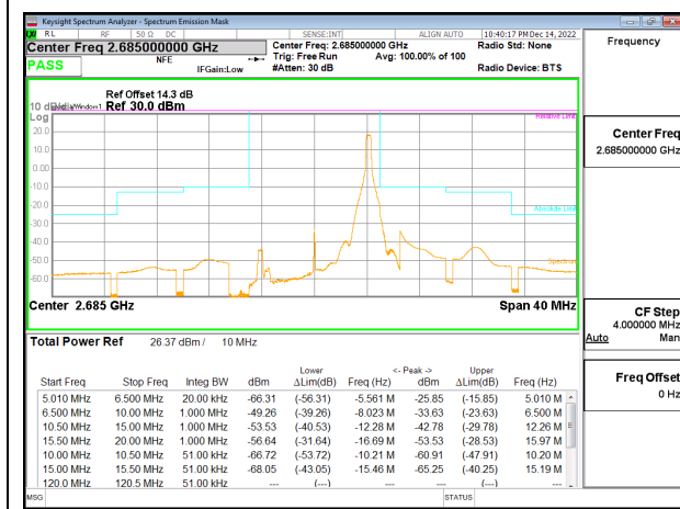
5G NR n41 10MHz BPSK High Channel RB1-23, ID:25780
