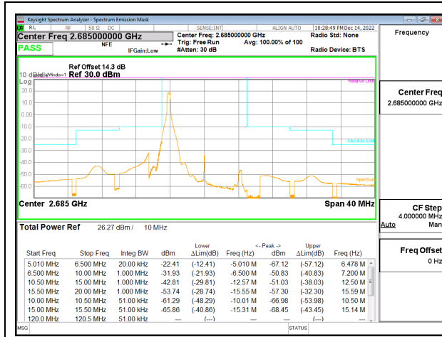
5G NR n41 10MHz BPSK High Channel RB1-0, ID:25780
