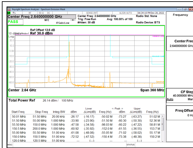
5G NR n41 100MHz BPSK High Channel RB1-0, ID:25780
