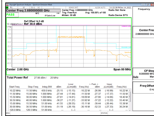
5G NR n41 20MHz BPSK High Channel RB50-0, ID:25780
