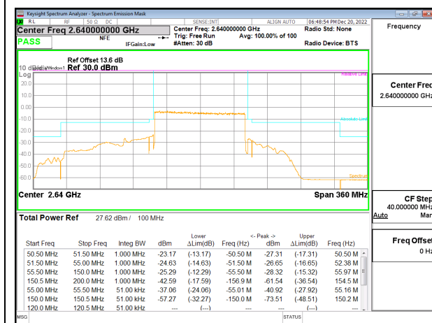
5G NR n41 100MHz BPSK High Channel RB270-0, ID:25780
