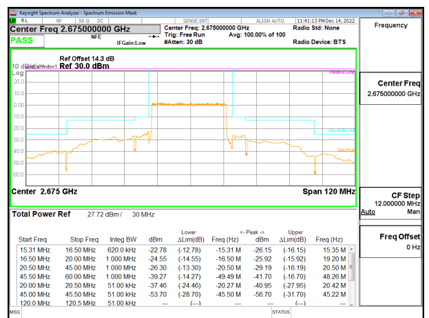
5G NR n41 30MHz BPSK High Channel RB75-0, ID:25780
