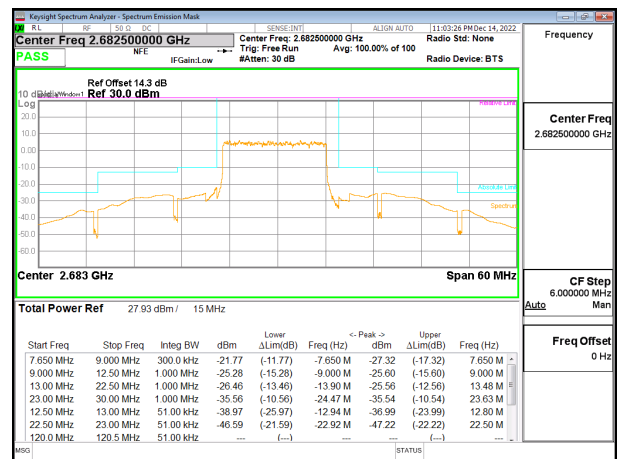
5G NR n41 15MHz BPSK High Channel RB36-0, ID:25780
