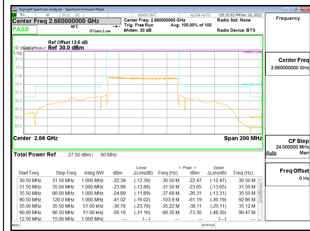
5G NR n41 60MHz BPSK High Channel RB162-0, ID:25780
