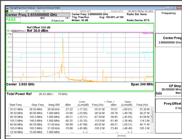
5G NR n41 70MHz BPSK High Channel RB1-0, ID:25780
