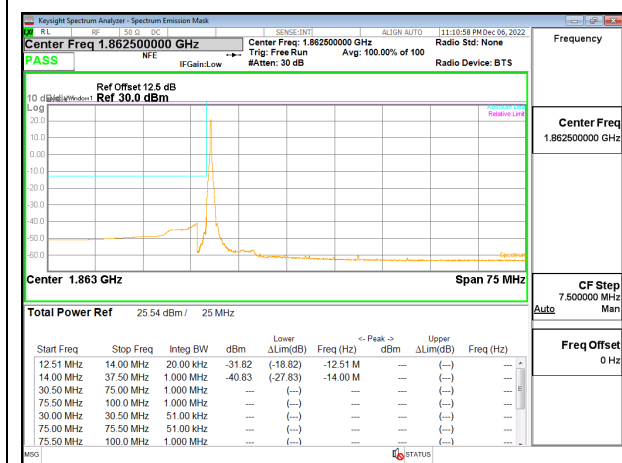
5G NR n25 25MHz BPSK Low Channel RB1-0, ID:19146
