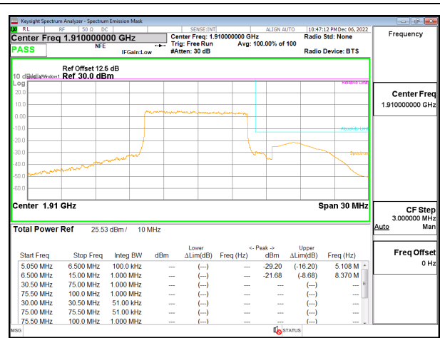
5G NR n25 10MHz BPSK High Channel RB50-0, ID:19146
