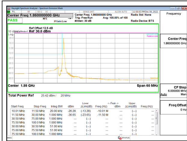
5G NR n25 20MHz BPSK Low Channel RB1-0, ID:19146
