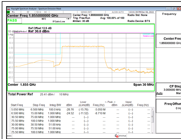
5G NR n25 10MHz BPSK Low Channel RB50-0, ID:19146
