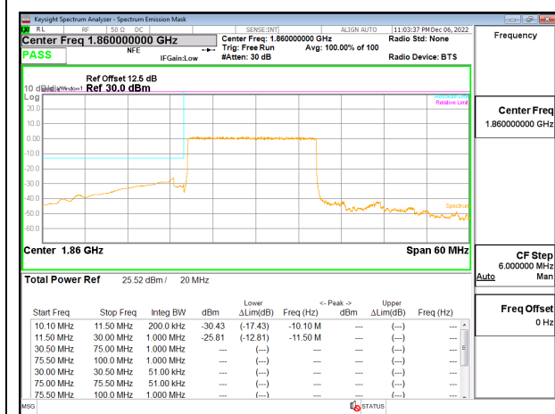
5G NR n25 20MHz BPSK Low Channel RB100-0, ID:19146
