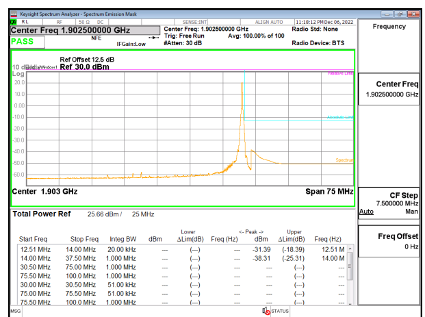
5G NR n25 25MHz BPSK High Channel RB132-0, ID:19146
