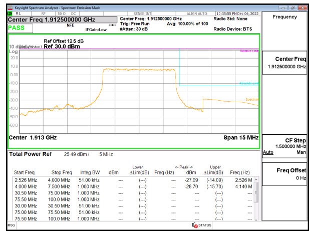
5G NR n25 5MHz BPSK High Channel RB25-0, ID:19146
