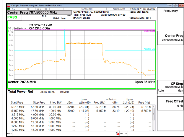
5G NR n12 10MHz BPSK Middle Channel RB50-0, ID:19146
