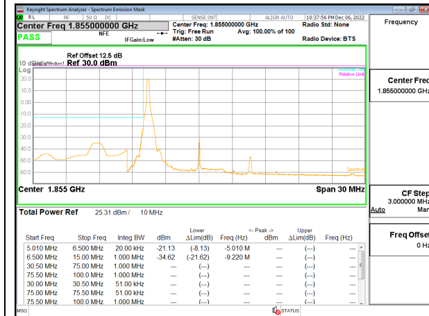
5G NR n25 10MHz BPSK Low Channel RB1-0, ID:19146
