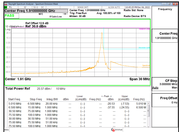
5G NR n25 10MHz BPSK High Channel RB1-51, ID:19146
