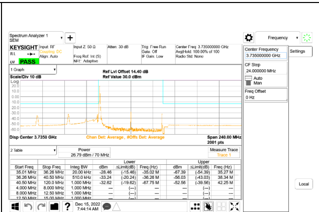
5G NR n77 70MHz BPSK Low Channel RB1-0, ID:50822
