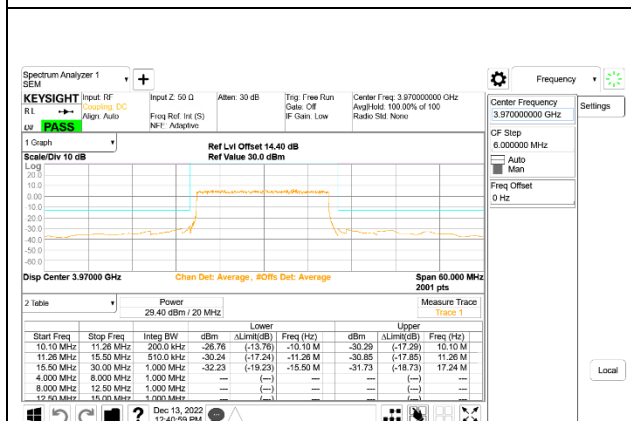
5G NR n77 20MHz BPSK High Channel RB50-0, ID:50822
