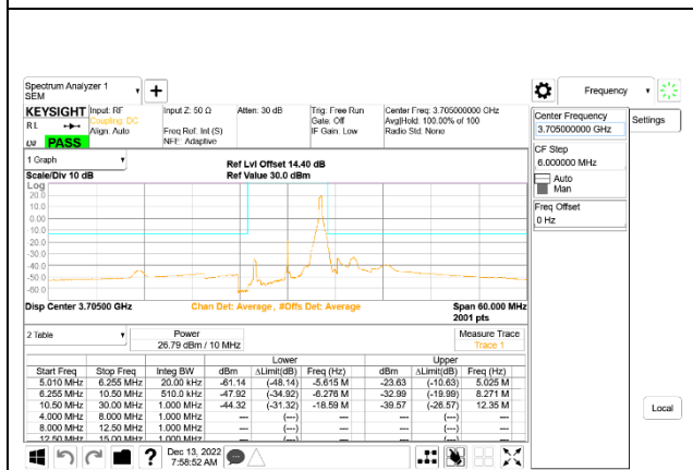
5G NR n77 10MHz BPSK Low Channel RB1-23, ID:50822
