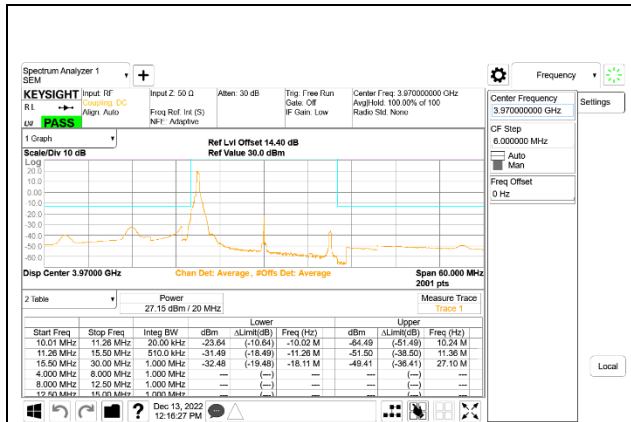
5G NR n77 20MHz BPSK High Channel RB1-0, ID:50822
