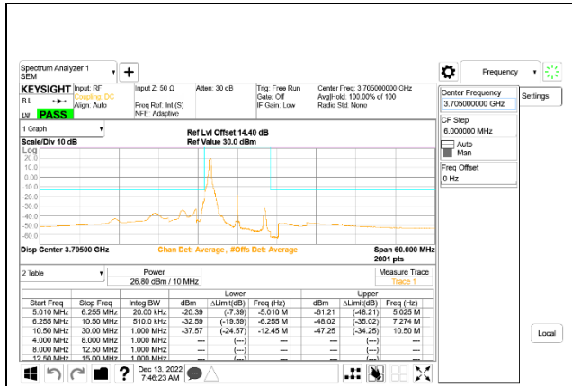
5G NR n77 10MHz BPSK Low Channel RB1-0, ID:50822
