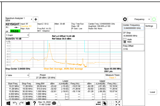
5G NR n77 20MHz BPSK Middle Channel RB1-0, ID:50822
