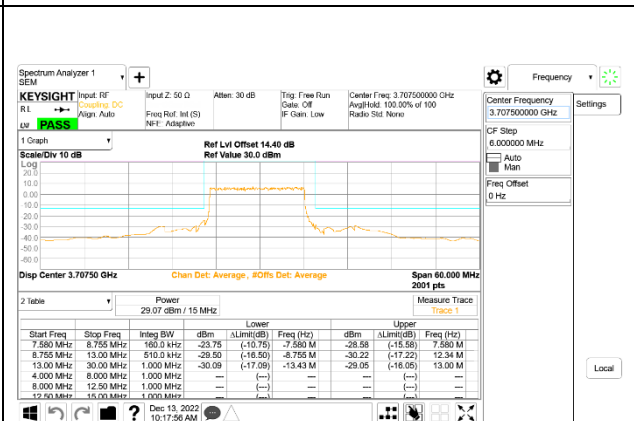
5G NR n77 15MHz BPSK Low Channel RB36-0, ID:50822
