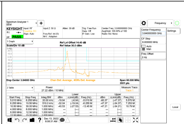
5G NR n77 10MHz BPSK Middle Channel RB1-0, ID:50822
