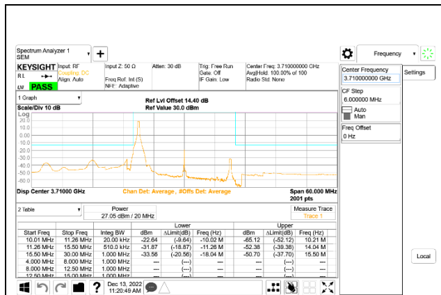
5G NR n77 20MHz BPSK Low Channel RB1-0, ID:50822
