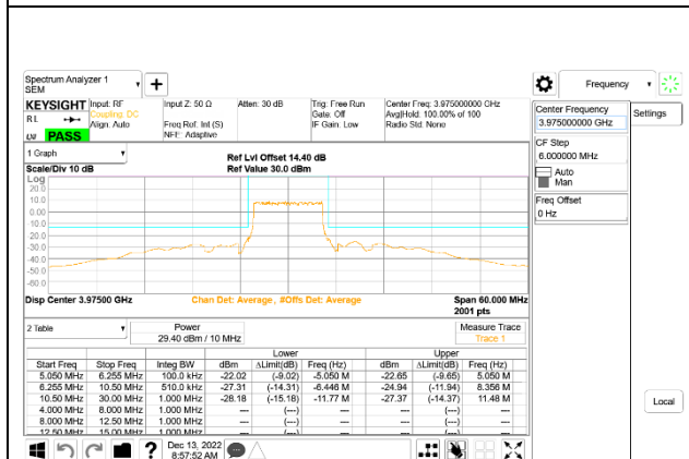
5G NR n77 10MHz BPSK High Channel RB24-0, ID:50822
