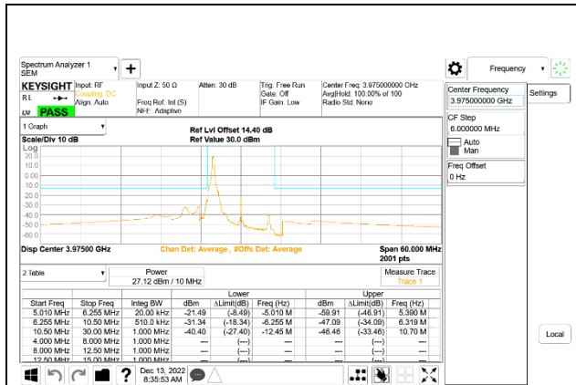
5G NR n77 10MHz BPSK High Channel RB1-0, ID:50822
