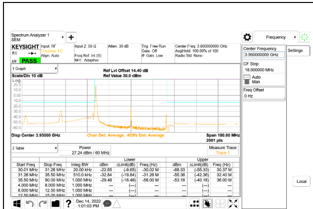
5G NR n77 60MHz BPSK High Channel RB1-0, ID:50822
