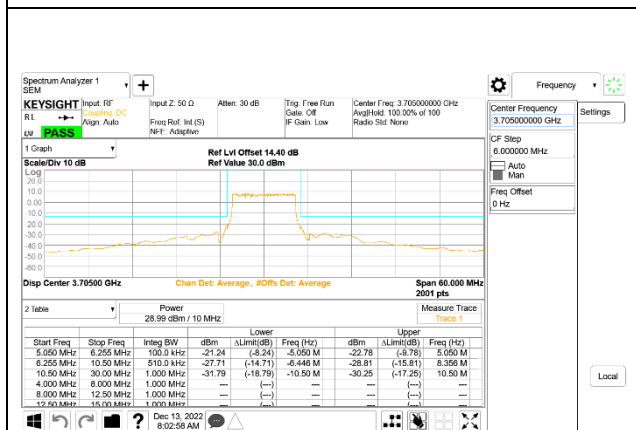
5G NR n77 10MHz BPSK Low Channel RB24-0, ID:50822
