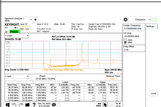
5G NR n77 70MHz BPSK Low Channel RB1-188, ID:50822
