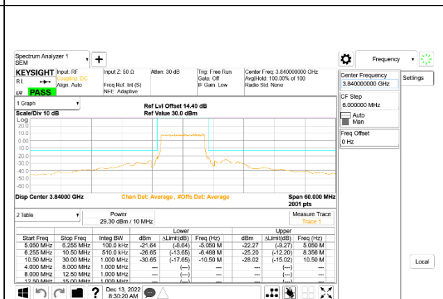
5G NR n77 10MHz BPSK Middle Channel RB24-0, ID:50822
