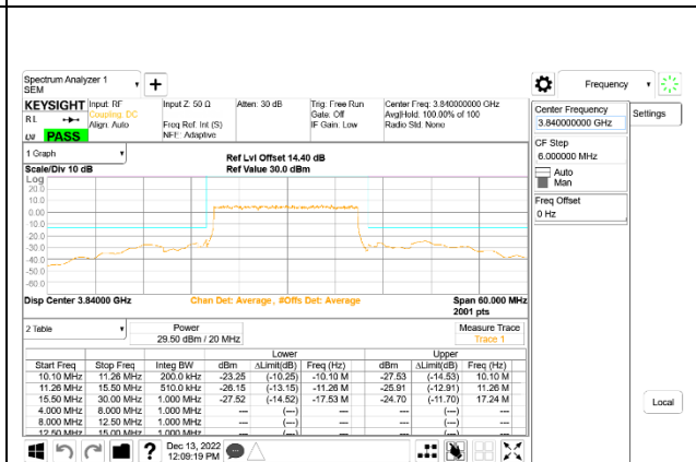
5G NR n77 20MHz BPSK Middle Channel RB50-0, ID:50822
