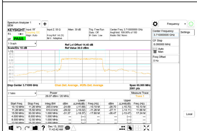
5G NR n77 20MHz BPSK Low Channel RB50-0, ID:50822
