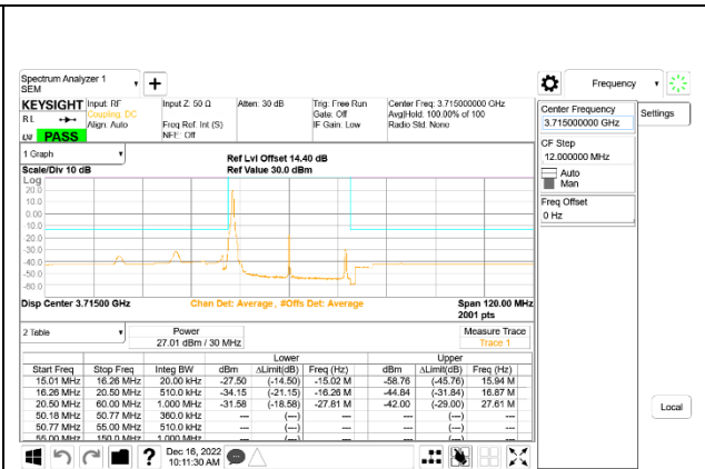
5G NR n77 30MHz BPSK Low Channel RB1-0, ID:50822
