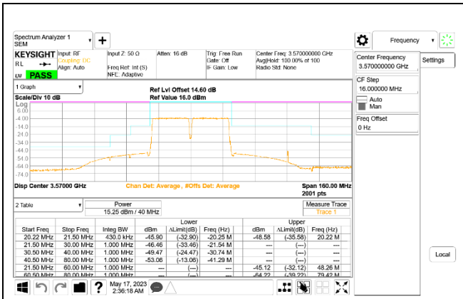
LTE B48 20MHz + 20MHz QPSK Low Ch RB100-0 + RB100-0 ID:27342
