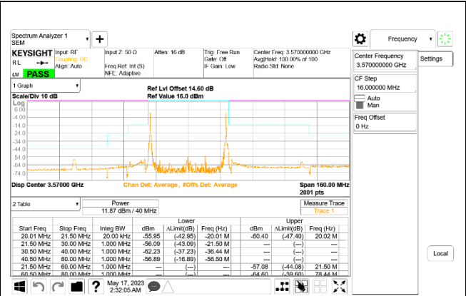
LTE B48 20MHz + 20MHz 16QAM Low Ch RB1-0 + RB1-99 ID:27342
