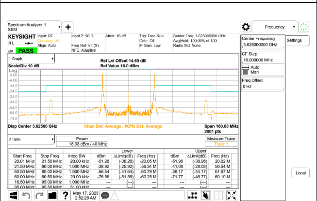
LTE B48 20MHz + 20MHz 16QAM Mid Ch RB1-0 + RB1-99 ID:27342
