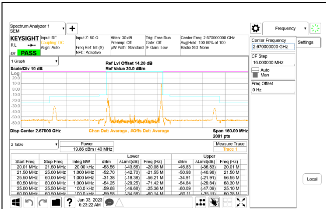
LTE B41 20MHz + 20MHz QPSK High Ch RB1-0 + RB1-99 ID:27342
