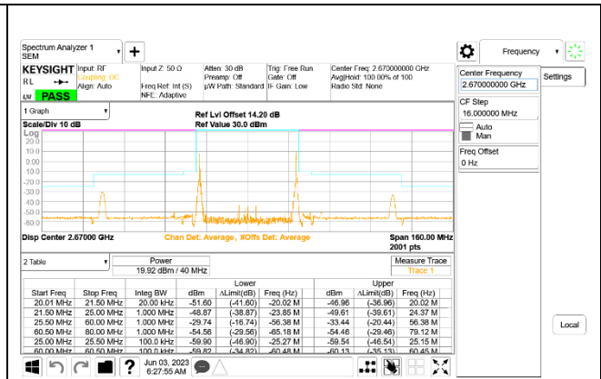
LTE B41 20MHz + 20MHz 16QAM High Ch RB1-0 + RB1-99 ID:27342
