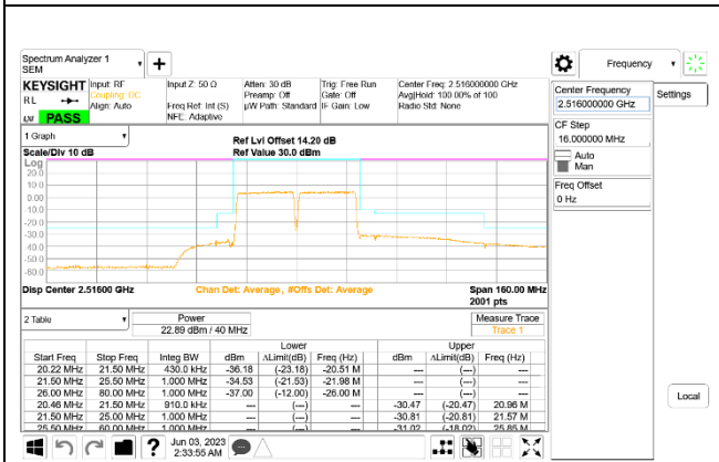
LTE B41 20MHz + 20MHz QPSK Low Ch RB100-0 + RB100-0 ID:27342
