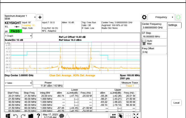
LTE B48 20MHz + 20MHz 16QAM High Ch RB1-0 + RB1-99 ID:27342
