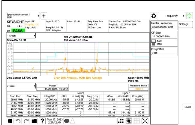
LTE B48 20MHz + 20MHz QPSK Low Ch RB1-0 + RB1-99 ID:27342
