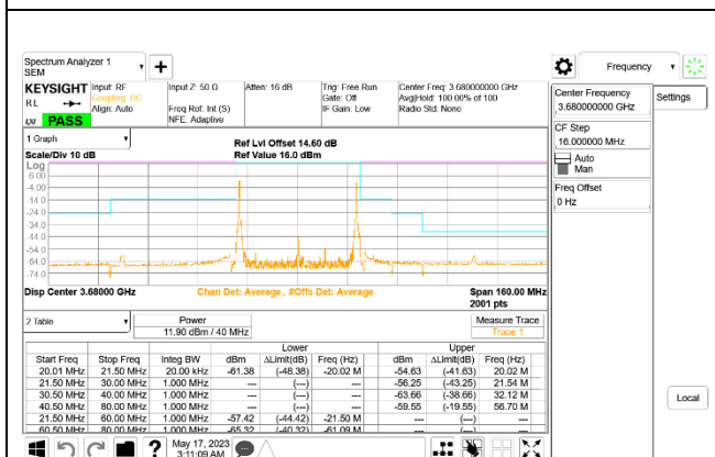
LTE B48 20MHz + 20MHz QPSK High Ch RB1-0 + RB1-99 ID:27342
