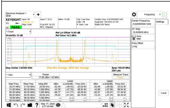
LTE B48 20MHz + 20MHz QPSK Mid Ch RB1-0 + RB1-99 ID:27342
