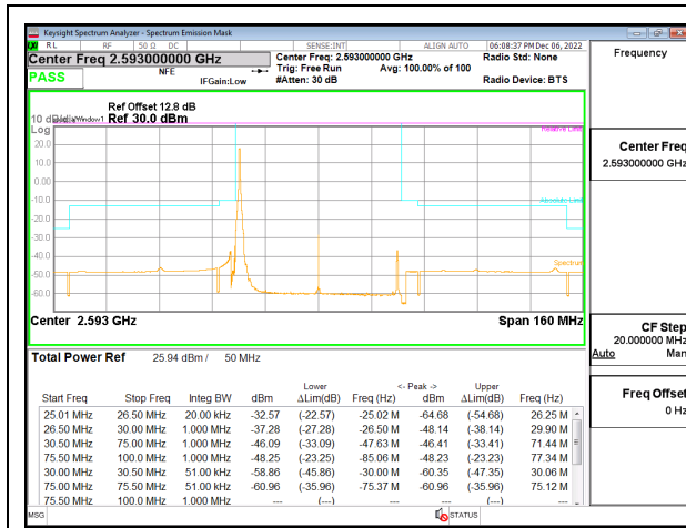
5G NR n41 50MHz BPSK Middle Channel RB1-0 ID:28498
