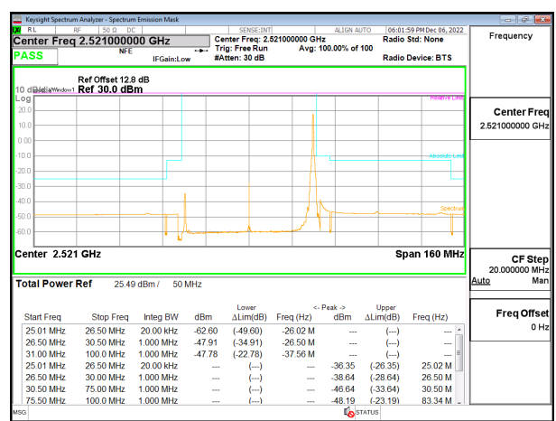
5G NR n41 50MHz BPSK Low Channel RB1-132 ID:28498
