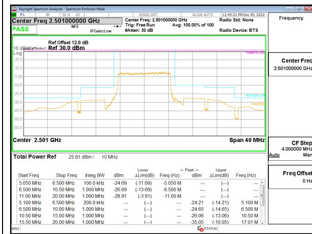
5G NR n41 10MHz BPSK Low Channel RB24-0 ID:28498
