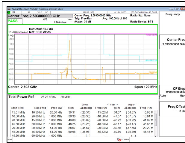
5G NR n41 30MHz BPSK Middle Channel RB1-0 ID:28498
