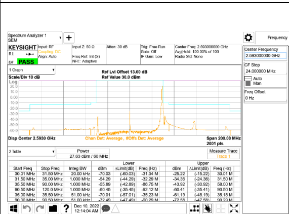
5G NR n41 60MHz BPSK Middle Channel RB1-161 ID:28498
