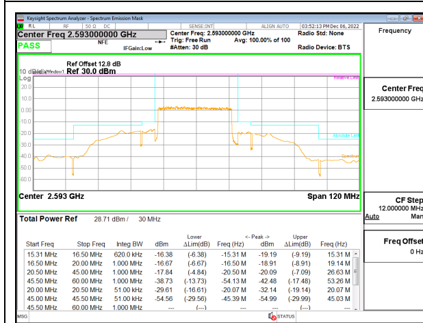
5G NR n41 30MHz BPSK Middle Channel RB75-0 ID:28498
