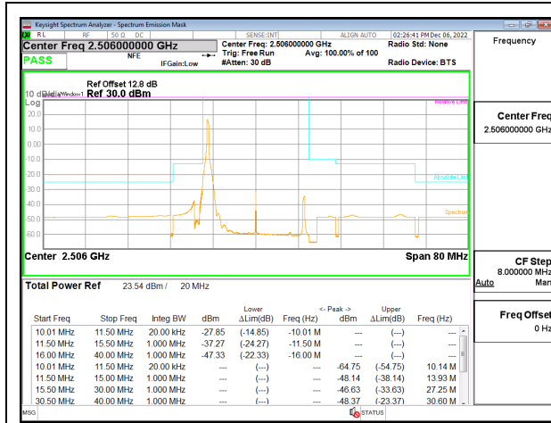
5G NR n41 20MHz BPSK Low Channel RB1-0 ID:28498
