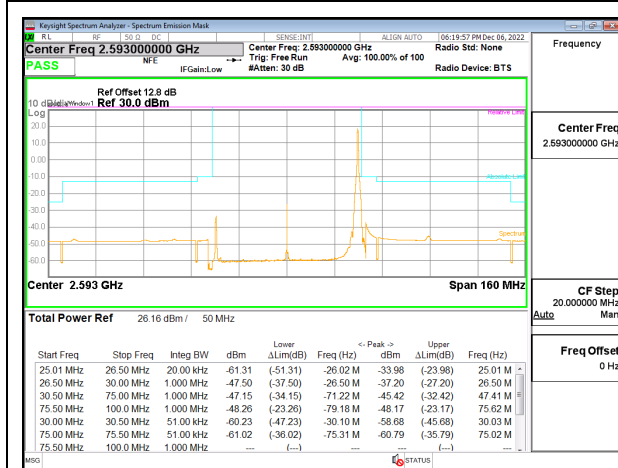
5G NR n41 50MHz BPSK Middle Channel RB1-132 ID:28498
