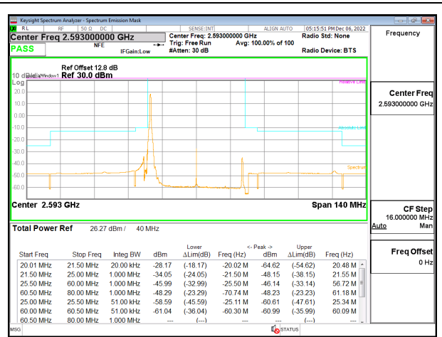
5G NR n41 40MHz BPSK Middle Channel RB1-0 ID:28498
