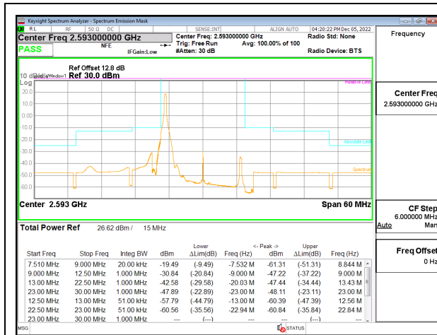
5G NR n41 15MHz BPSK Middle Channel RB1-0 ID:28498
