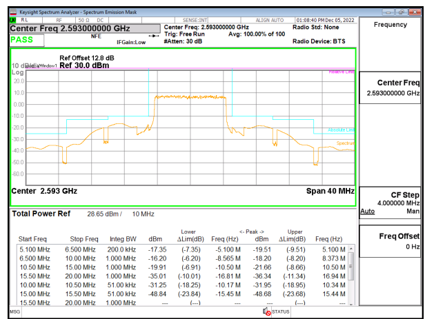
5G NR n41 10MHz BPSK Middle Channel RB24-0 ID:28498
