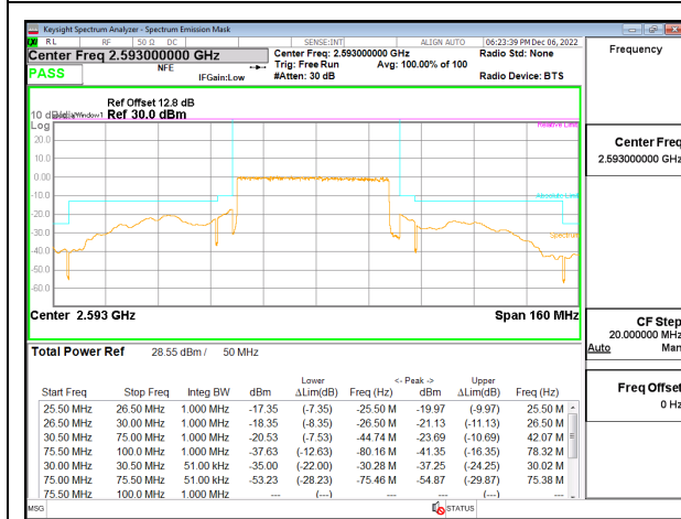
5G NR n41 50MHz BPSK Middle Channel RB128-0 ID:28498
