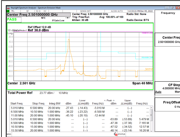
5G NR n41 10MHz BPSK Low Channel RB1-0 ID:28498
