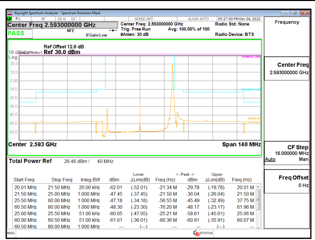
5G NR n41 40MHz BPSK Middle Channel RB1-105 ID:28498
