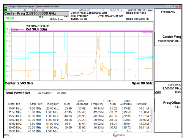
5G NR n41 20MHz BPSK Middle Channel RB1-50 ID:28498
