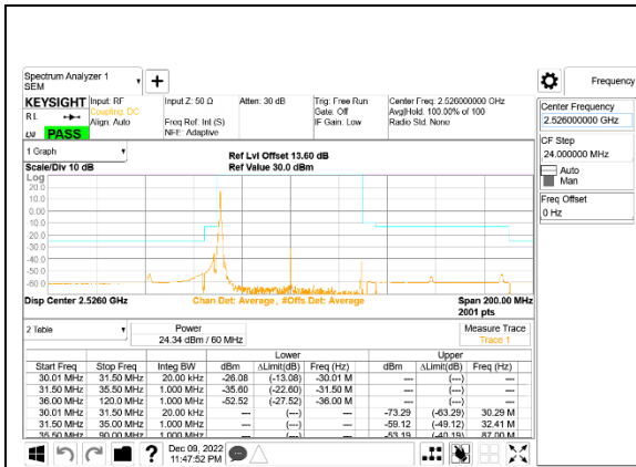
5G NR n41 60MHz BPSK Low Channel RB1-0 ID:28498
