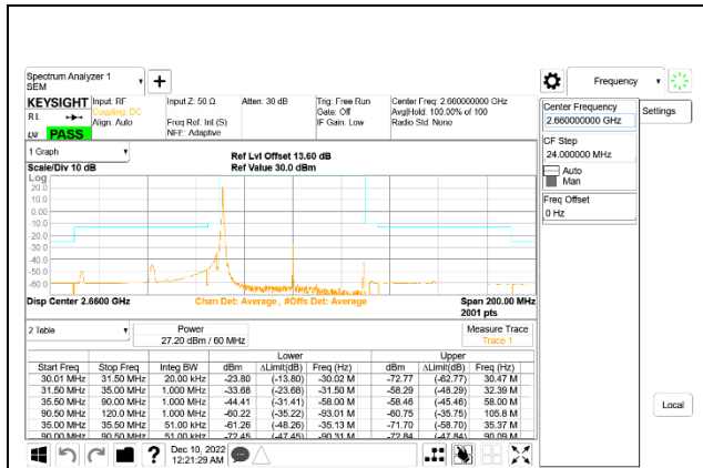
5G NR n41 60MHz BPSK High Channel RB1-0 ID:28498
