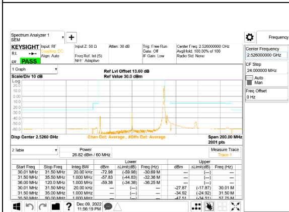
5G NR n41 60MHz BPSK Low Channel RB1-161 ID:28498
