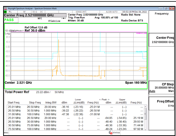
5G NR n41 50MHz BPSK Low Channel RB1-0 ID:28498
