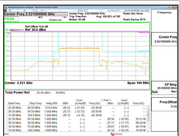
5G NR n41 50MHz BPSK Low Channel RB128-0 ID:28498
