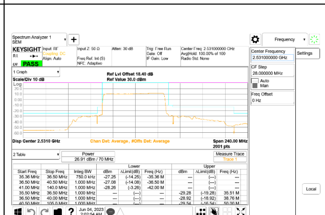
5G NR n41 70MHz BPSK Low Channel RB180-0 ID:28498
