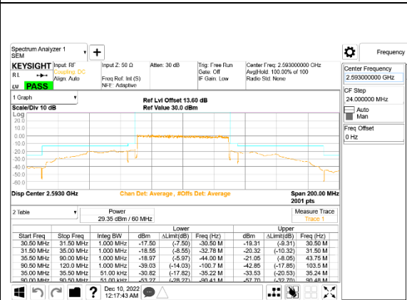
5G NR n41 60MHz BPSK Middle Channel RB162-0 ID:28498
