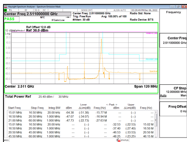
5G NR n41 30MHz BPSK Low Channel RB1-77 ID:28498
