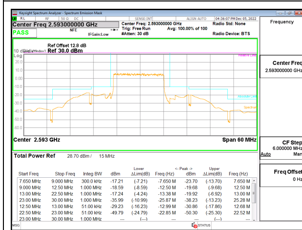
5G NR n41 15MHz BPSK Middle Channel RB36-0 ID:28498
