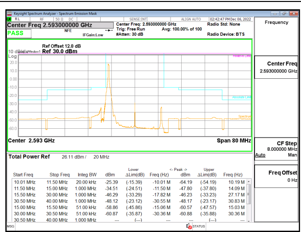
5G NR n41 20MHz BPSK Middle Channel RB1-0 ID:28498
