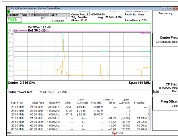
5G NR n41 40MHz BPSK Low Channel RB1-0 ID:28498
