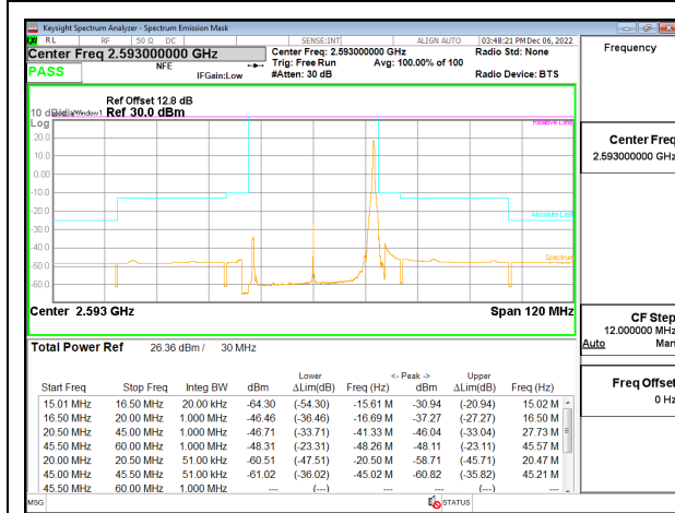
5G NR n41 30MHz BPSK Middle Channel RB1-77 ID:28498
