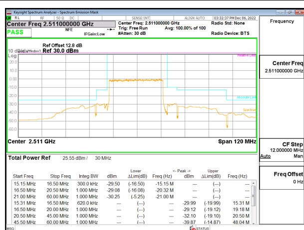
5G NR n41 30MHz BPSK Low Channel RB75-0 ID:28498
