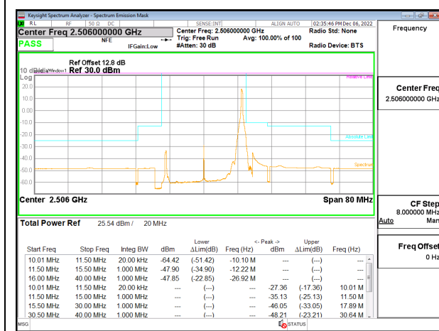
5G NR n41 20MHz BPSK Low Channel RB1-50 ID:28498
