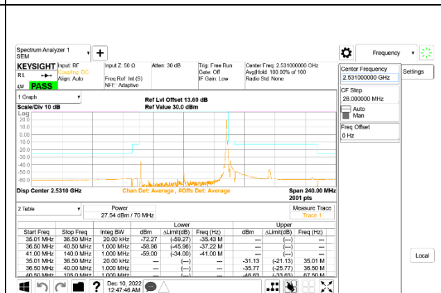
5G NR n41 70MHz BPSK Low Channel RB1-188 ID:28498
