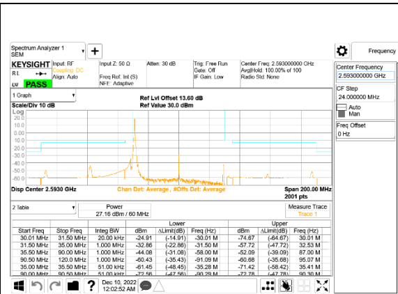
5G NR n41 60MHz BPSK Middle Channel RB1-0 ID:28498
