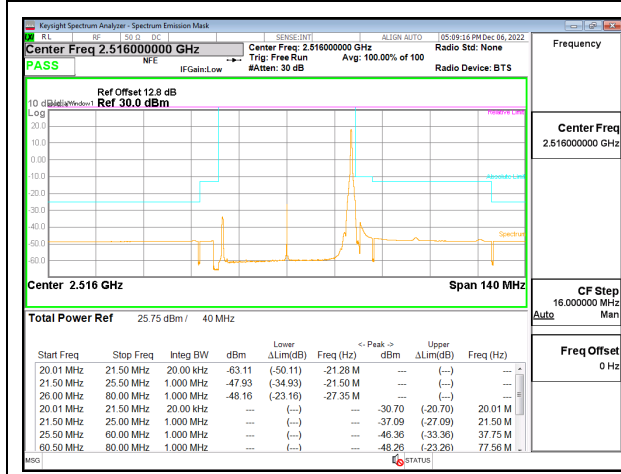
5G NR n41 40MHz BPSK Low Channel RB1-105 ID:28498
