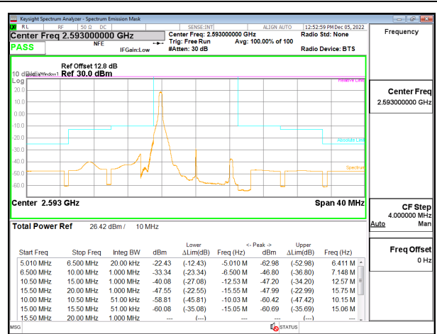
5G NR n41 10MHz BPSK Middle Channel RB1-0 ID:28498
