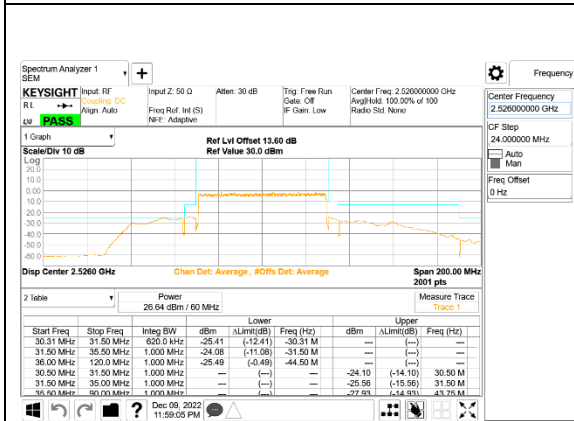
5G NR n41 60MHz BPSK Low Channel RB162-0 ID:28498
