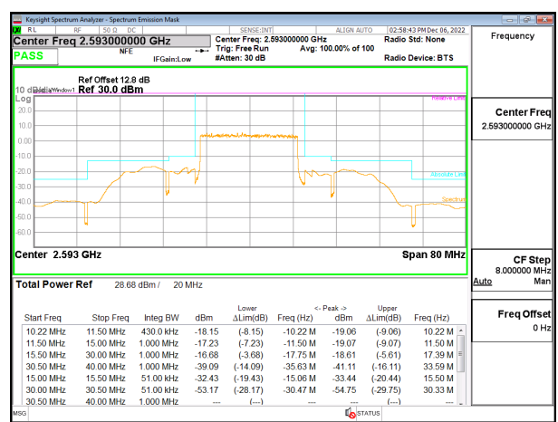
5G NR n41 20MHz BPSK Middle Channel RB50-0 ID:28498
