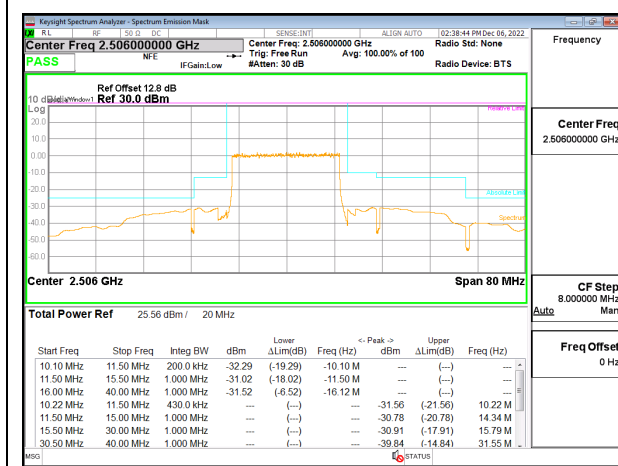
5G NR n41 20MHz BPSK Low Channel RB50-0 ID:28498
