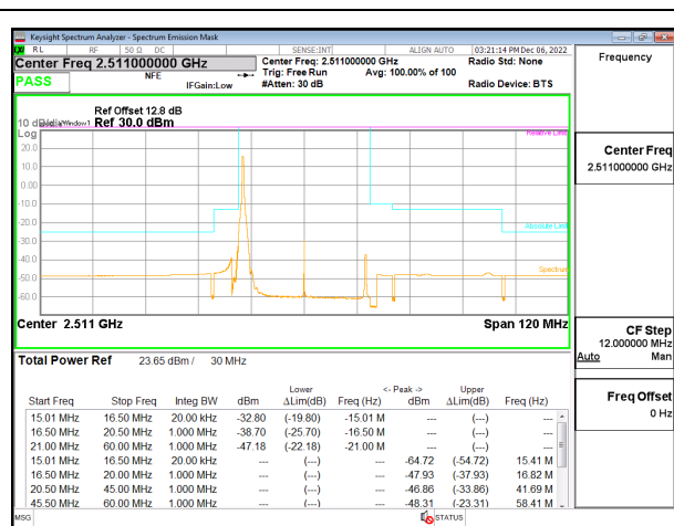
5G NR n41 30MHz BPSK Low Channel RB1-0 ID:28498
