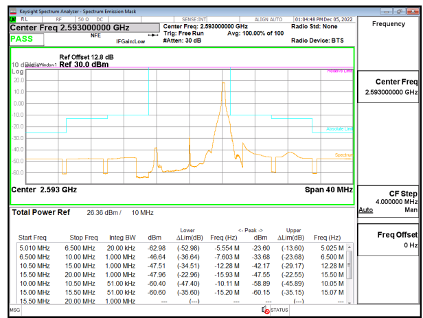
5G NR n41 10MHz BPSK Middle Channel RB1-23 ID:28498
