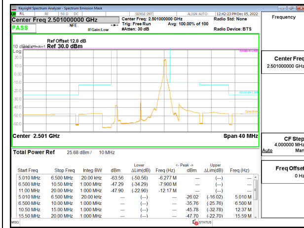
5G NR n41 10MHz BPSK Low Channel RB1-23 ID:28498
