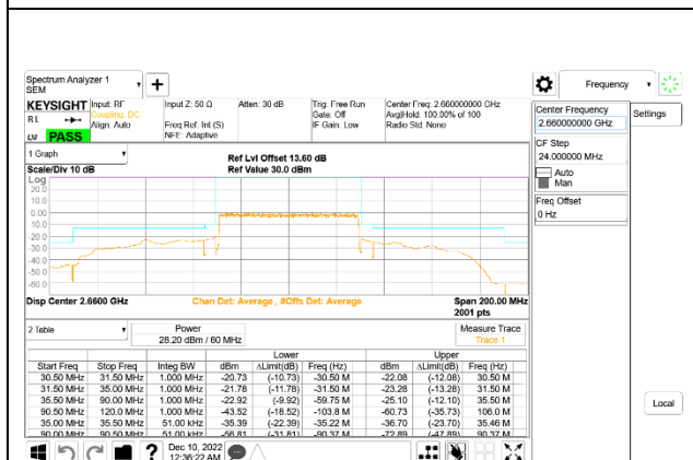
5G NR n41 60MHz BPSK High Channel RB162-0 ID:28498
