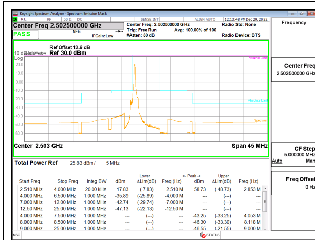
5G NR n7 5MHz BPSK Low Channel RB1-0, ID:28568
