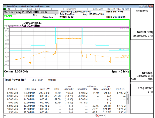
5G NR n7 10MHz BPSK Low Channel RB50-0, ID:28568
