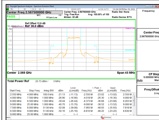
5G NR n7 5MHz BPSK High Channel RB25-0, ID:28568
