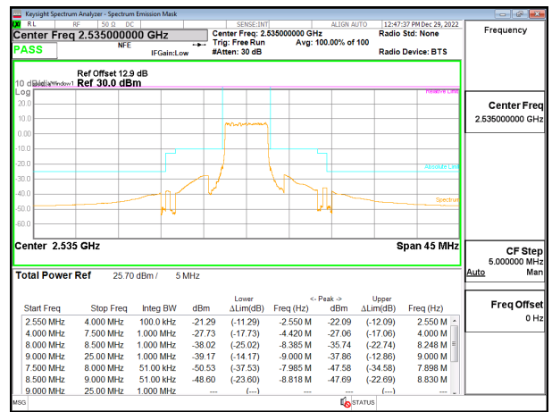
5G NR n7 5MHz BPSK Middle Channel RB25-0, ID:28568
