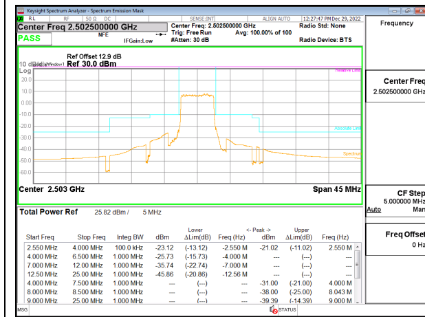
5G NR n7 5MHz BPSK Low Channel RB25-0, ID:28568
