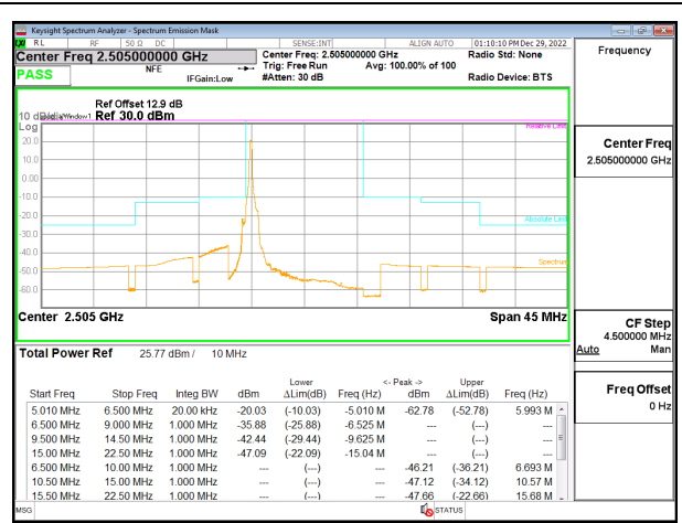
5G NR n7 10MHz BPSK Low Channel RB1-0, ID:28568
