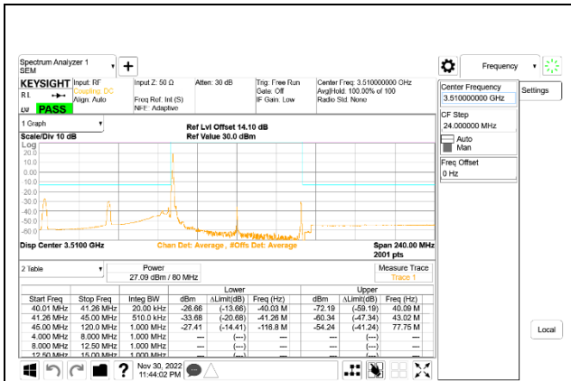
5G NR n77 80MHz BPSK High Channel RB1-0: ID 52275
