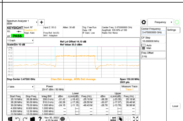
5G NR n77 50MHz BPSK Low Channel RB128-0: ID 52275
