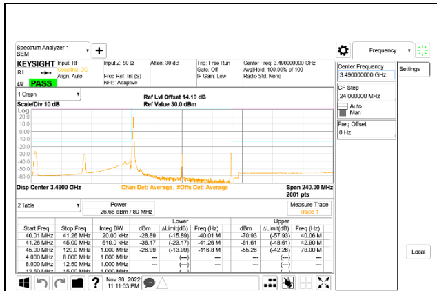
5G NR n77 80MHz BPSK Low Channel RB1-0: ID 52275
