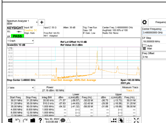
5G NR n77 60MHz BPSK Low Channel RB1-161: ID 52275
