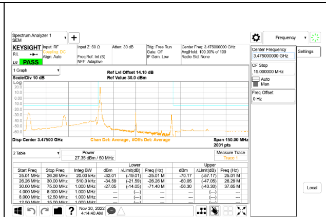
5G NR n77 50MHz BPSK Low Channel RB1-0: ID 52275
