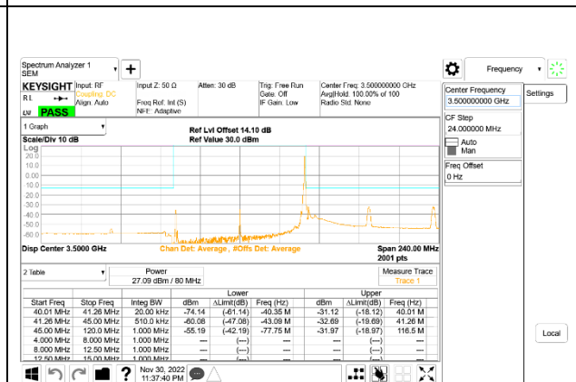
5G NR n77 80MHz BPSK Middle Channel RB1-216: ID 52275
