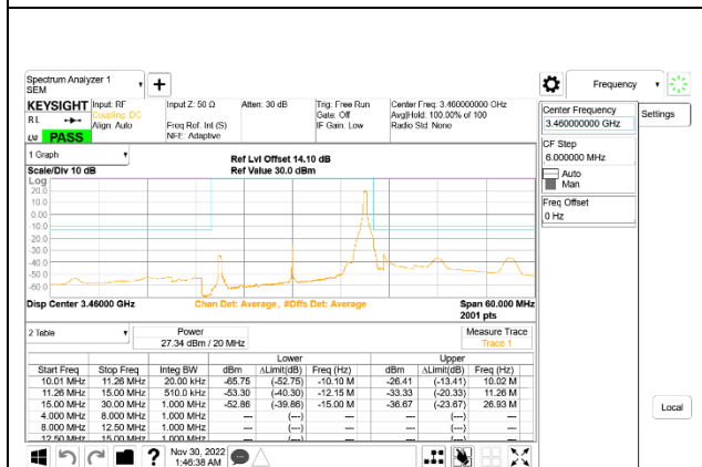
5G NR n77 20MHz BPSK Low Channel RB1-50: ID 52275
