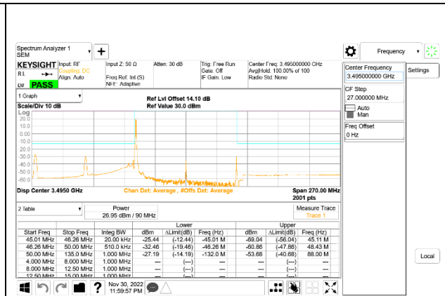
5G NR n77 90MHz BPSK Low Channel RB1-0: ID 52275
