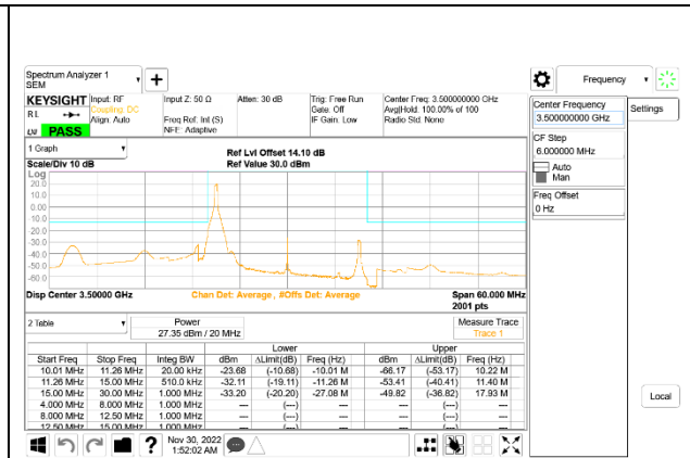
5G NR n77 20MHz BPSK Middle Channel RB1-0: ID 52275
