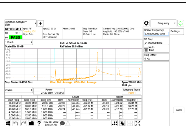
5G NR n77 70MHz BPSK Low Channel RB1-188: ID 52275
