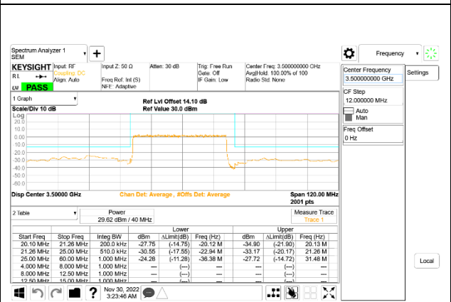
5G NR n77 40MHz BPSK Middle Channel RB100-0: ID 52275
