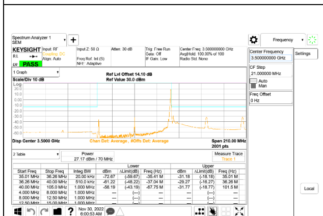
5G NR n77 70MHz BPSK Middle Channel RB1-188: ID 52275
