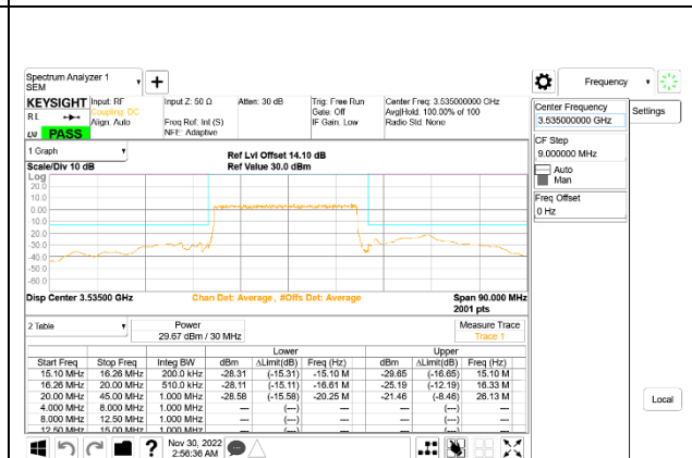
5G NR n77 30MHz BPSK High Channel RB75-0: ID 52275
