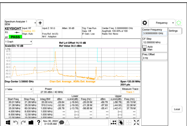
5G NR n77 40MHz BPSK Middle Channel RB1-0: ID 52275
