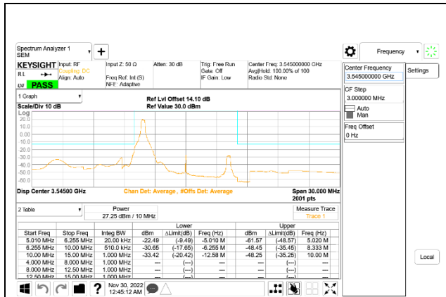
5G NR n77 10MHz BPSK High Channel RB1-0: ID 52275
