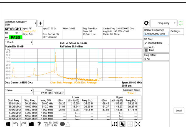
5G NR n77 70MHz BPSK Low Channel RB1-0: ID 52275
