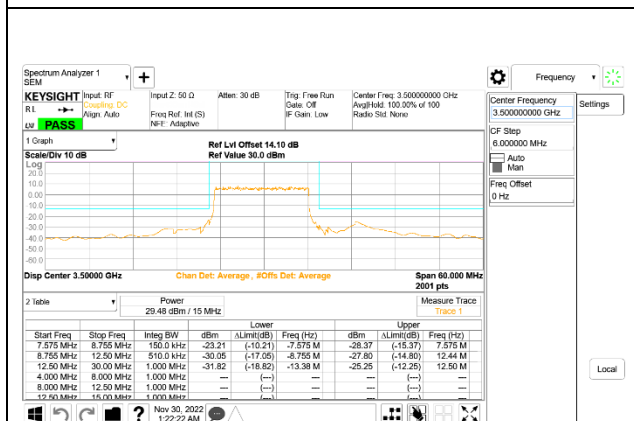
5G NR n77 15MHz BPSK Middle Channel RB36-0: ID 52275
