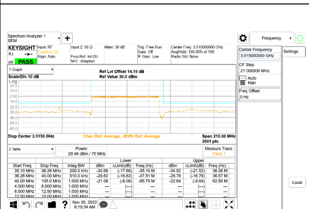
5G NR n77 70MHz BPSK High Channel RB180-0: ID 52275
