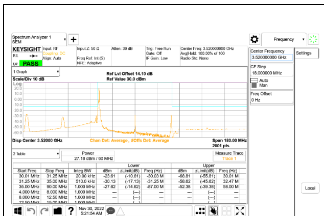
5G NR n77 60MHz BPSK High Channel RB1-0: ID 52275
