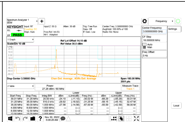
5G NR n77 60MHz BPSK Middle Channel RB1-0: ID 52275
