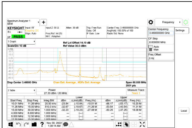
5G NR n77 20MHz BPSK Low Channel RB1-0: ID 52275
