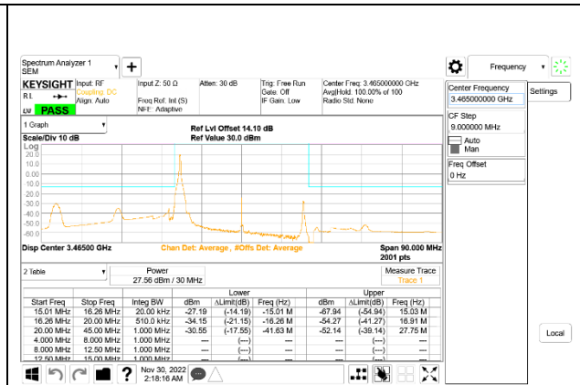
5G NR n77 30MHz BPSK Low Channel RB1-0: ID 52275
