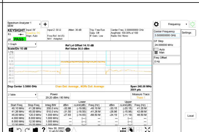
5G NR n77 80MHz BPSK Middle Channel RB216-0: ID 52275
