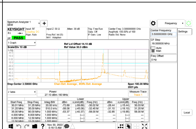
5G NR n77 60MHz BPSK Middle Channel RB1-161: ID 52275
