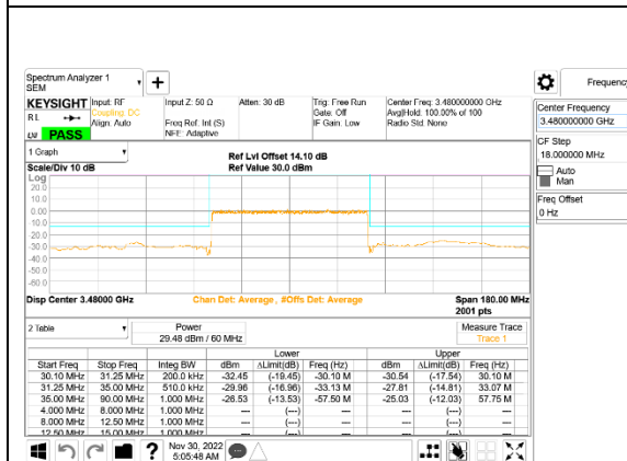
5G NR n77 60MHz BPSK Low Channel RB162-0: ID 52275
