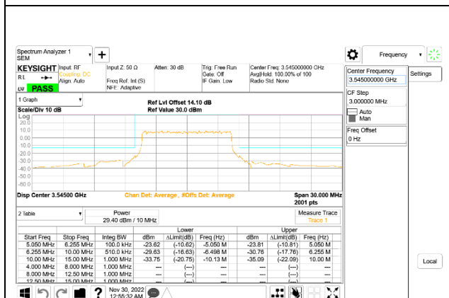
5G NR n77 10MHz BPSK High Channel RB24-0: ID 52275
