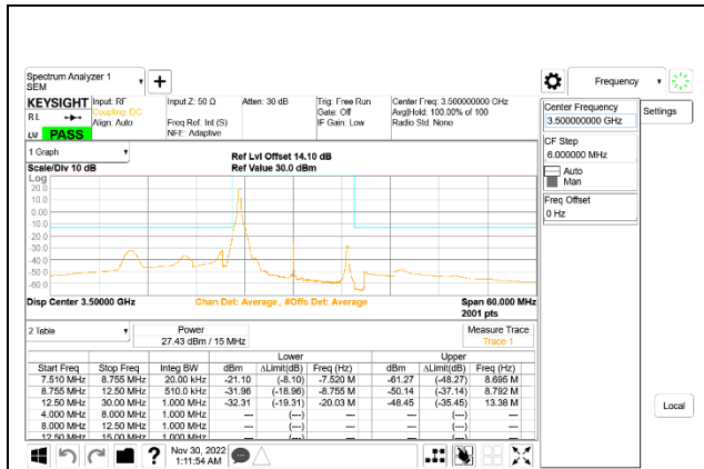
5G NR n77 15MHz BPSK Middle Channel RB1-0: ID 52275
