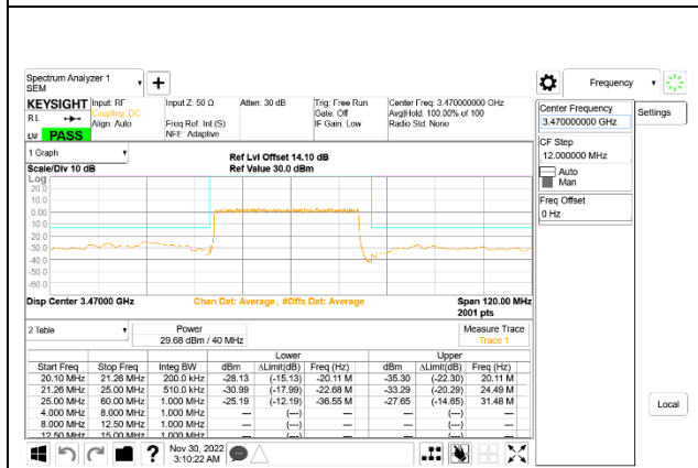
5G NR n77 40MHz BPSK Low Channel RB100-0: ID 52275
