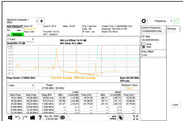
5G NR n77 30MHz BPSK Middle Channel RB1-0: ID 52275
