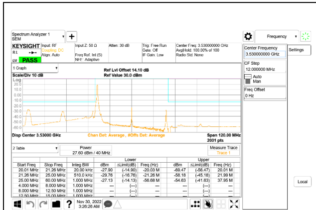
5G NR n77 40MHz BPSK High Channel RB1-0: ID 52275
