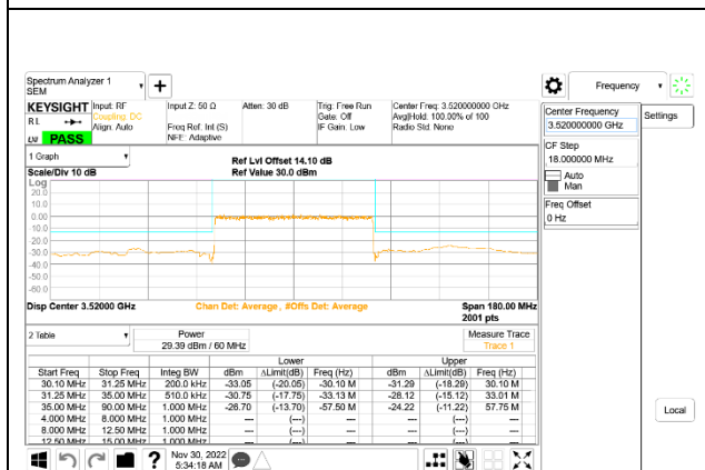
5G NR n77 60MHz BPSK High Channel RB162-0: ID 52275
