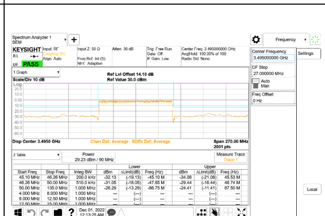
5G NR n77 90MHz BPSK Low Channel RB243-0: ID 52275
