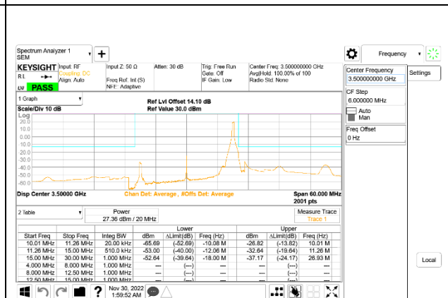
5G NR n77 20MHz BPSK Middle Channel RB1-50: ID 52275
