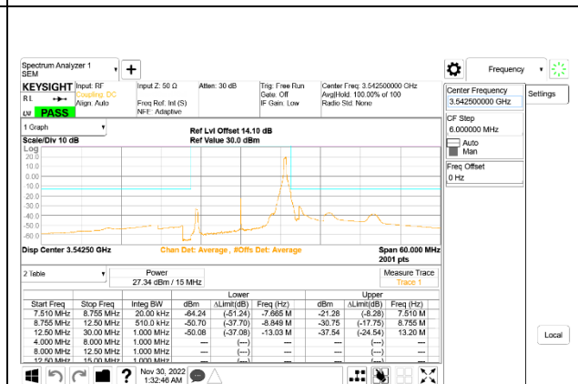
5G NR n77 15MHz BPSK High Channel RB1-37: ID 52275
