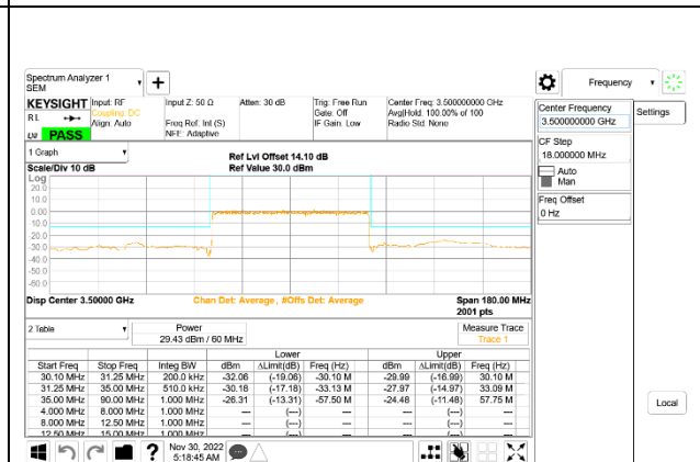
5G NR n77 60MHz BPSK Middle Channel RB162-0: ID 52275
