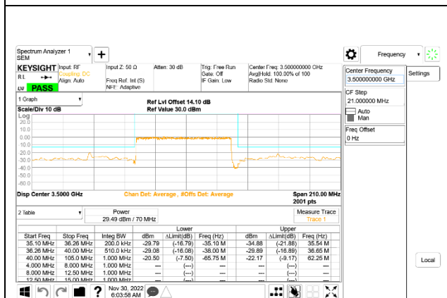
5G NR n77 70MHz BPSK Middle Channel RB180-0: ID 52275
