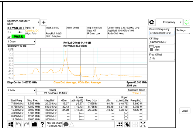
5G NR n77 15MHz BPSK Low Channel RB1-0: ID 52275
