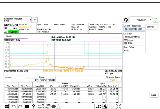
5G NR n77 70MHz BPSK High Channel RB1-0: ID 52275
