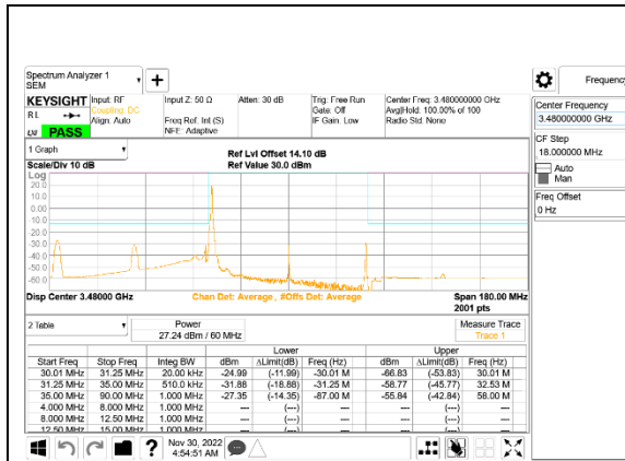
5G NR n77 60MHz BPSK Low Channel RB1-0: ID 52275
