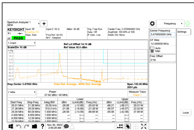
5G NR n77 40MHz BPSK Low Channel RB1-0: ID 52275
