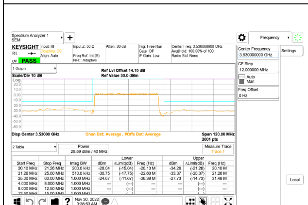
5G NR n77 40MHz BPSK High Channel RB100-0: ID 52275
