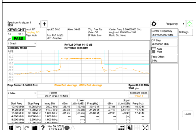
5G NR n77 20MHz BPSK High Channel RB50-0: ID 52275
