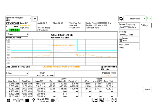
5G NR n77 15MHz BPSK Low Channel RB36-0: ID 52275
