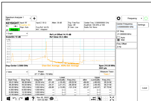
5G NR n77 70MHz BPSK Middle Channel RB1-0: ID 52275
