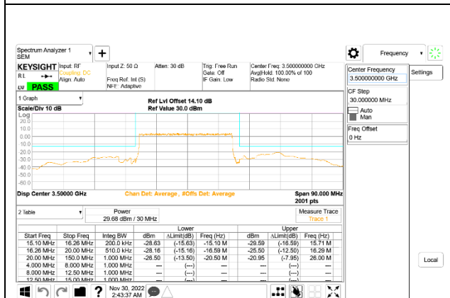
5G NR n77 30MHz BPSK Middle Channel RB75-0: ID 52275
