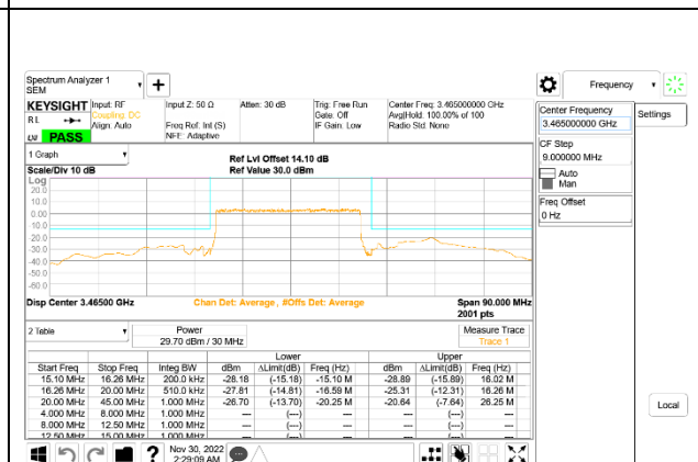
5G NR n77 30MHz BPSK Low Channel RB75-0: ID 52275
