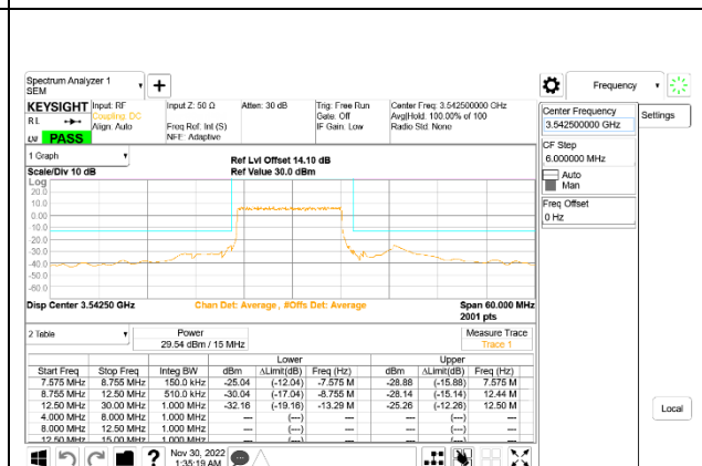
5G NR n77 15MHz BPSK High Channel RB36-0: ID 52275
