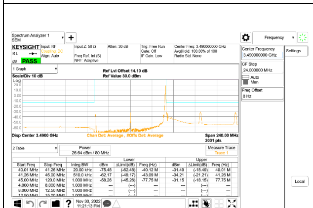
5G NR n77 80MHz BPSK Low Channel RB1-216: ID 52275
