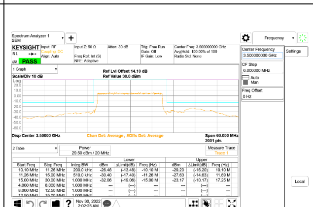
5G NR n77 20MHz BPSK Middle Channel RB50-0: ID 52275
