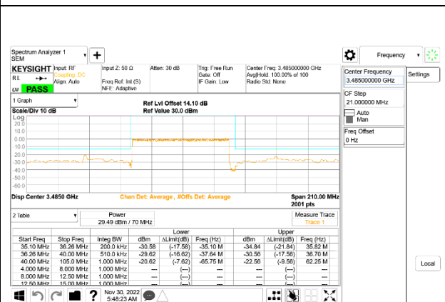
5G NR n77 70MHz BPSK Low Channel RB180-0: ID 52275
