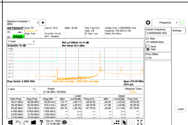
5G NR n77 90MHz BPSK Low Channel RB1-244: ID 52275
