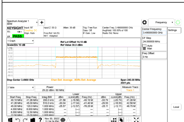
5G NR n77 80MHz BPSK Low Channel RB216-0: ID 52275
