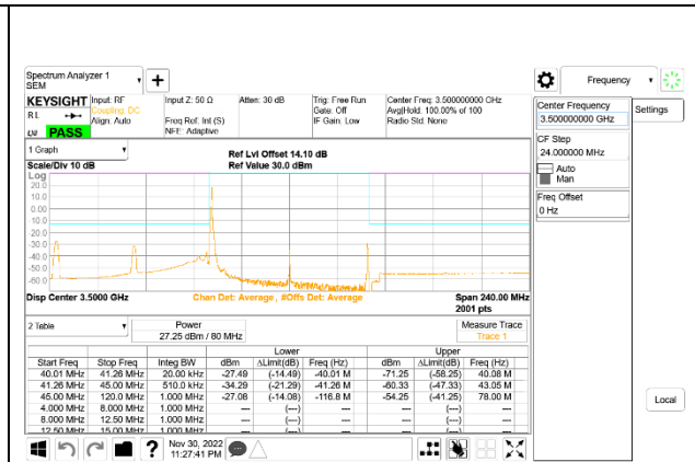
5G NR n77 80MHz BPSK Middle Channel RB1-0: ID 52275
