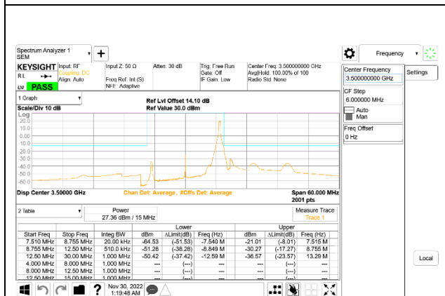
5G NR n77 15MHz BPSK Middle Channel RB1-37: ID 52275
