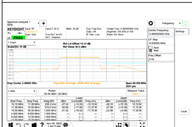
5G NR n77 20MHz BPSK Low Channel RB50-0: ID 52275
