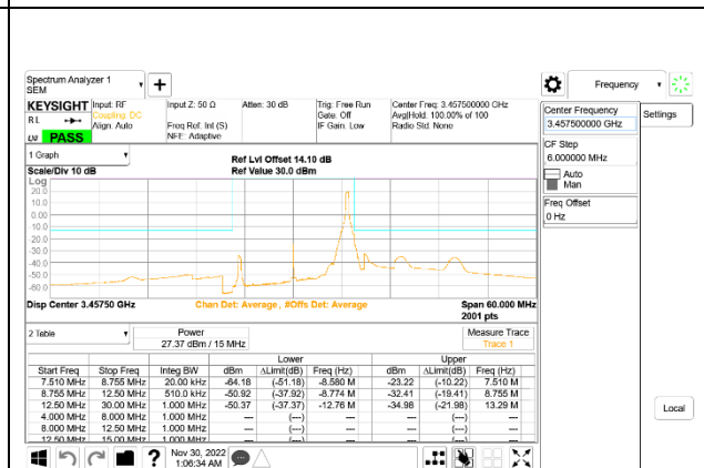
5G NR n77 15MHz BPSK Low Channel RB1-37: ID 52275
