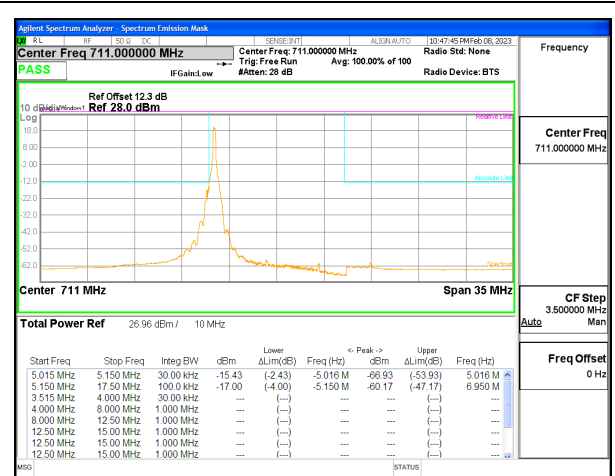
5G NR n12 10MHz BPSK High Channel RB1-0, ID:12482
