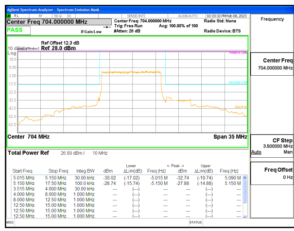
5G NR n12 10MHz BPSK Low Channel RB50-0, ID:12482
