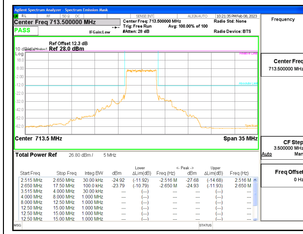
5G NR n12 5MHz BPSK High Channel RB25-0, ID:12482
