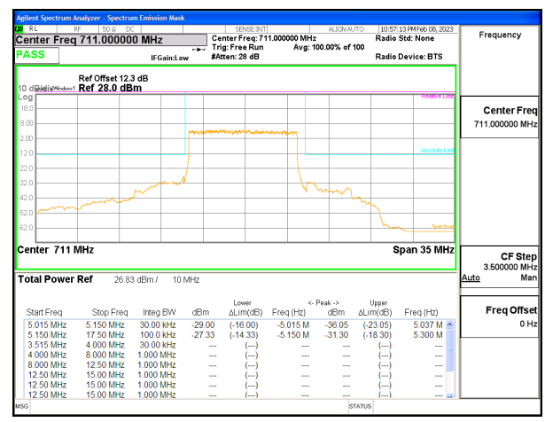
5G NR n12 10MHz BPSK High Channel RB50-0, ID:12482
