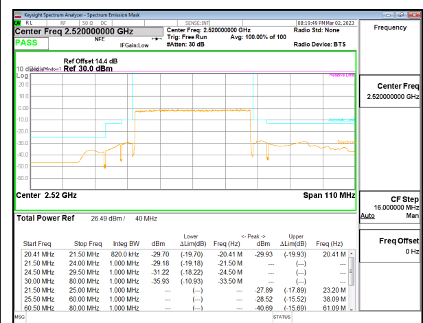
5G NR n7 40MHz BPSK Low Channel RB216-0, ID:32061
