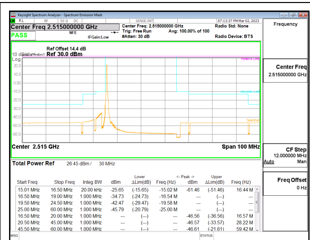
5G NR n7 30MHz BPSK Low Channel RB1-0, ID:32061
