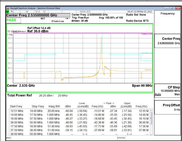
5G NR n7 25MHz BPSK Middle Channel RB1-132, ID:32061
