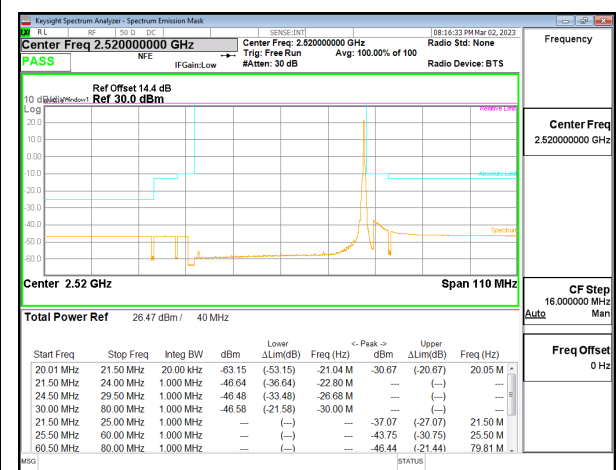
5G NR n7 40MHz BPSK Low Channel RB1-215, ID:32061
