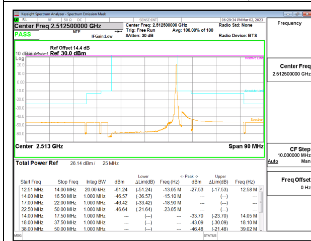
5G NR n7 25MHz BPSK Low Channel RB1-132, ID:32061
