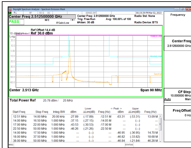
5G NR n7 25MHz BPSK Low Channel RB1-0, ID:32061
