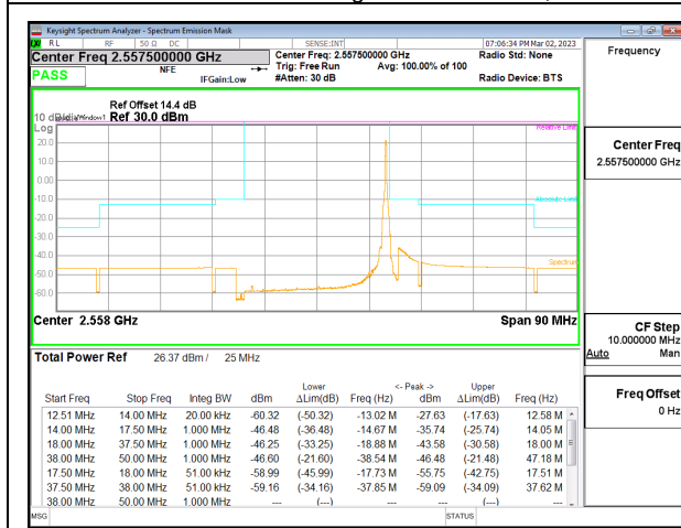
5G NR n7 25MHz BPSK High Channel RB1-132, ID:32061
