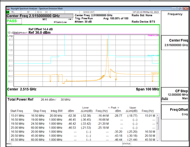
5G NR n7 30MHz BPSK Low Channel RB1-159, ID:32061
