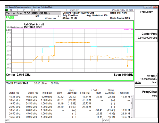
5G NR n7 30MHz BPSK Low Channel RB160-0, ID:32061
