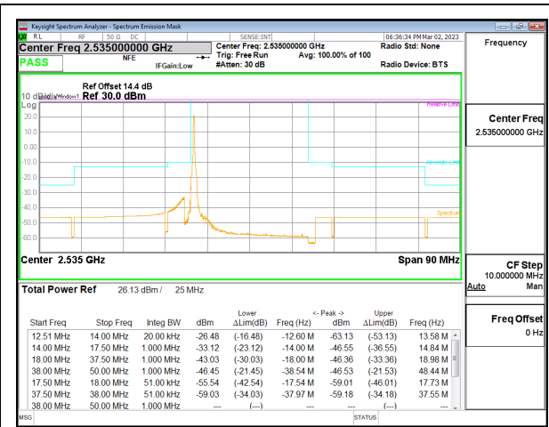
5G NR n7 25MHz BPSK Middle Channel RB1-0, ID:32061
