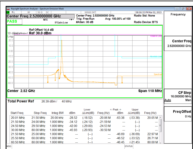
5G NR n7 40MHz BPSK Low Channel RB1-0, ID:32061
