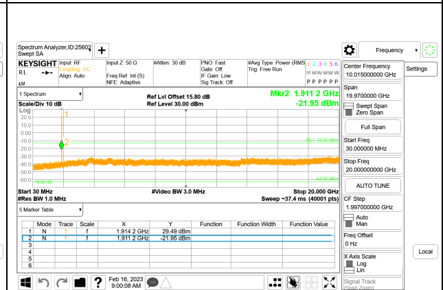
5G NR n25 30MHz BPSK High Channel RB1-159
