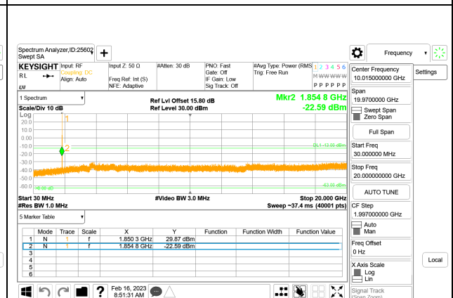
5G NR n25 20MHz BPSK Low Channel RB1-0
