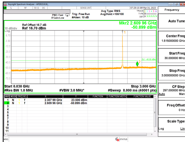
5G NR n30 5MHz QPSK Mid Channel RB1-0 (30MHz to 3GHz) ID:32061
