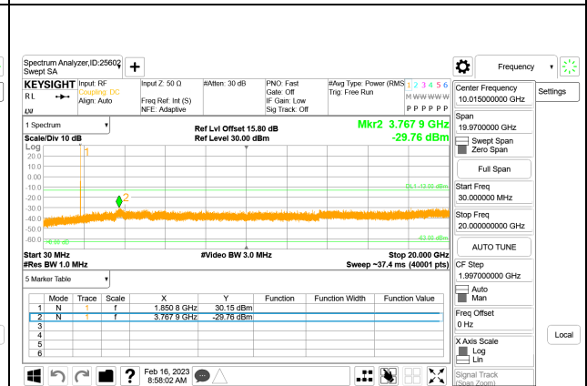
5G NR n25 30MHz BPSK Low Channel RB1-0
