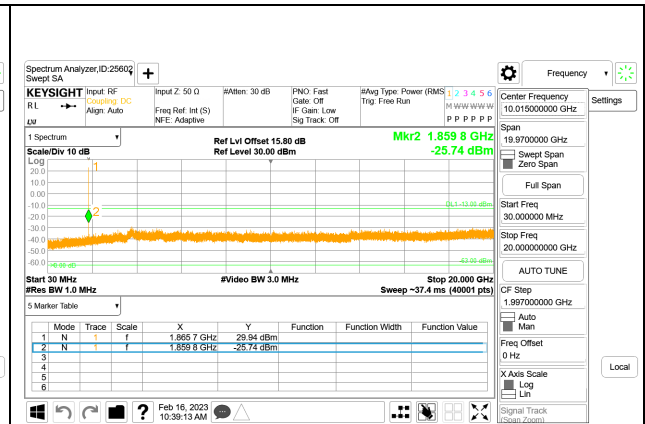
5G NR n25 35MHz BPSK Low Channel RB1-1
