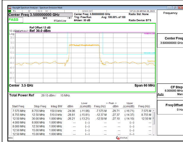
5G NR n77 15MHz BPSK Middle Channel RB36-0, ID:19146
