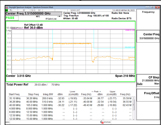
5G NR n77 70MHz BPSK High Channel RB180-0, ID:19146
