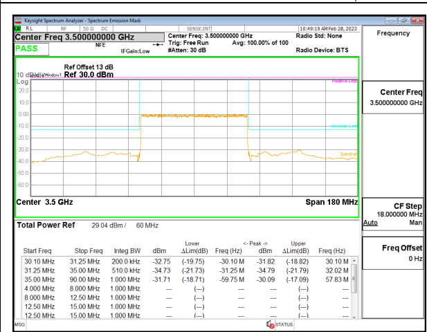
5G NR n77 60MHz BPSK Middle Channel RB162-0, ID:19146
