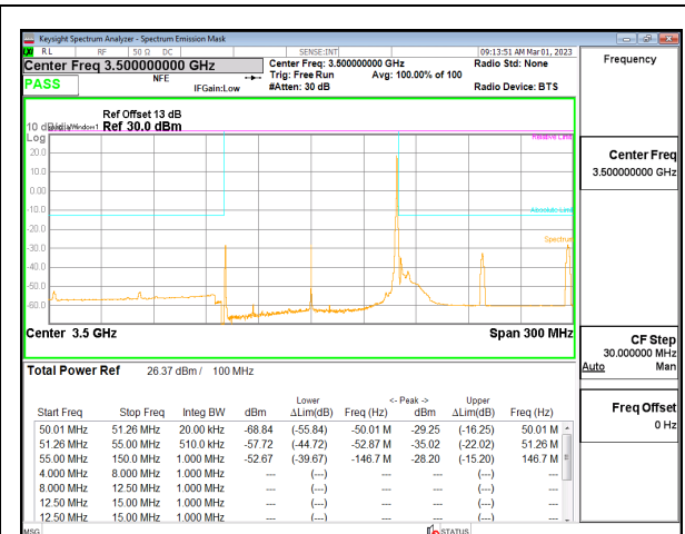
5G NR n77 100MHz BPSK Middle Channel RB1-272, ID:19146
