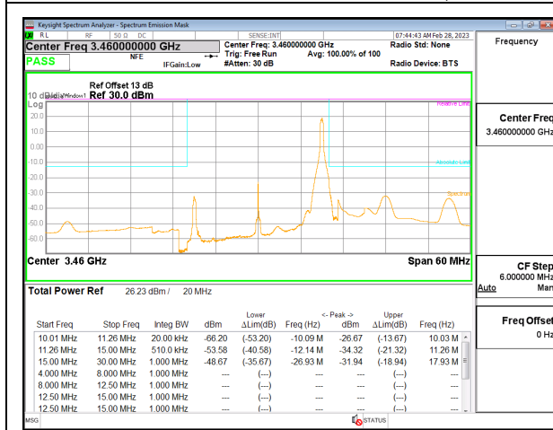
5G NR n77 20MHz BPSK Low Channel RB1-50, ID:19146
