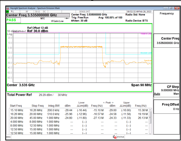
5G NR n77 30MHz BPSK High Channel RB75-0, ID:19146
