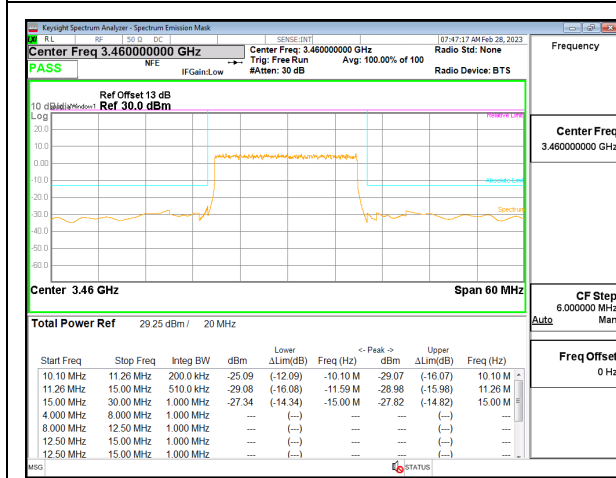
5G NR n77 20MHz BPSK Low Channel RB50-0, ID:19146
