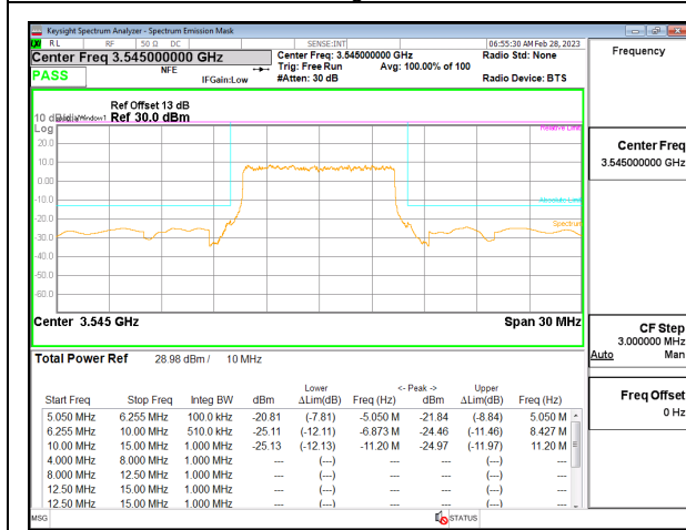
5G NR n77 10MHz BPSK High Channel RB24-0, ID:19146
