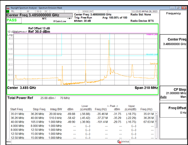
5G NR n77 70MHz BPSK Low Channel RB1-188, ID:19146
