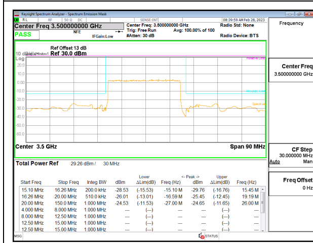
5G NR n77 30MHz BPSK Middle Channel RB75-0, ID:19146
