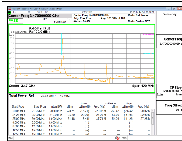
5G NR n77 40MHz BPSK Low Channel RB1-0, ID:19146
