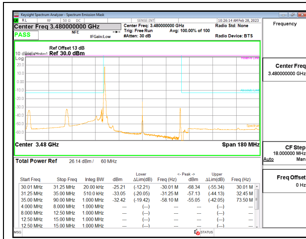
5G NR n77 60MHz BPSK Low Channel RB1-0, ID:19146
