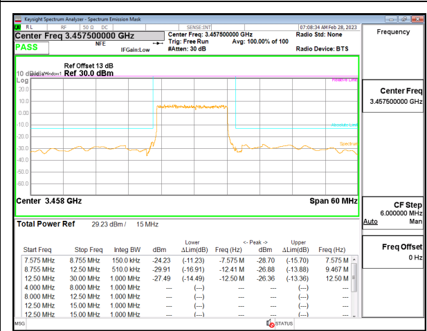
5G NR n77 15MHz BPSK Low Channel RB36-0, ID:19146
