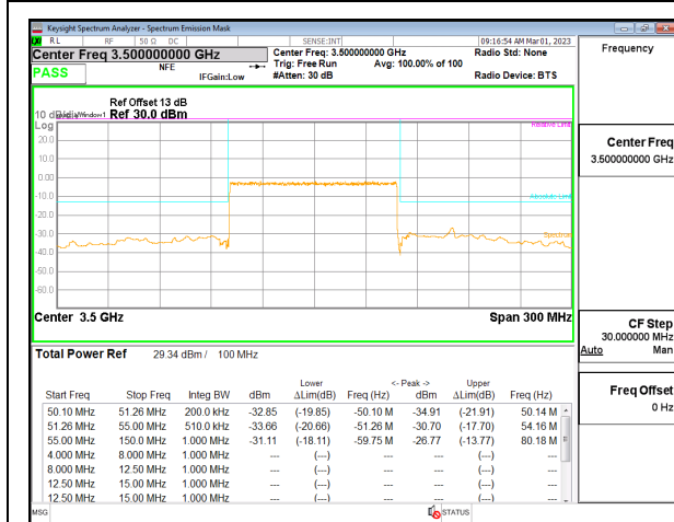
5G NR n77 100MHz BPSK Middle Channel RB270-0, ID:19146
