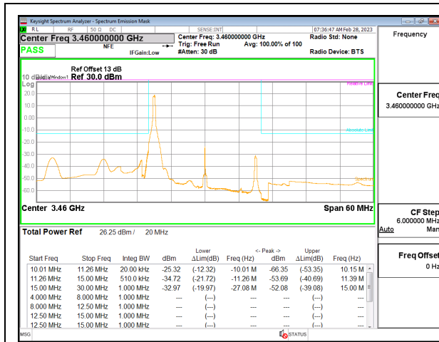
5G NR n77 20MHz BPSK Low Channel RB1-0, ID:19146
