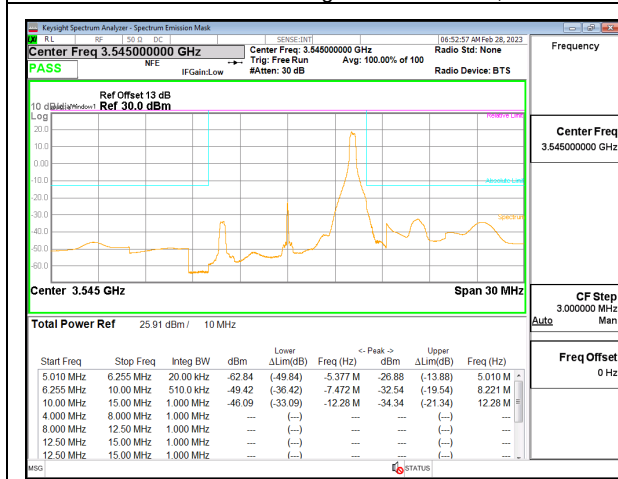
5G NR n77 10MHz BPSK High Channel RB1-23, ID:19146
