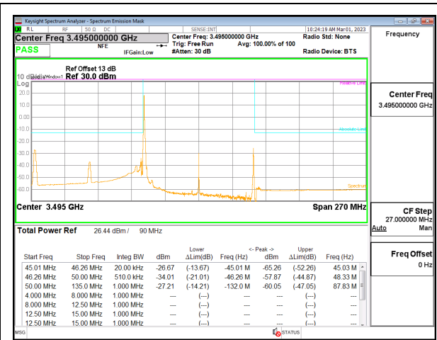
5G NR n77 90MHz BPSK Low Channel RB1-0, ID:19146
