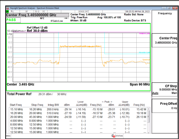
5G NR n77 30MHz BPSK Low Channel RB75-0, ID:19146
