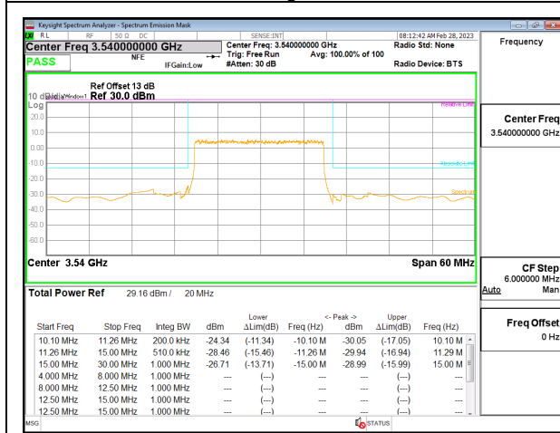
5G NR n77 20MHz BPSK High Channel RB50-0, ID:19146
