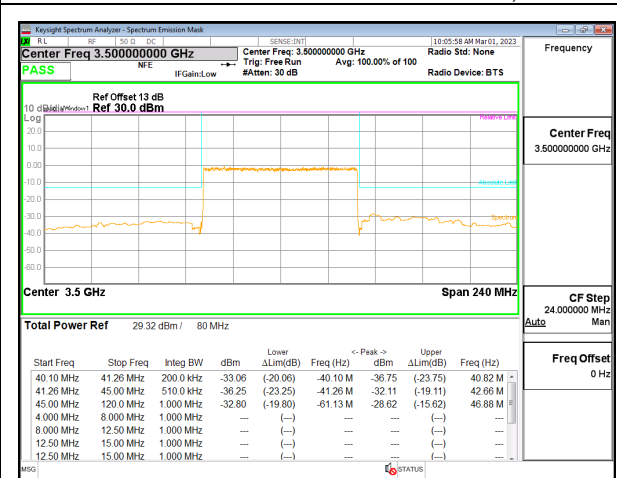
5G NR n77 80MHz BPSK Middle Channel RB216-0, ID:19146
