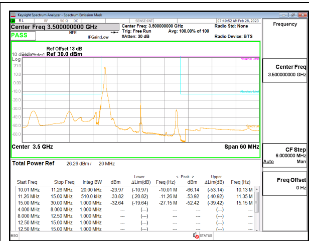
5G NR n77 20MHz BPSK Middle Channel RB1-0, ID:19146
