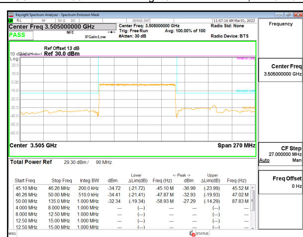
5G NR n77 90MHz BPSK High Channel RB243-0, ID:19146
