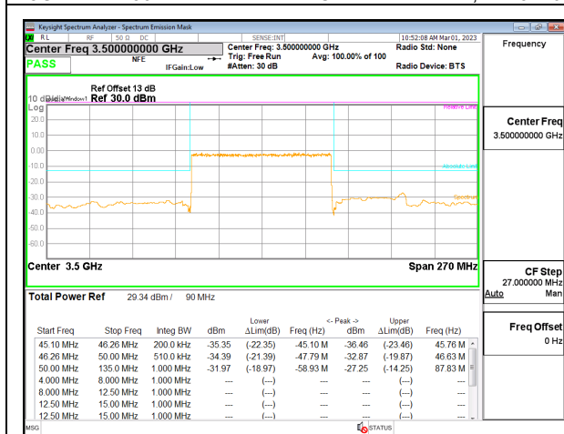
5G NR n77 90MHz BPSK Middle Channel RB243-0, ID:19146
