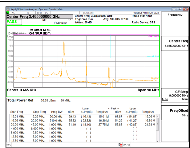
5G NR n77 30MHz BPSK Low Channel RB1-0, ID:19146
