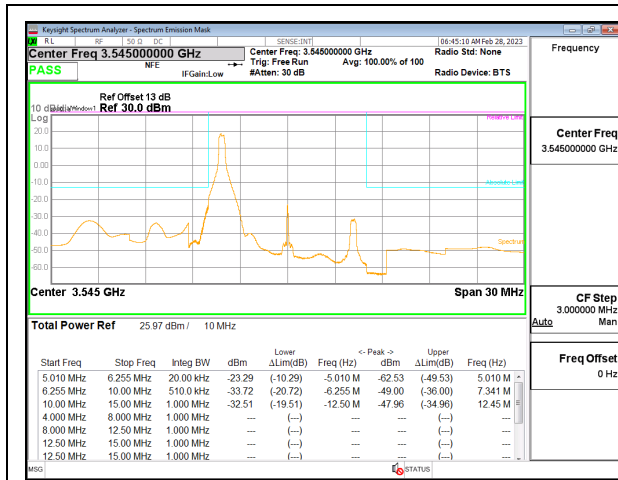
5G NR n77 10MHz BPSK High Channel RB1-0, ID:19146
