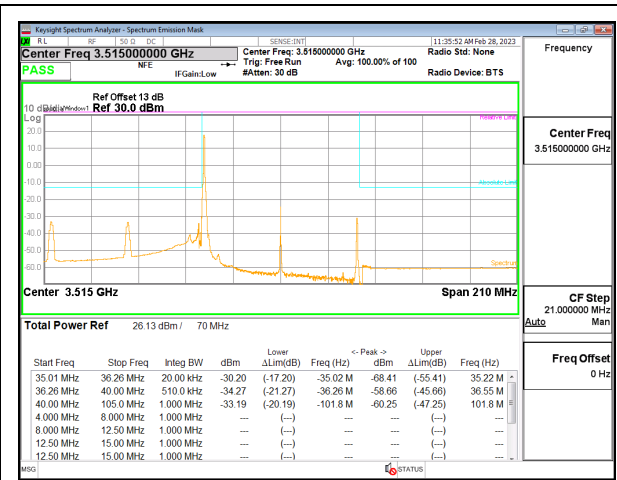
5G NR n77 70MHz BPSK High Channel RB1-0, ID:19146
