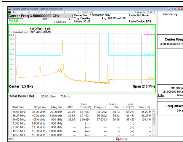
5G NR n77 70MHz BPSK Middle Channel RB1-0, ID:19146
