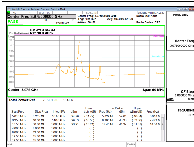
5G NR n77 10MHz BPSK High Channel RB1-0, ID:50822
