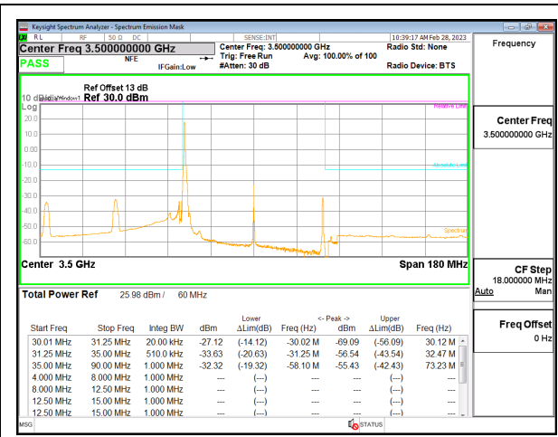
5G NR n77 60MHz BPSK Middle Channel RB1-0, ID:19146
