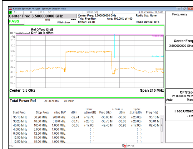
5G NR n77 70MHz BPSK Middle Channel RB180-0, ID:19146
