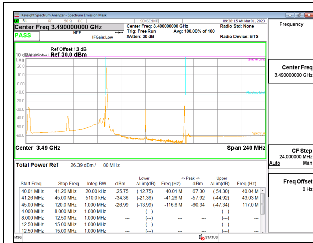
5G NR n77 80MHz BPSK Low Channel RB1-0, ID:19146
