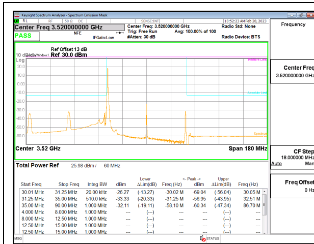
5G NR n77 60MHz BPSK High Channel RB1-0, ID:19146
