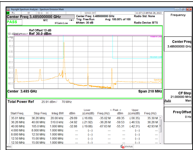
5G NR n77 70MHz BPSK Low Channel RB1-0, ID:19146
