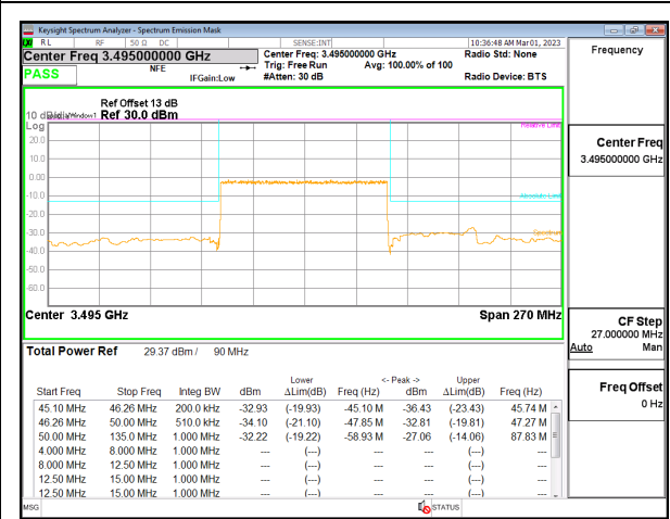
5G NR n77 90MHz BPSK Low Channel RB243-0, ID:19146
