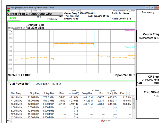
5G NR n77 80MHz BPSK Low Channel RB216-0, ID:19146
