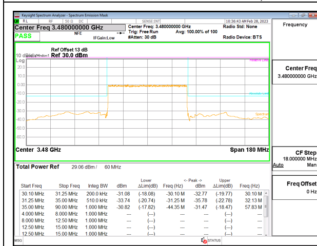
5G NR n77 60MHz BPSK Low Channel RB162-0, ID:19146
