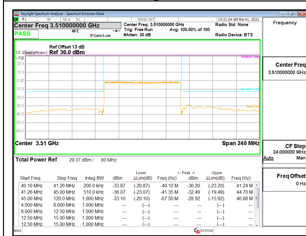
5G NR n77 80MHz BPSK High Channel RB216-0, ID:19146
