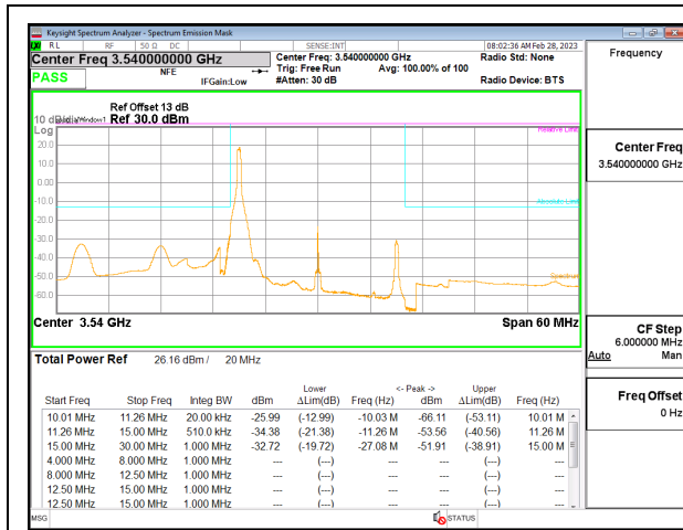
5G NR n77 20MHz BPSK High Channel RB1-0, ID:19146
