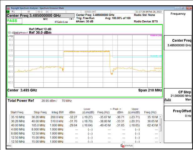
5G NR n77 70MHz BPSK Low Channel RB180-0, ID:19146
