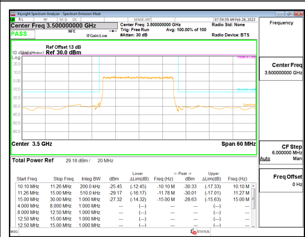
5G NR n77 20MHz BPSK Middle Channel RB50-0, ID:19146
