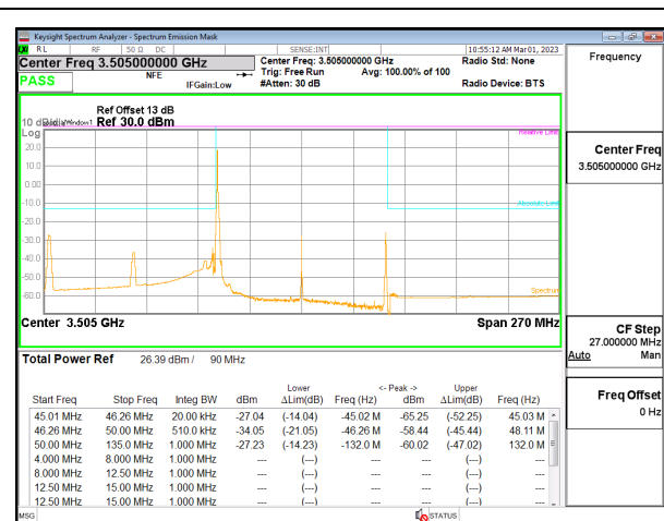
5G NR n77 90MHz BPSK High Channel RB1-0, ID:19146
