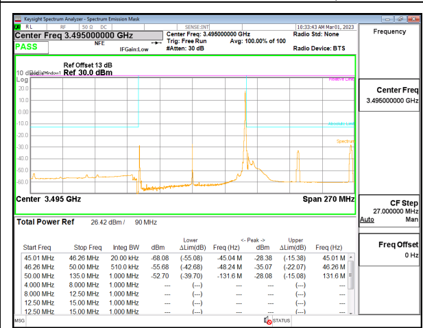
5G NR n77 90MHz BPSK Low Channel RB1-244, ID:19146
