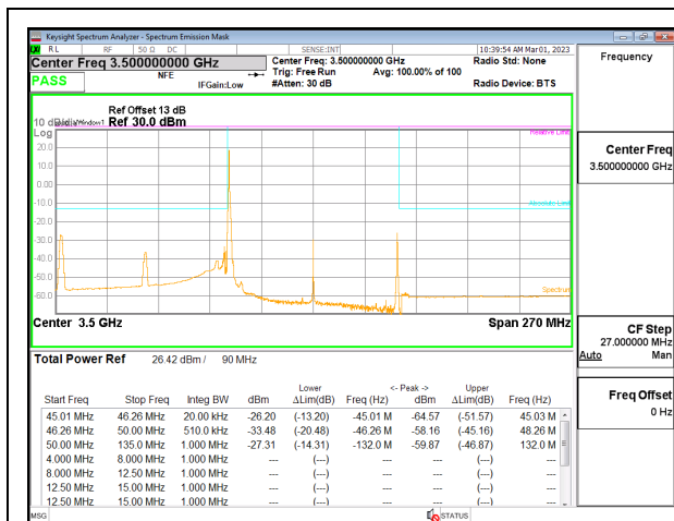
5G NR n77 90MHz BPSK Middle Channel RB1-0, ID:19146
