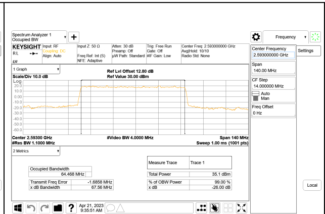
5G NR n41 70MHz BPSK Middle Channel RB180-0.ID:32061
