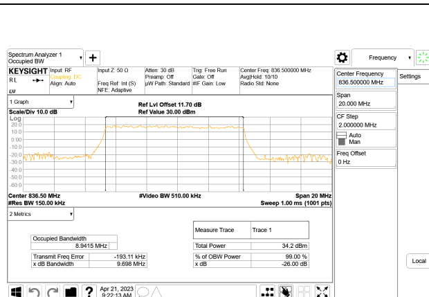
5G NR n26 10MHz BPSK Middle Channel RB50-0,ID:32061
