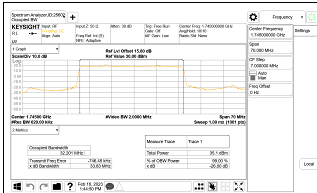
5G NR n66 35MHz BPSK Middle Channel RB180-0
