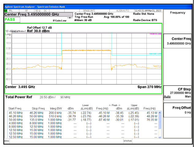
5G NR n77 90MHz BPSK Low Channel RB243-0, ID:28568
