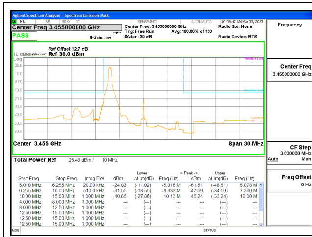
5G NR n77 10MHz BPSK Low Channel RB1-0, ID:28568
