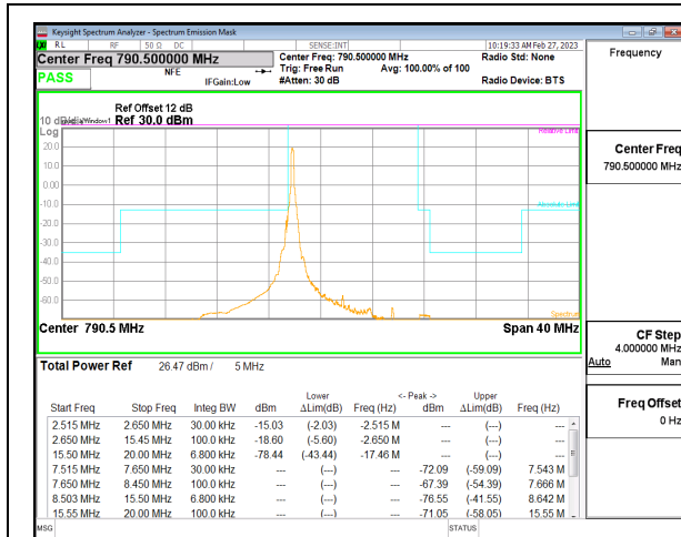
5G NR n14 5MHz BPSK Low Channel RB1-0, ID:28568
