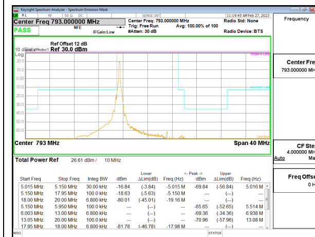
5G NR n14 10MHz BPSK Middle Channel RB1-0, ID:28568
