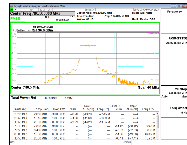
5G NR n14 5MHz BPSK Low Channel RB25-0, ID:28568
