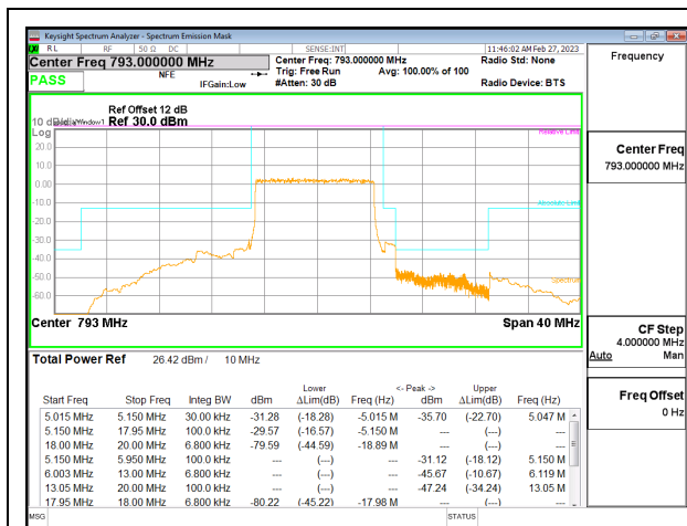
5G NR n14 10MHz BPSK Middle Channel RB50-0, ID:28568
