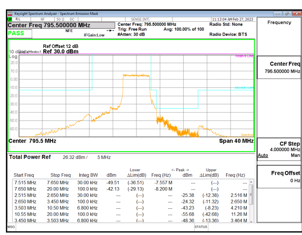
5G NR n14 5MHz BPSK High Channel RB25-0, ID:28568
