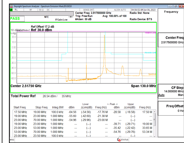
5G NR n7 35MHz BPSK Low Channel RB1-187
