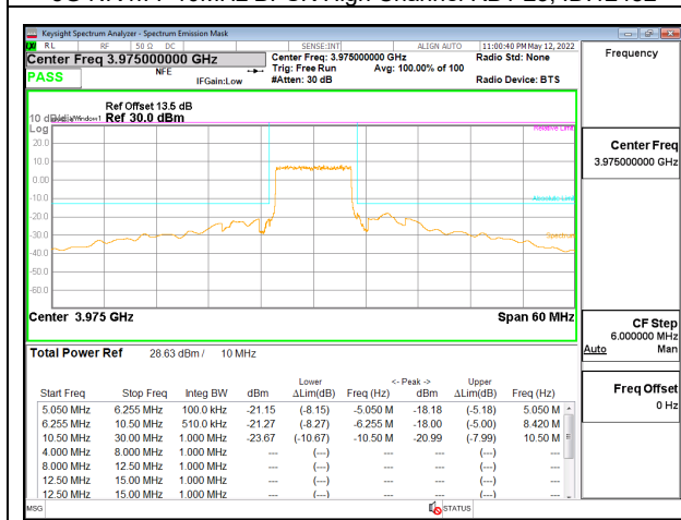
5G NR n77 10MHz BPSK High Channel RB24-0, ID:12482
