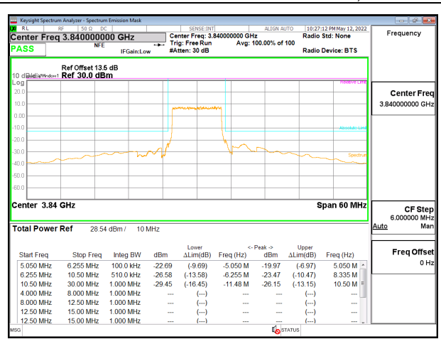
5G NR n77 10MHz BPSK Middle Channel RB24-0, ID:12482
