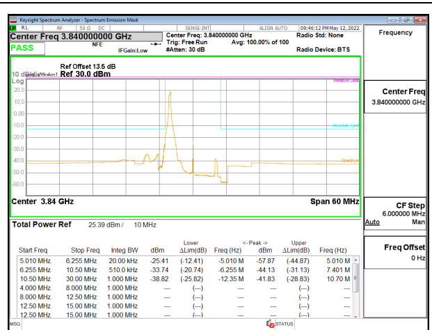
5G NR n77 10MHz BPSK Middle Channel RB1-0, ID:12482
