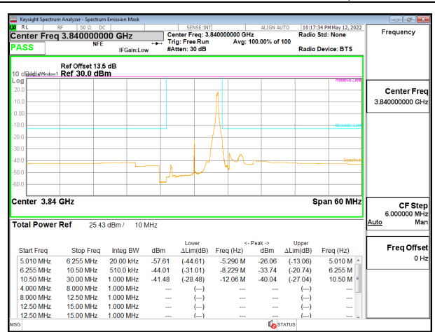
5G NR n77 10MHz BPSK Middle Channel RB1-23, ID:12482
