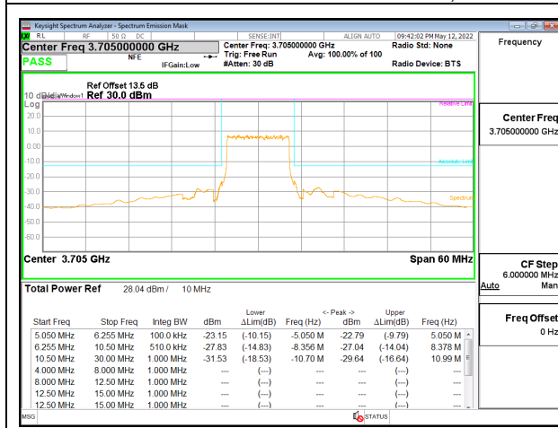
5G NR n77 10MHz BPSK Low Channel RB24-0, ID:12482
