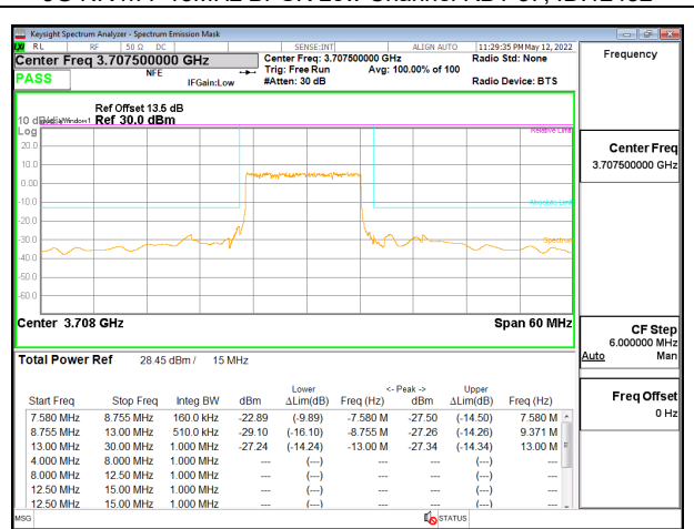
5G NR n77 15MHz BPSK Low Channel RB36-0, ID:12482
