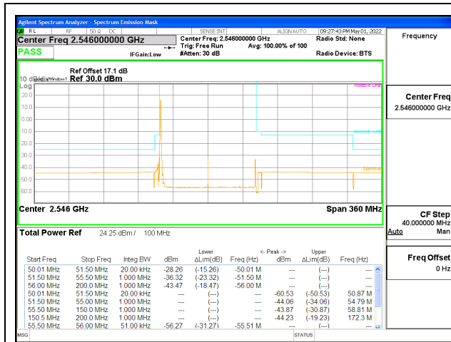
5G NR n41 100MHz BPSK Low Channel RB1-0, ID:25780
