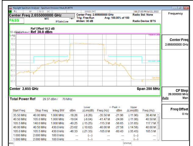
5G NR n41 60MHz BPSK High Channel RB162-0, ID:28774
