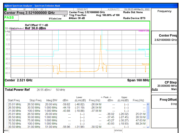
5G NR n41 50MHz BPSK Low Channel RB1-132, ID:25780
