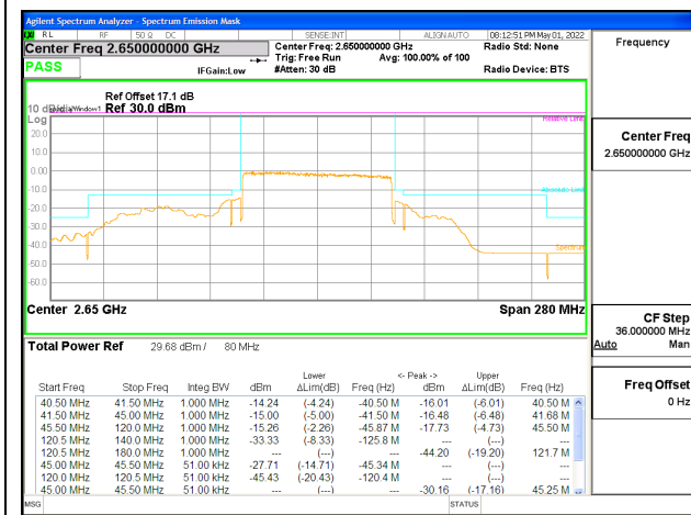
5G NR n41 80MHz BPSK High Channel RB216-0, ID:25780
