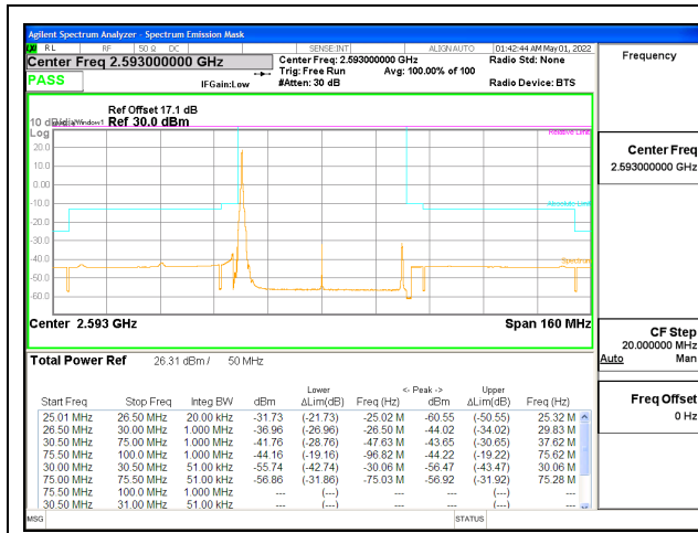
5G NR n41 50MHz BPSK Middle Channel RB1-0, ID:25780
