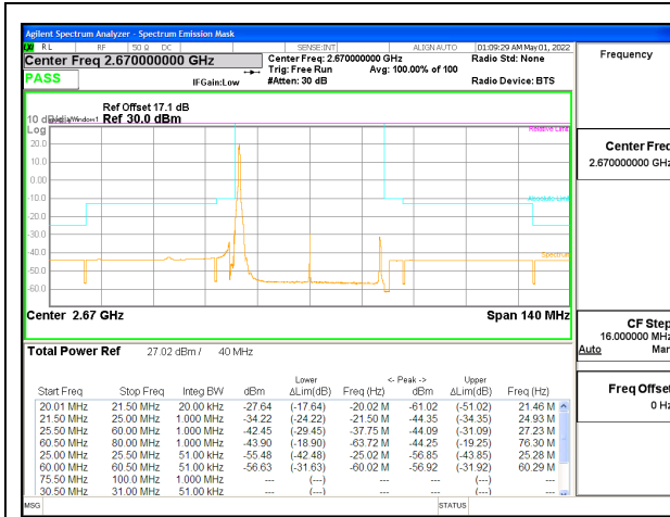
5G NR n41 40MHz BPSK High Channel RB1-0, ID:25780
