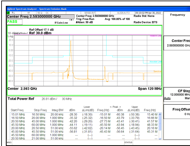
5G NR n41 30MHz BPSK Middle Channel RB1-0, ID:25780
