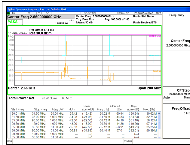
5G NR n41 60MHz BPSK High Channel RB1-0, ID:25780
