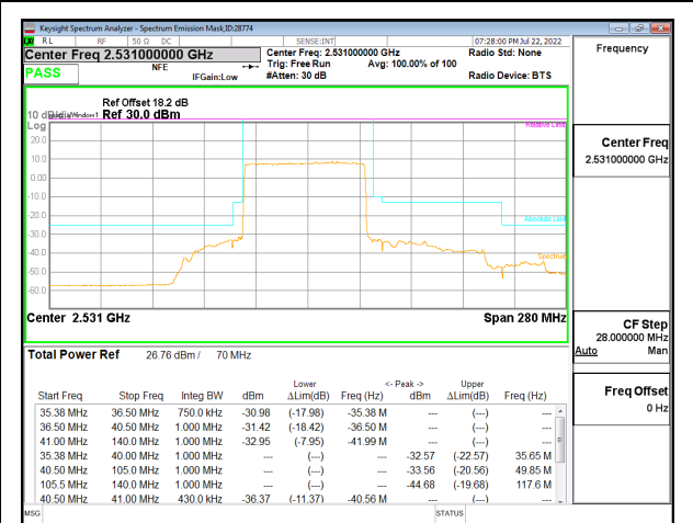
5G NR n41 70MHz BPSK Low Channel RB180-0, ID:28774
