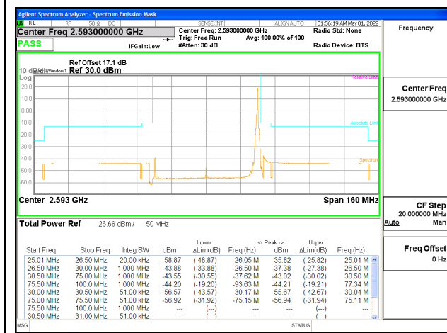
5G NR n41 50MHz BPSK Middle Channel RB1-132, ID:25780
