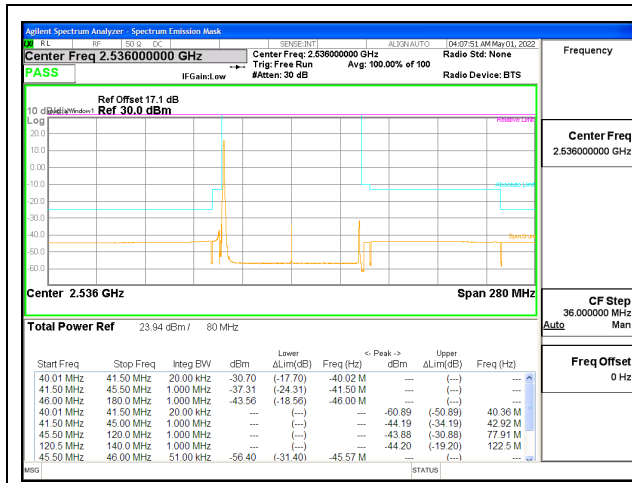
5G NR n41 80MHz BPSK Low Channel RB1-0, ID:25780
