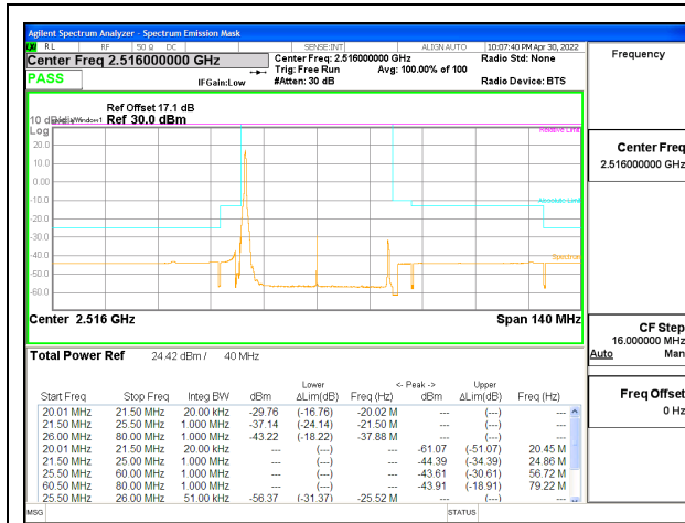
5G NR n41 40MHz BPSK Low Channel RB1-0, ID:25780
