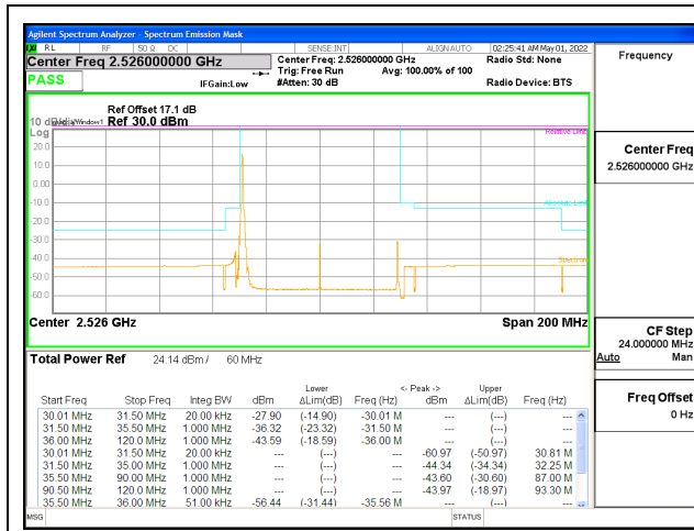
5G NR n41 60MHz BPSK Low Channel RB1-0, ID:25780
