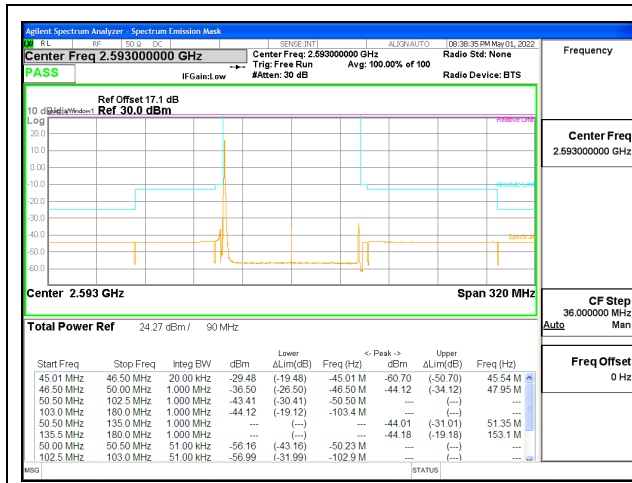
5G NR n41 90MHz BPSK Middle Channel RB1-0, ID:25780
