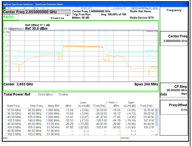
5G NR n41 70MHz BPSK High Channel RB180-0, ID:25780
