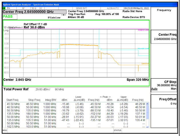
5G NR n41 90MHz BPSK High Channel RB243-0, ID:25780
