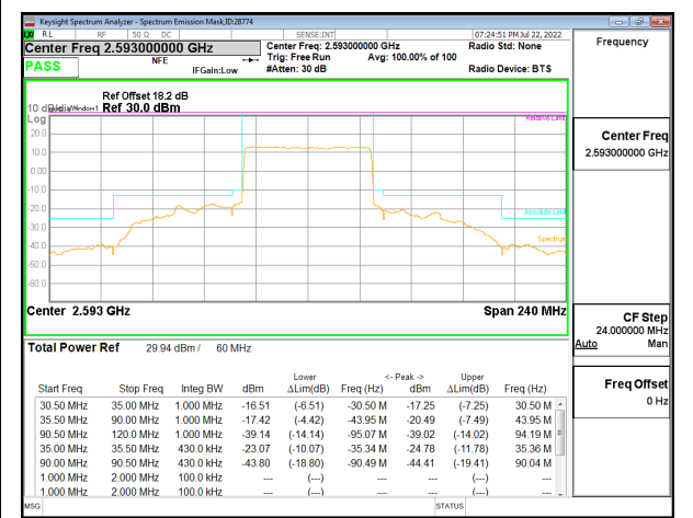
5G NR n41 60MHz BPSK Middle Channel RB162-0, ID:28774
