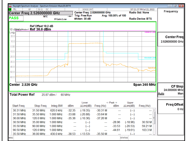
5G NR n41 60MHz BPSK Low Channel RB162-0, ID:28774
