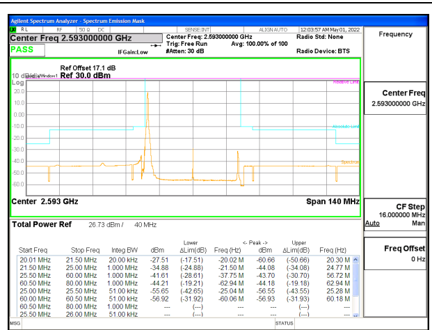
5G NR n41 40MHz BPSK Middle Channel RB1-0, ID:25780
