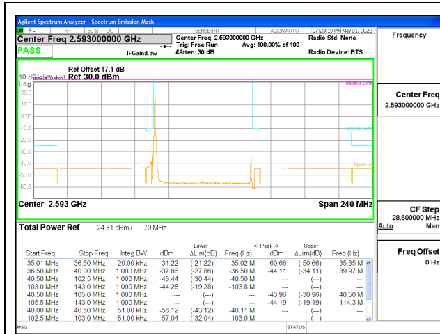
5G NR n41 70MHz BPSK Middle Channel RB1-0, ID:25780
