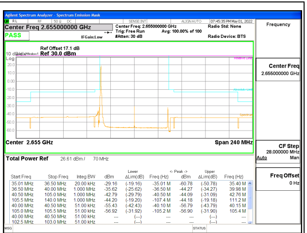
5G NR n41 70MHz BPSK High Channel RB1-0, ID:25780
