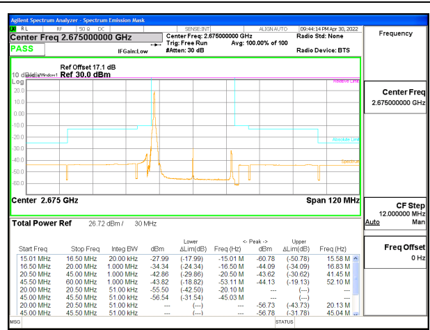
5G NR n41 30MHz BPSK High Channel RB1-0, ID:25780
