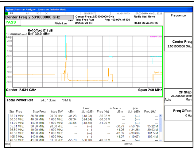
5G NR n41 70MHz BPSK Low Channel RB1-0, ID:25780
