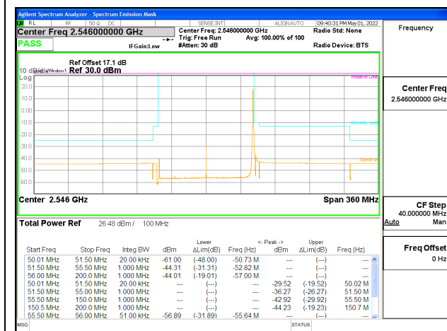
5G NR n41 100MHz BPSK Low Channel RB1-272, ID:25780
