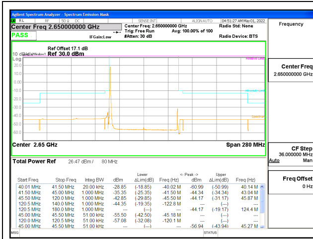
5G NR n41 80MHz BPSK High Channel RB1-0, ID:25780
