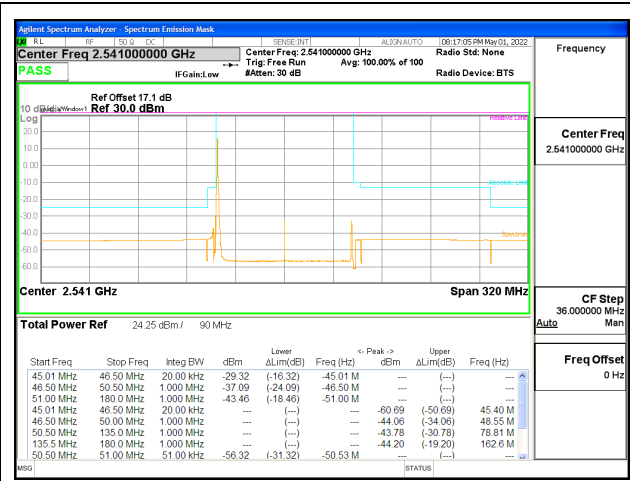
5G NR n41 90MHz BPSK Low Channel RB1-0, ID:25780
