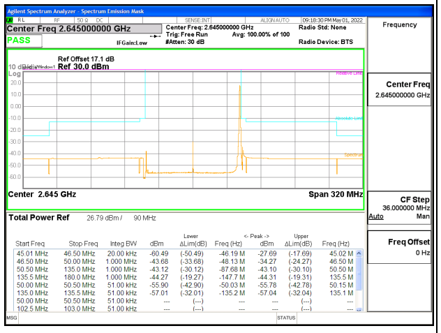
5G NR n41 90MHz BPSK High Channel RB1-244, ID:25780
