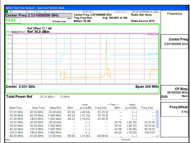
5G NR n41 70MHz BPSK Low Channel RB1-188, ID:25780
