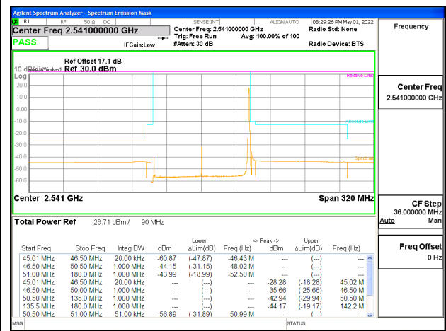
5G NR n41 90MHz BPSK Low Channel RB1-244, ID:25780
