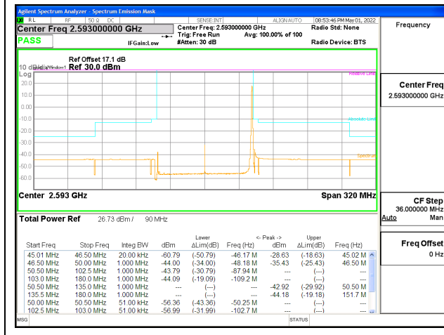
5G NR n41 90MHz BPSK Middle Channel RB1-244, ID:25780
