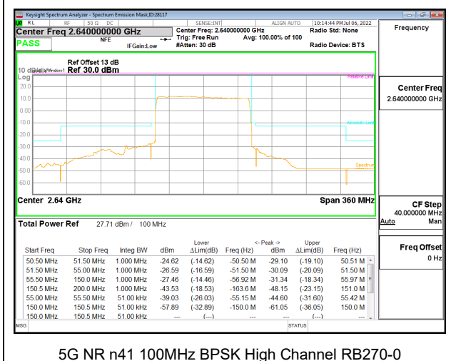
5G NR n41 100MHz BPSK High Channel RB270-0
