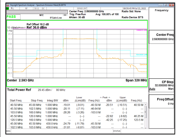
5G NR n41 80MHz BPSK Middle Channel RB216-0, ID:28774
