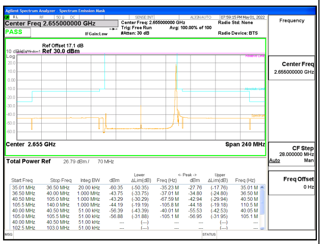
5G NR n41 70MHz BPSK High Channel RB1-188, ID:25780
