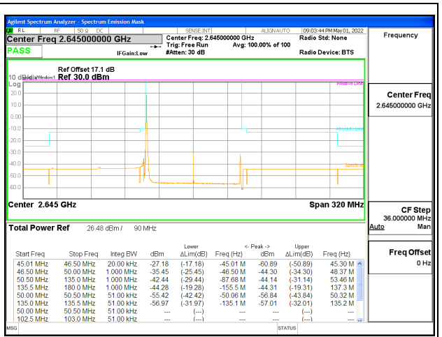
5G NR n41 90MHz BPSK High Channel RB1-0, ID:25780
