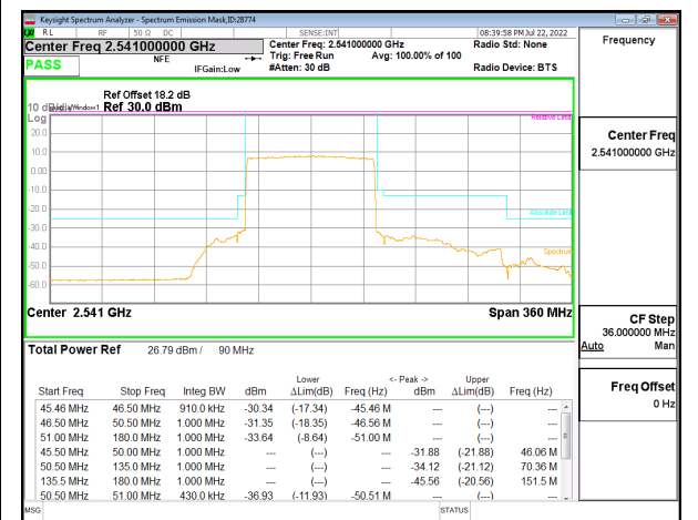
5G NR n41 90MHz BPSK Low Channel RB243-0, ID:28774
