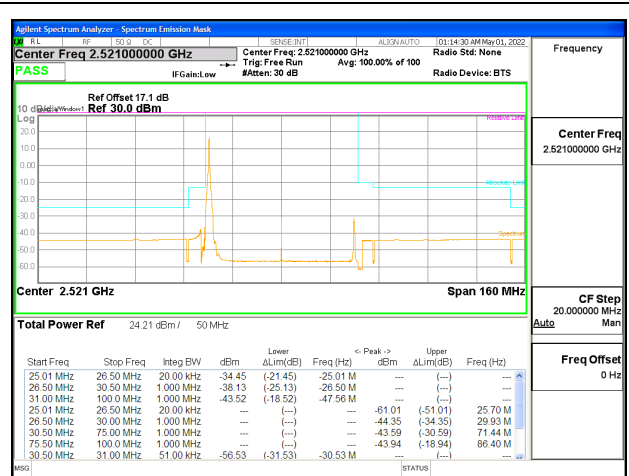
5G NR n41 50MHz BPSK Low Channel RB1-0, ID:25780
