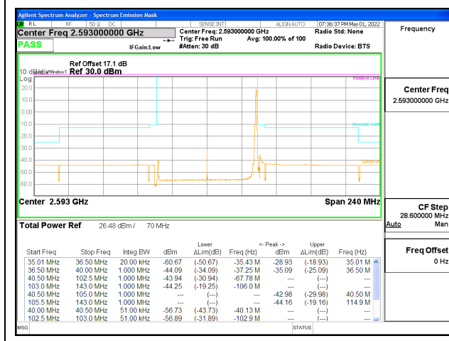
5G NR n41 70MHz BPSK Middle Channel RB1-188, ID:25780
