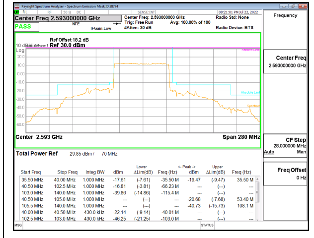
5G NR n41 70MHz BPSK Middle Channel RB180-0, ID:28774
