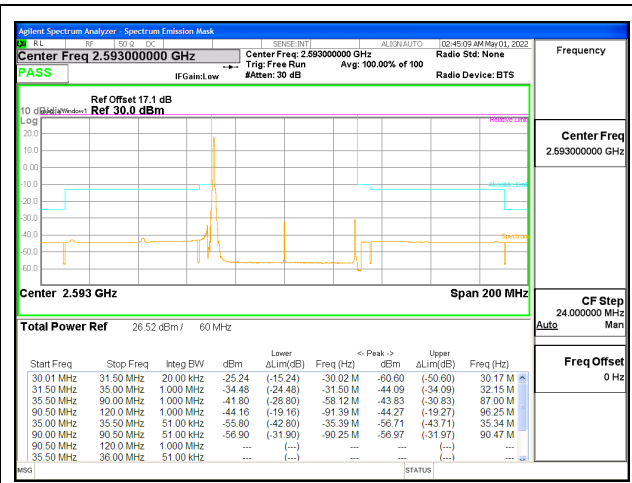
5G NR n41 60MHz BPSK Middle Channel RB1-0, ID:25780
