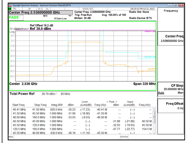
5G NR n41 80MHz BPSK Low Channel RB216-0, ID:28774
