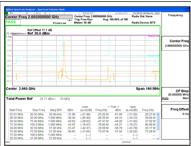
5G NR n41 50MHz BPSK High Channel RB1-0, ID:25780
