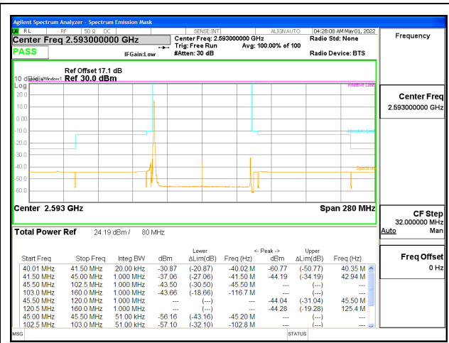
5G NR n41 80MHz BPSK Middle Channel RB1-0, ID:25780
