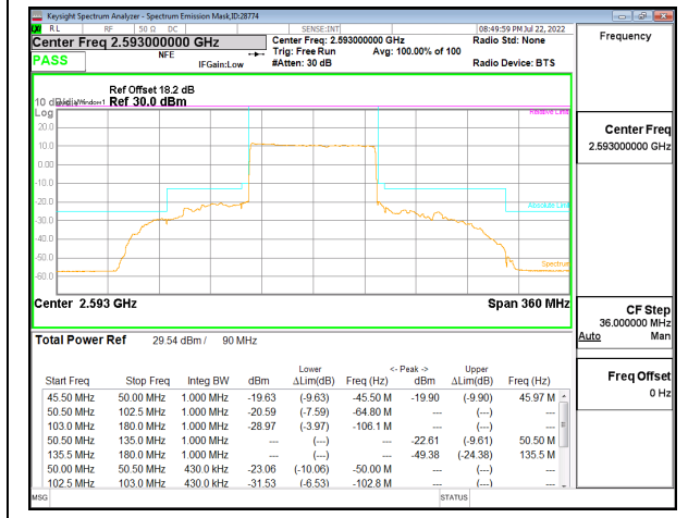
5G NR n41 90MHz BPSK Middle Channel RB243-0, ID:28774
