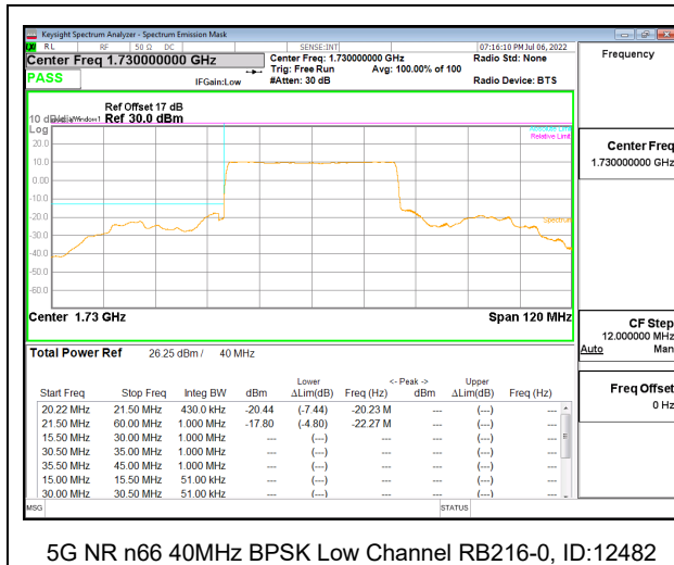
5G NR n66 40MHz BPSK Low Channel RB216-0, ID:12482
