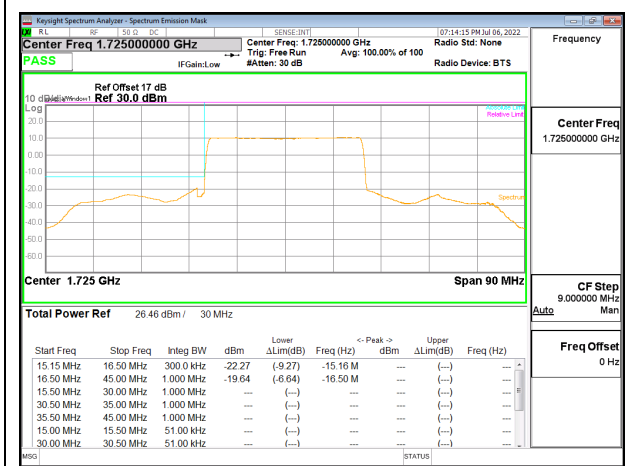
5G NR n66 30MHz BPSK Low Channel RB160-0, ID:12482
