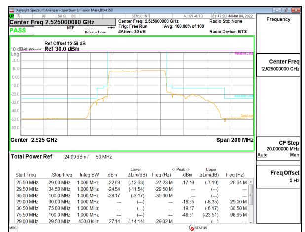
5G NR n7 50MHz BPSK Low Channel RB270-0
