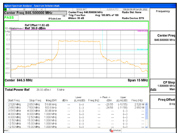
5G NR n5 5MHz BPSK High Channel RB25-0: ID 52275
