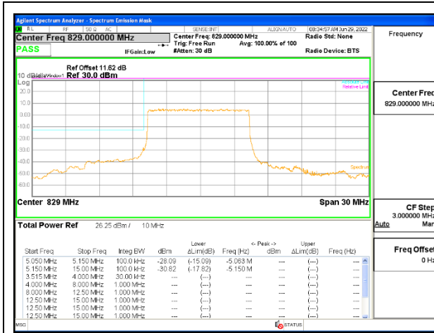
5G NR n5 10MHz BPSK Low Channel RB50-0: ID 52275
