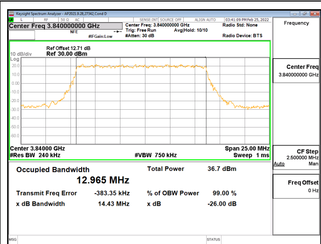
5G NR n77 15MHz BPSK Middle Channel RB24-0
