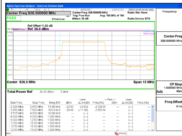
5G NR n5 5MHz BPSK Low Channel RB25-0: ID 52275
