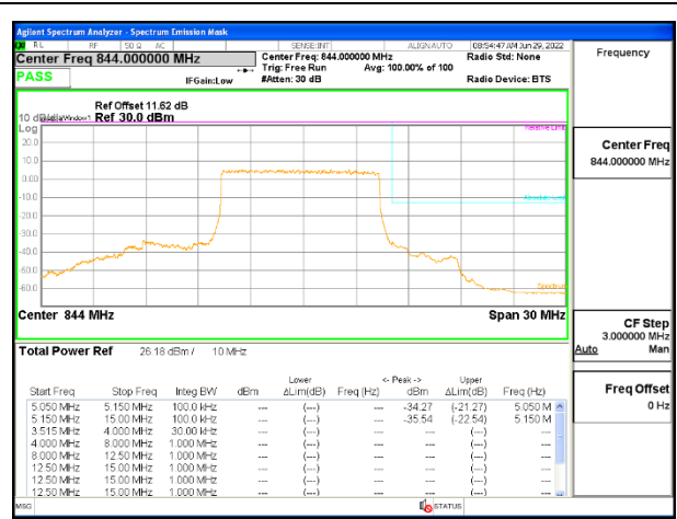
5G NR n5 10MHz BPSK High Channel RB50-0: ID 52275
