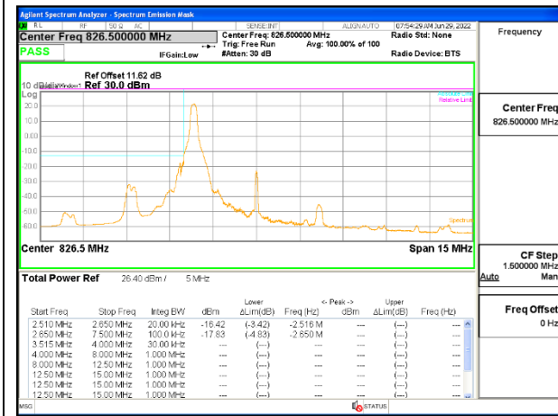
5G NR n5 5MHz BPSK Low Channel RB1-0: ID 52275
