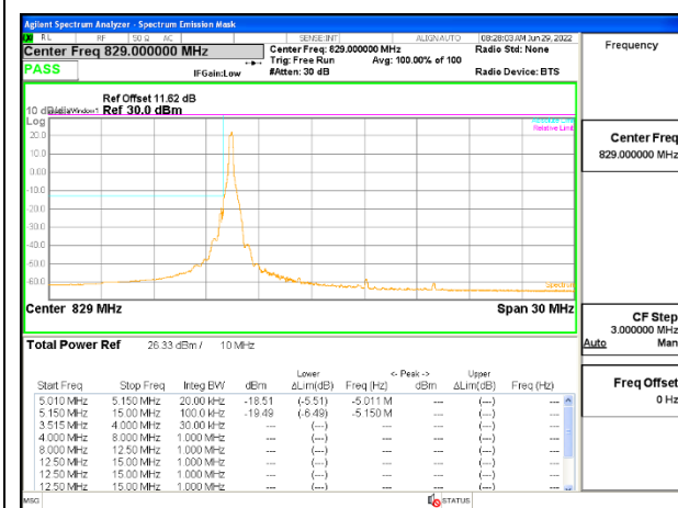
5G NR n5 10MHz BPSK Low Channel RB1-0: ID 52275
