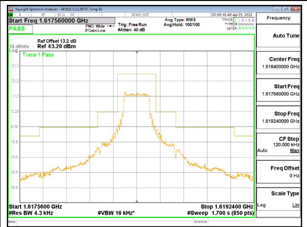
Mid 1618.40MHz
