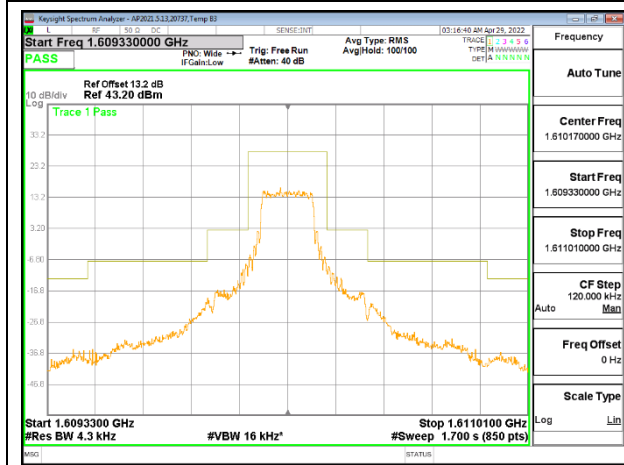
Low 1610.17MHz
