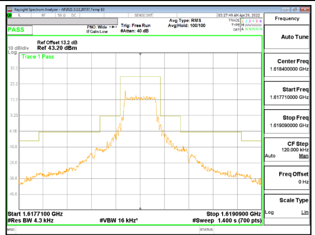
Mid 1618.40MHz
