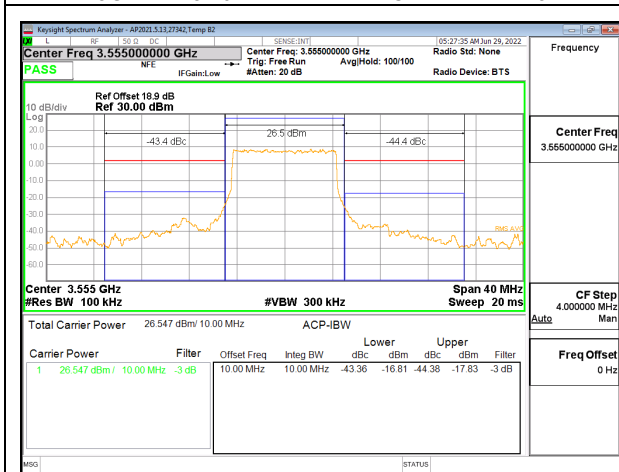
5G NR n48 10MHz BPSK Low Channel RB24-0
