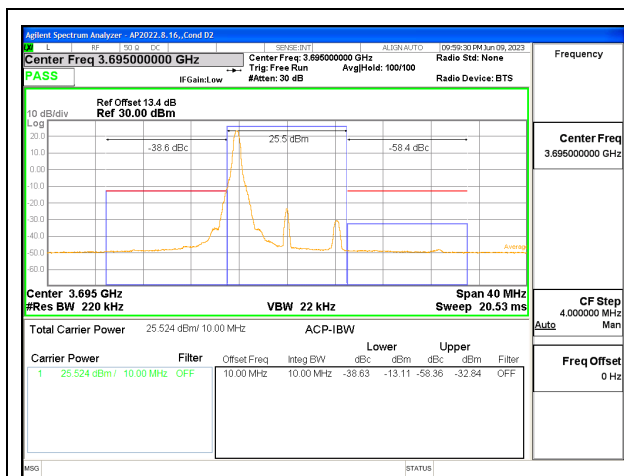
5G NR n48 10MHz BPSK High Channel RB1-0, ID:12482
