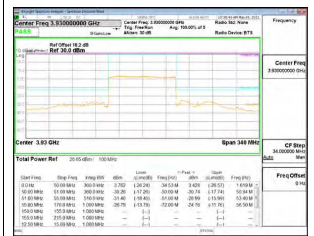
5G NR n77 100MHz BPSK High Channel RB270-0
